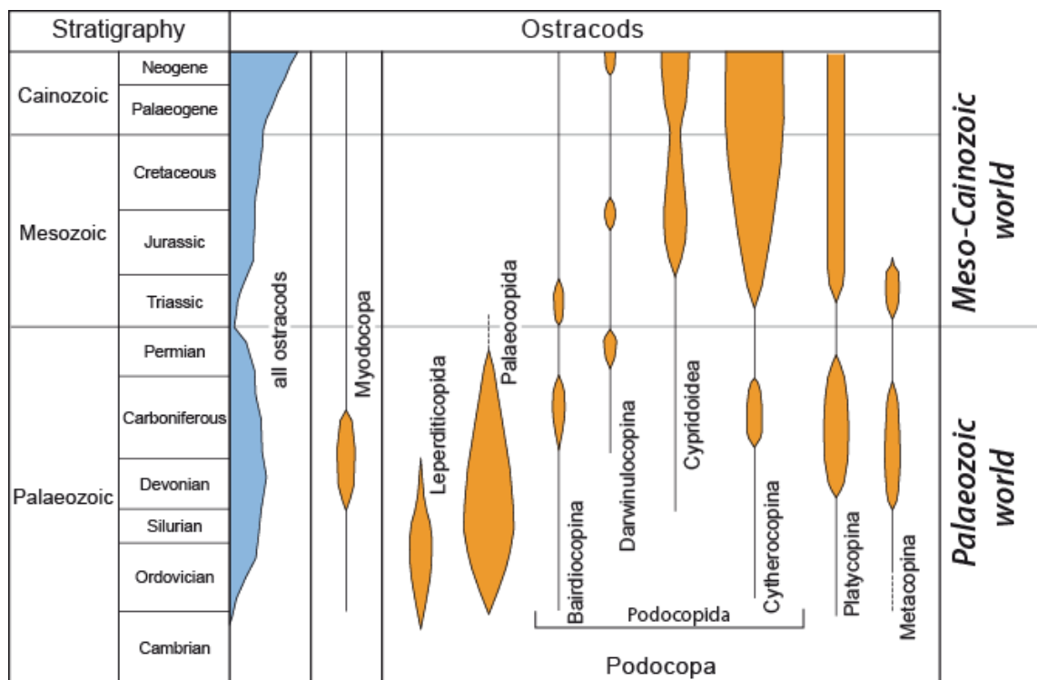
Figure 24 : Répartition stratigraphique des différents groupes d'ostracodes au cours du Phanérozoïque. Extrait de Crasquin & Forel (2014).
