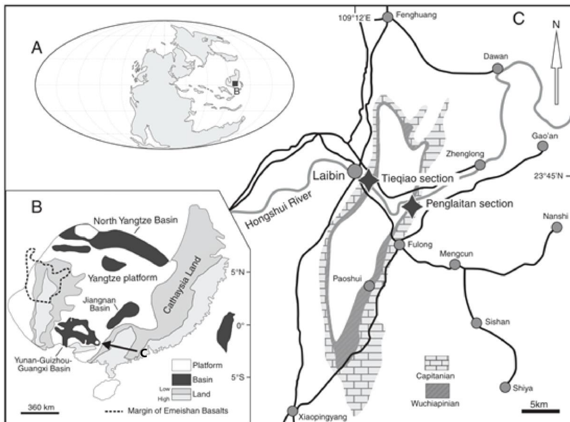
Figure 16 : A : Carte paléogéographique du Permien supérieur et localisation du bloc de Chine du Sud ; B : Paléogéographie du bloc de Chine du Sud au Wuchiapingien ; C : Localisation de la coupe de Penglaitan. Extrait de Chen et al. (2011).
