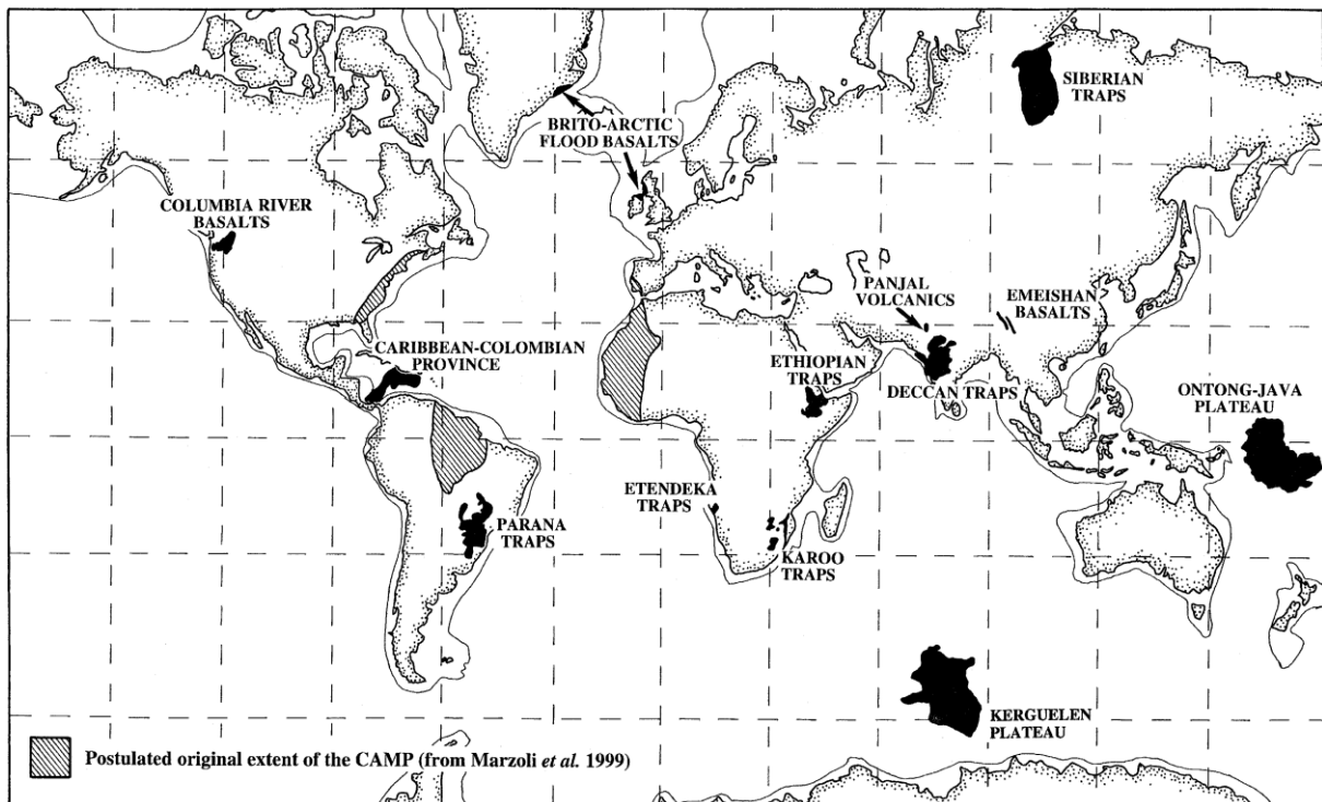
Figure 9 : Répartition géographique actuelle des principales provinces volcaniques. Extrait de Wignall 2001.
