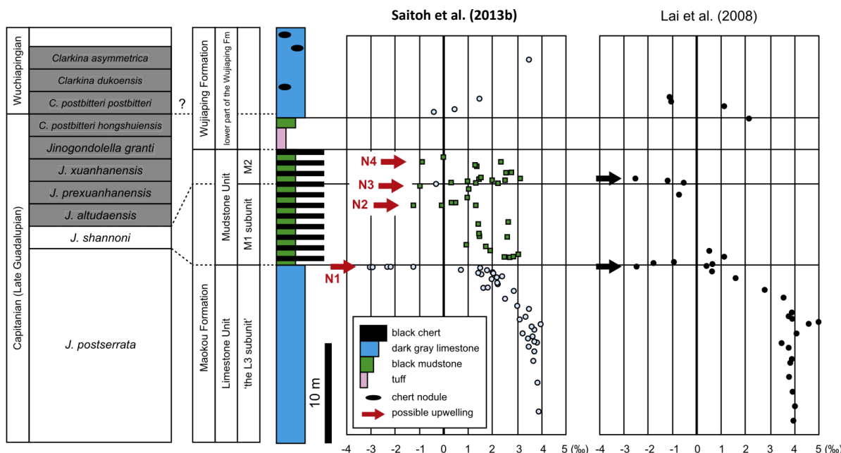
Figure 14 : Comparaison des données isotopiques ( \delta^{13}\text{C}_{\text{carb}} ) obtenues à Chaotian par Lai et al. (2008) et Saitoh et al. (2013b). D'après Saitoh et al. (2013b).
