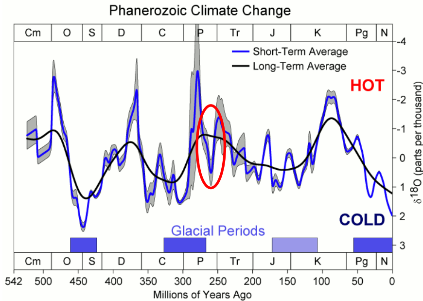
Figure 4: Diagramme représentant les variations du \delta^{18}\text{O} au cours du Phanérozoïque (Image issue de http://www.globalwarmingart.com ; simplifiée d'après Veizer et al. 2000).
