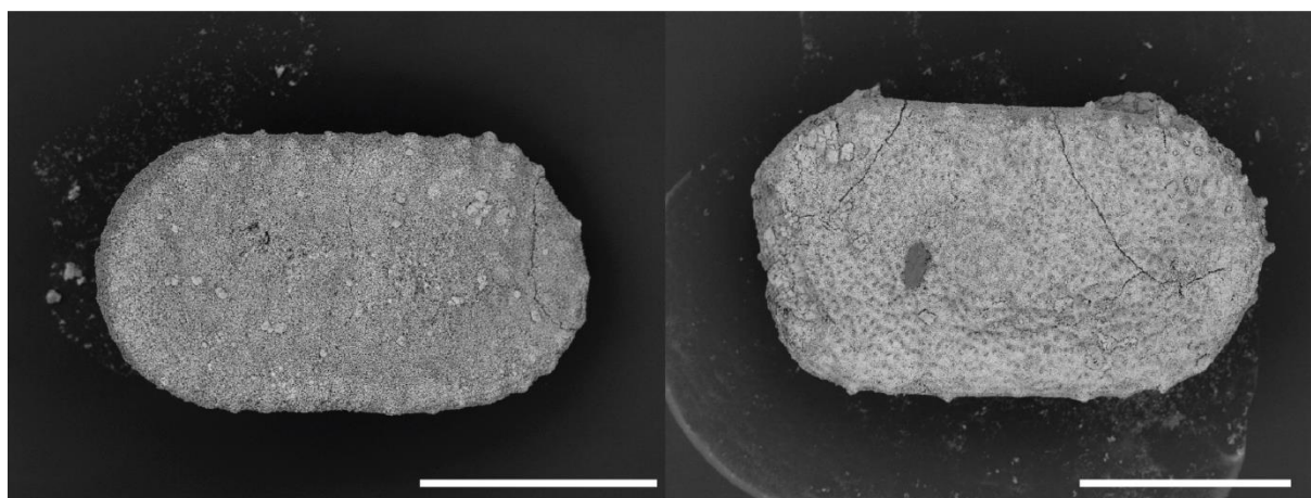
Figure 27 : Spécimens de Roundyella? suboblunga Wang, 1978. Valve entière à gauche, valve cassée à droite. Échelle égale à 300µm à gauche et à 400µm à droite.
