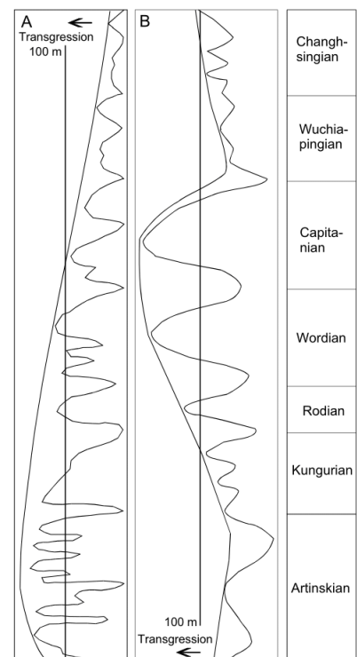
Figure 6 : Évolution du niveau marin au Permien. A : courbe du niveau marin global de Ross & Ross (1995), B : courbe du niveau marin en Chine du Sud de Chen et al. (1998). D'après de Mertmann (2003).
