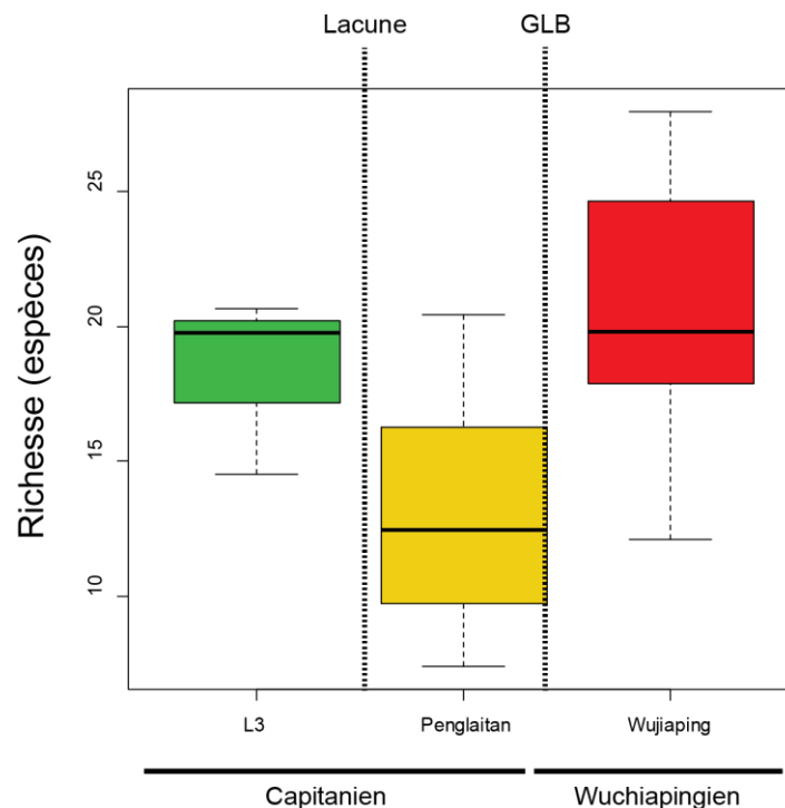
Figure 44 : Boxplot représentant la richesse spécifique standardisée par échantillon ( n=65 ). La boîte verte correspond à L3, la boîte jaune au Laibin Limestone (Penglaitan) et la boîte rouge à la formation Wujiaping.
