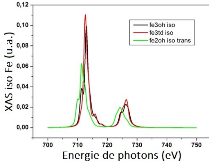
Figure 87: Courbes XAS théoriques calculées par P. Saintavit pour les ions \text{Fe}^{3+} et \text{Fe}^{2+} en sites octaédriques et tétraédriques.
