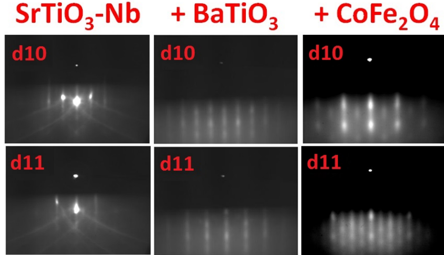
Figure 27: Clichés RHEED finsaux à chaque étape de la réalisation d'un échantillon d'un échantillon de 6 nm de \text{CoFe}_2\text{O}_4 sur 15 nm de \text{BaTiO}_3 sur \text{SrTiO}_3(\text{Nb}) . A gauche, le substrat de \text{SrTiO}_3 avant dépôt. Au milieu, les clichés pour \text{BaTiO}_3 en fin de dépôt, qui sont ceux sur lesquels \text{CoFe}_2\text{O}_4 sera déposé. A droite, clichés RHEED du spinelle \text{CoFe}_2\text{O}_4 en fin de dépôt. Les tiges spinelles sont bien visibles.
