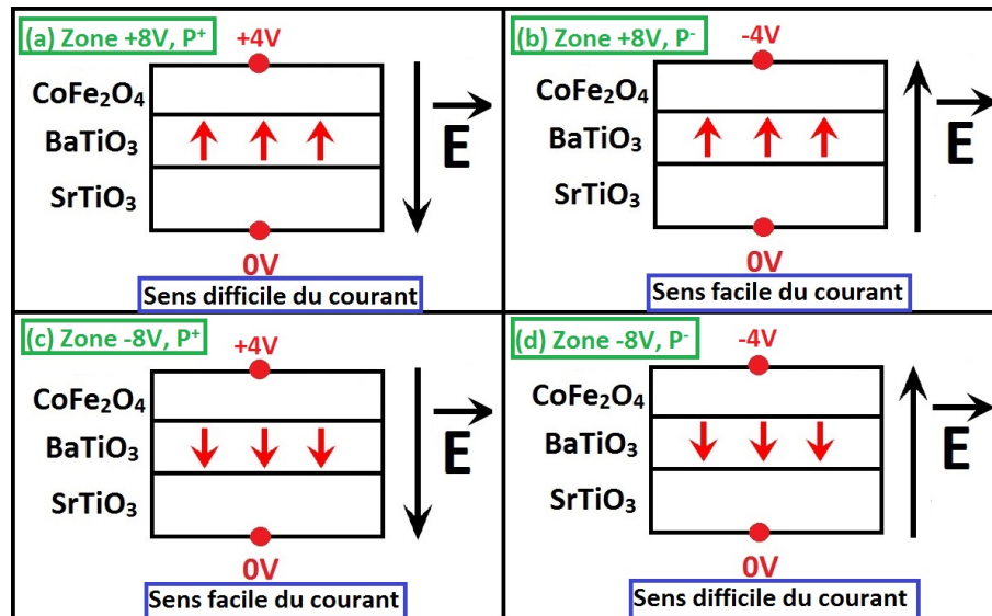
Figure 101: Sens de passage facile ou difficile du courant selon la direction de polarisation de BaTiO_3 et le potentiel appliqué par la pointe à la surface de l'échantillon V_{\text{pointe}} . Les cas (b) et (c) permettent d'obtenir un courant plus élevé que (a) et (d), donc une résistance électrique plus faible.
