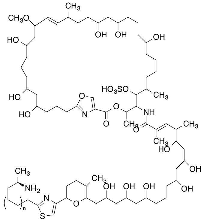
théonézolide A (T17) n = 1 théonézolide B (T18) n = 2 théonézolide C (T19) n = 3
