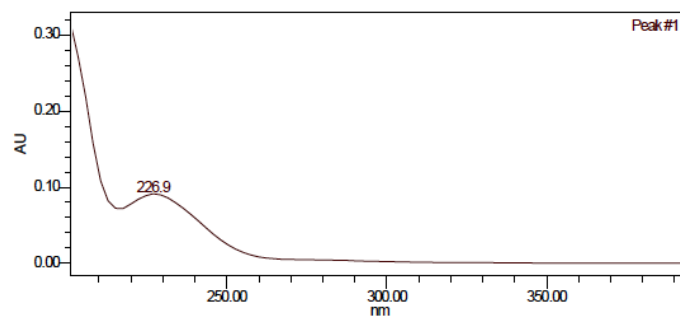
Spectre UV du composé HF1
