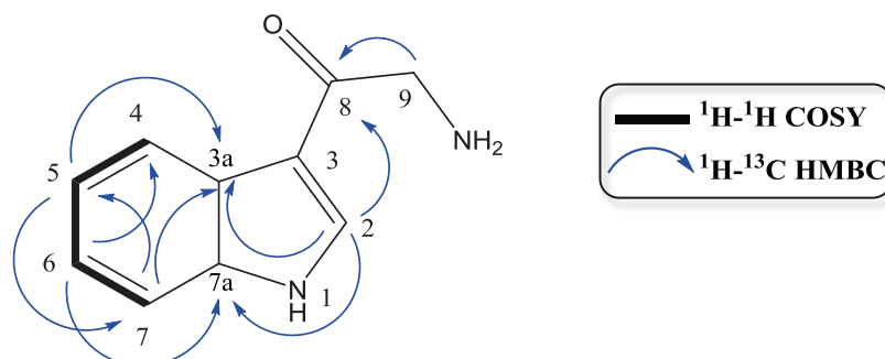
Figure 32 : Corrélations RMN 2D clés du métabolite FR2 .
