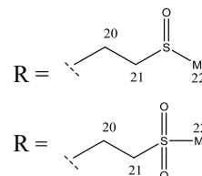
Dérivé sulfoné du waiakéamide ( H46 )
