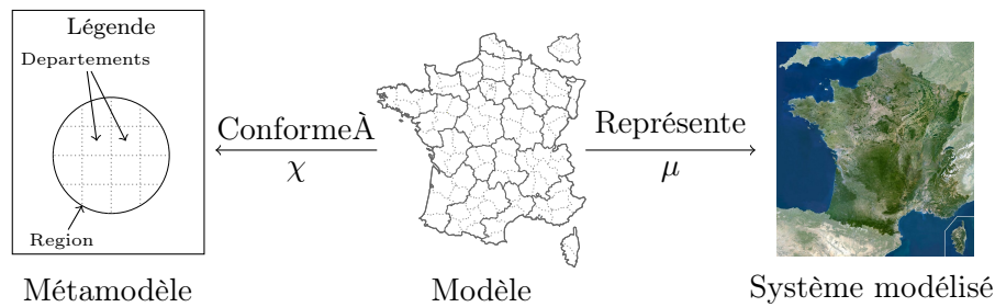
FIGURE 3.3 – Relations entre système, modèles, métamodèle et langage de modélisation [2006-1]
