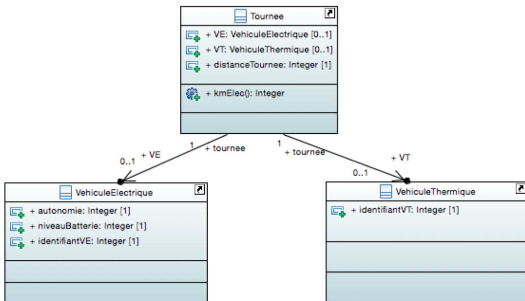
FIGURE 5.9 – Aspect information de la vue fonctionnelle modélisé sous la forme d'un diagramme de classes fUML avec Papyrus
