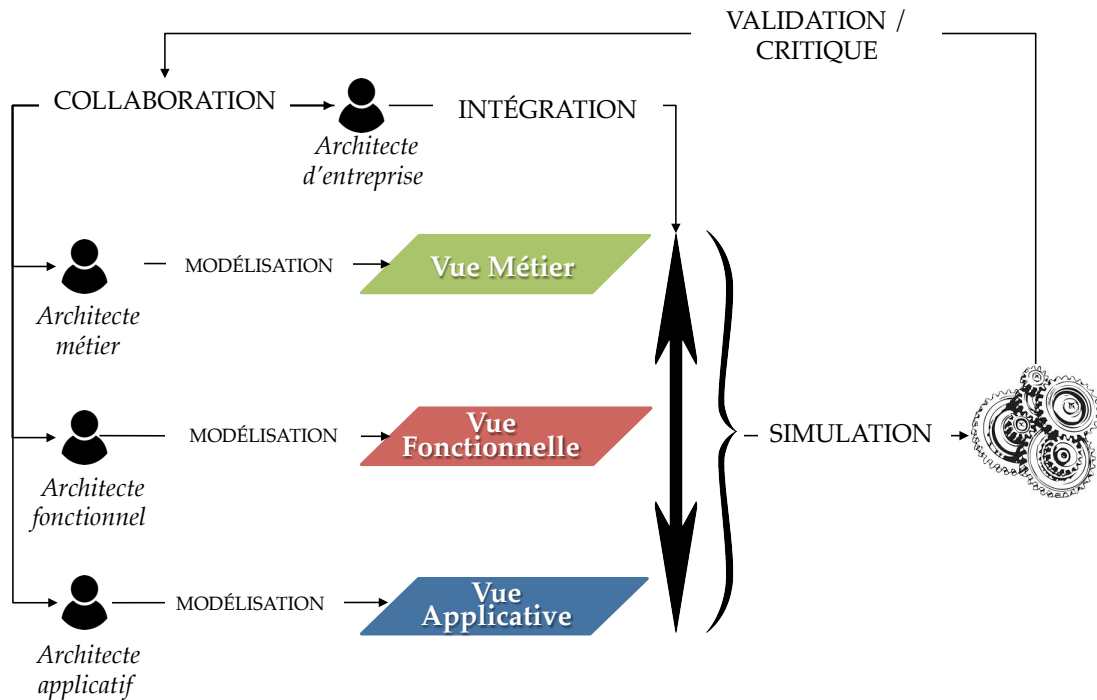
FIGURE 4.12 – Approche conceptuelle du framework ExecuteEA
