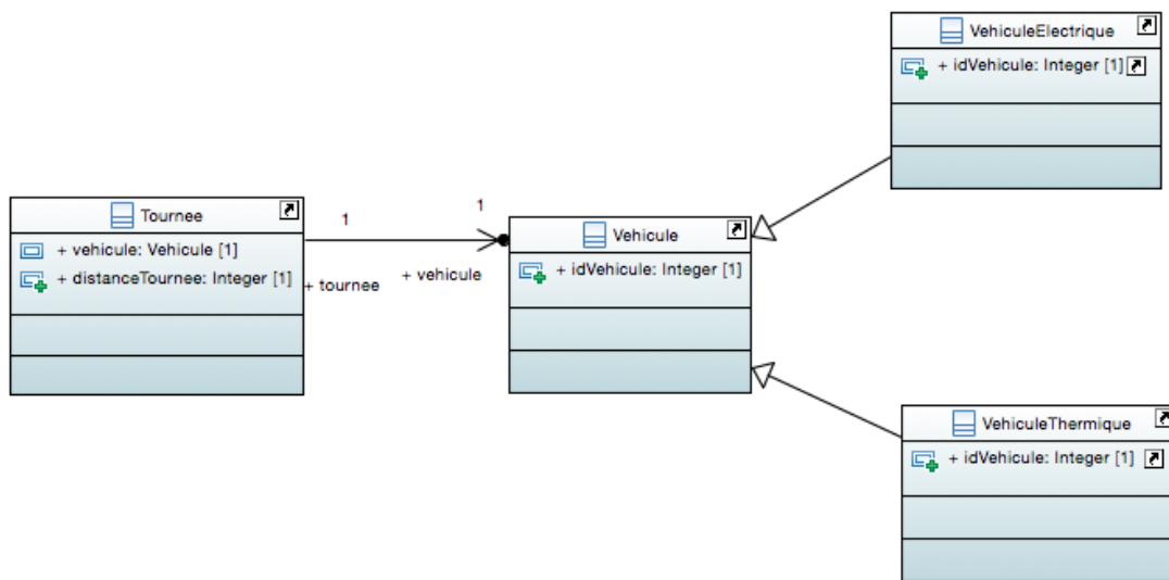
FIGURE 5.8 – Aspect information de la vue métier modélisé sous la forme d'un diagramme de classes fUML avec Papyrus
