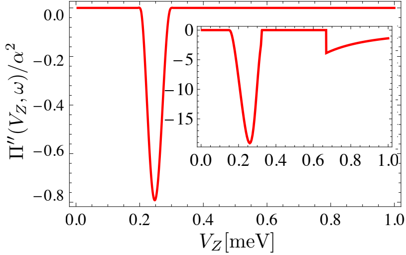
Figure E.3: La partie imaginaire de la susceptibilité électronique [\Pi''(\omega)] en tant qu'une fonction de l'énergie Zeeman V_Z pour un nanofil avec interaction spin-orbite dans le cas de conditions périodique aux limites ayant les paramètres L = 2 \mu\text{m} , t = 0.5 \cdot 10^{-2} \text{ eV} , \alpha = 0.4 \text{ meV} , \mu = -10^{-2} \text{ eV} , \Delta = 0.25 \text{ meV} , N = 80 , et \omega = 0.1 \text{ meV} ( \omega = 0.2 \text{ meV} dans l'encart). La transition topologique a lieu pour V_Z \approx 0.25 \text{ meV} , pour lequel la susceptibilité atteint son maximum. L'émergence d'un deuxième pic est due à la condition de résonance autours de gaps extérieurs ( k \sim k_F ).
