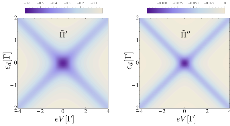
Figure E.2: \tilde{\Pi}'(\omega) \equiv \Pi'(\omega)/(\beta_L - \lambda)^2 (à gauche) et \tilde{\Pi}''(\omega) \equiv \Pi''(\omega)/(\beta_L - \lambda)^2 (à droite) en fonction de eV et \epsilon_d pour \beta_L = \beta_R , \Gamma_L = \Gamma_R = 0.5 et \omega = 0.1 . Toutes les énergies sont exprimées en termes de \Gamma = \Gamma_L + \Gamma_R .
