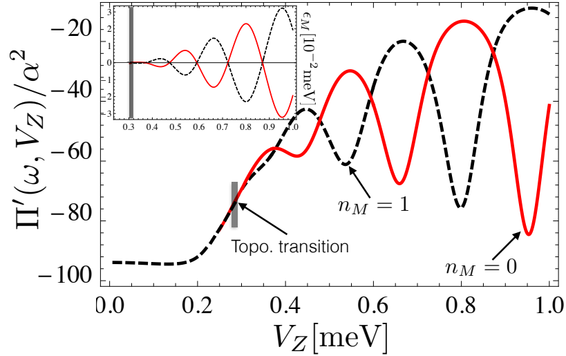
Figure E.4: Dépendance entre \Pi'(\omega, V_Z) et l'énergie Zeeman V_Z . Au dessus de la transition topologique (indiqué sur l'image), les courbes rouge (continue) et noire (pointillée) correspondent à \Pi'(\omega, V_Z) pour respectivement la parité n_M = 0 et n_M = 1 . \Pi'(\omega, V_Z) comprend des oscillations en tant que fonction de V_Z . Ces oscillations ont des amplitudes différentes pour les parités n_M = 0, 1 (mais les périodes égales) et se croisent dans les points où \epsilon_M = 0 (voir l'encart). Au dessous de la transition topologique, la susceptibilité reproduit celle des conditions périodiques aux limites. Nos paramètres sont [8]: L = 2\mu\text{m} , t = 0.5 \cdot 10^{-2}\text{eV} , \alpha = 0.4\text{meV} , \mu = -10^{-2}\text{eV} , \Delta = 0.25\text{meV} , \omega = 0.02\text{meV} , and N = 80 .
