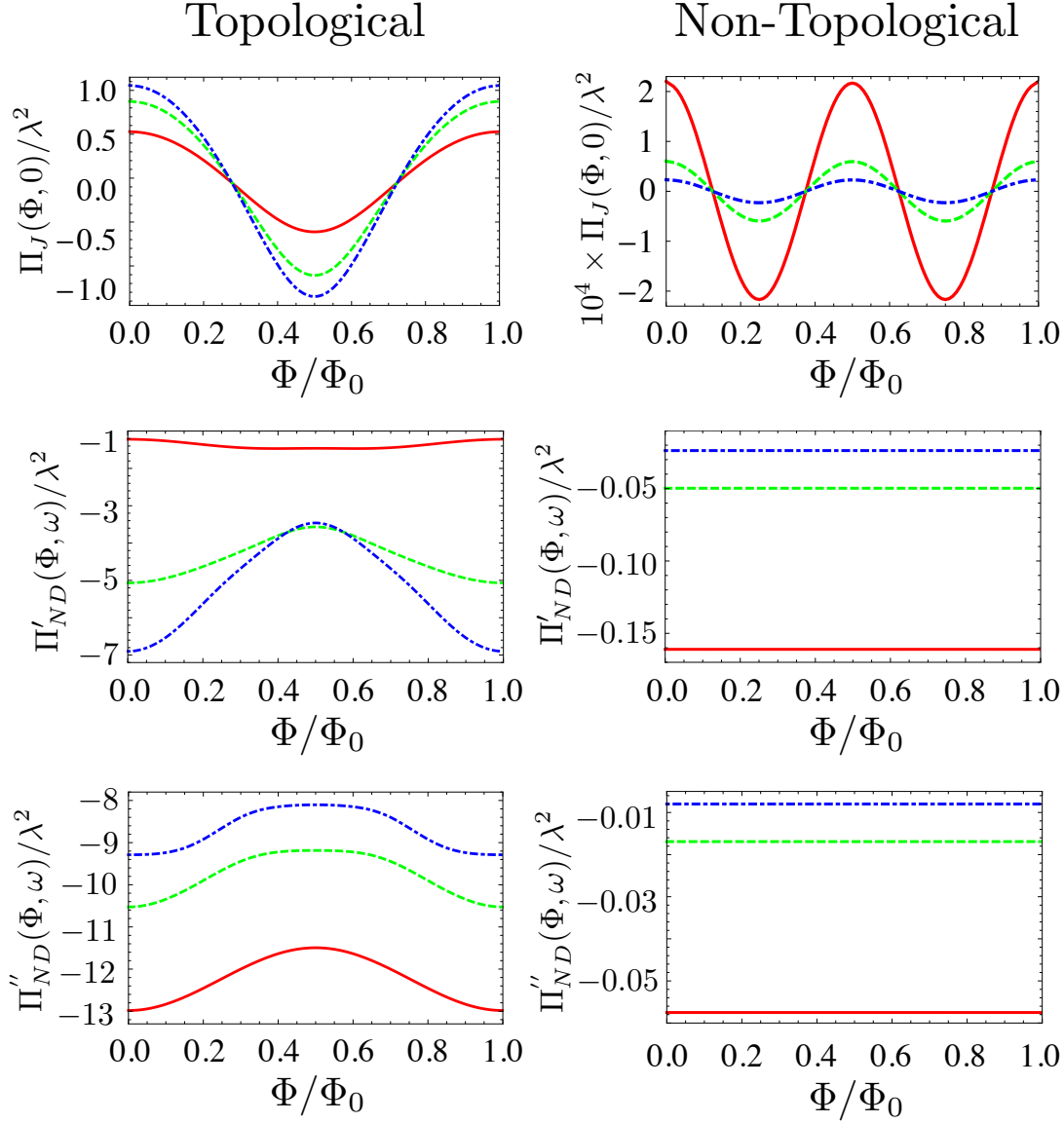
Figure E.5: Colonne gauche (colonne droite), de haut en bas: dépendance entre la susceptibilité de Josephson, les parties réelle et imaginaire de la susceptibilité non-diagonale et le flux magnétique \Phi/\Phi_0 pour f_M = 0 , dans la région topologique (non-topologique). Les lignes rouge, verte et bleue correspondent respectivement à \mu = -1.5 ( \mu = -2.5 ), \mu = -1 ( \mu = -3 ), et \mu = -0.5 ( \mu = -3.5 ). Le point de transition de phase est \mu = -2 . Les paramètres sont \Delta = 0.1 , t' = 0.2 , N = 50 et toutes les énergies sont exprimées en termes de t = 1 .
