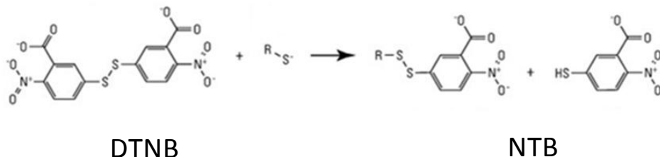
Figure 17 : Réaction de liaison du réactif d'Ellman avec un composé soufré (R-S-). Cette réaction donne lieu à la production d'une molécule de NTB quantifiable par la mesure de l'absorbance du mélange à 412 nm.
