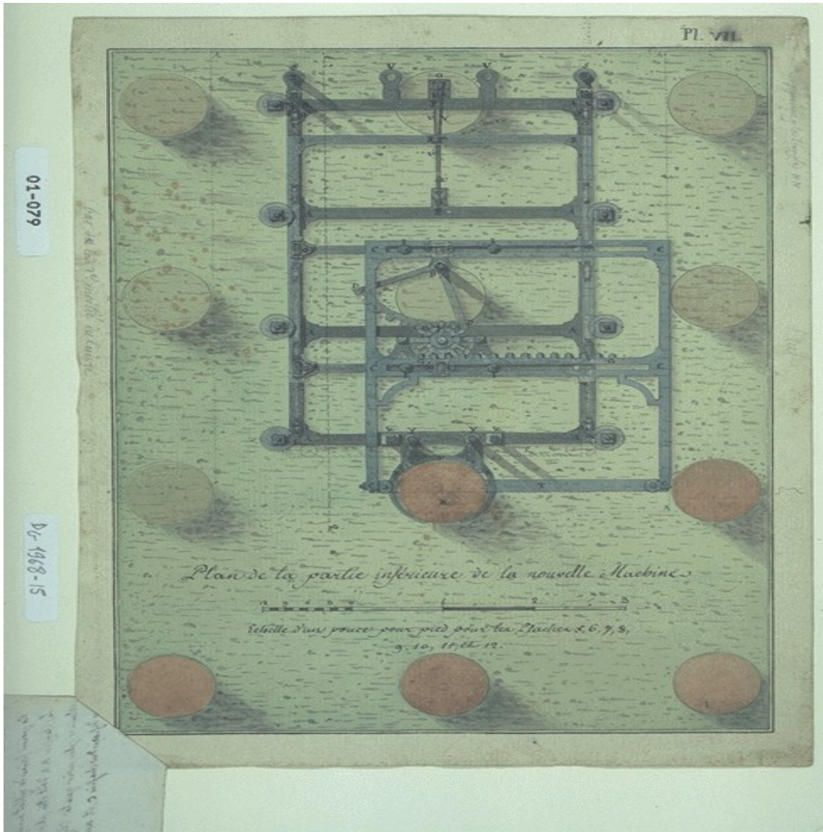
Figura 4 J. Dillon, Plan de la partie inférieure de la nouvelle machine à réceper les pieux dans l'eau (2) , 1791
