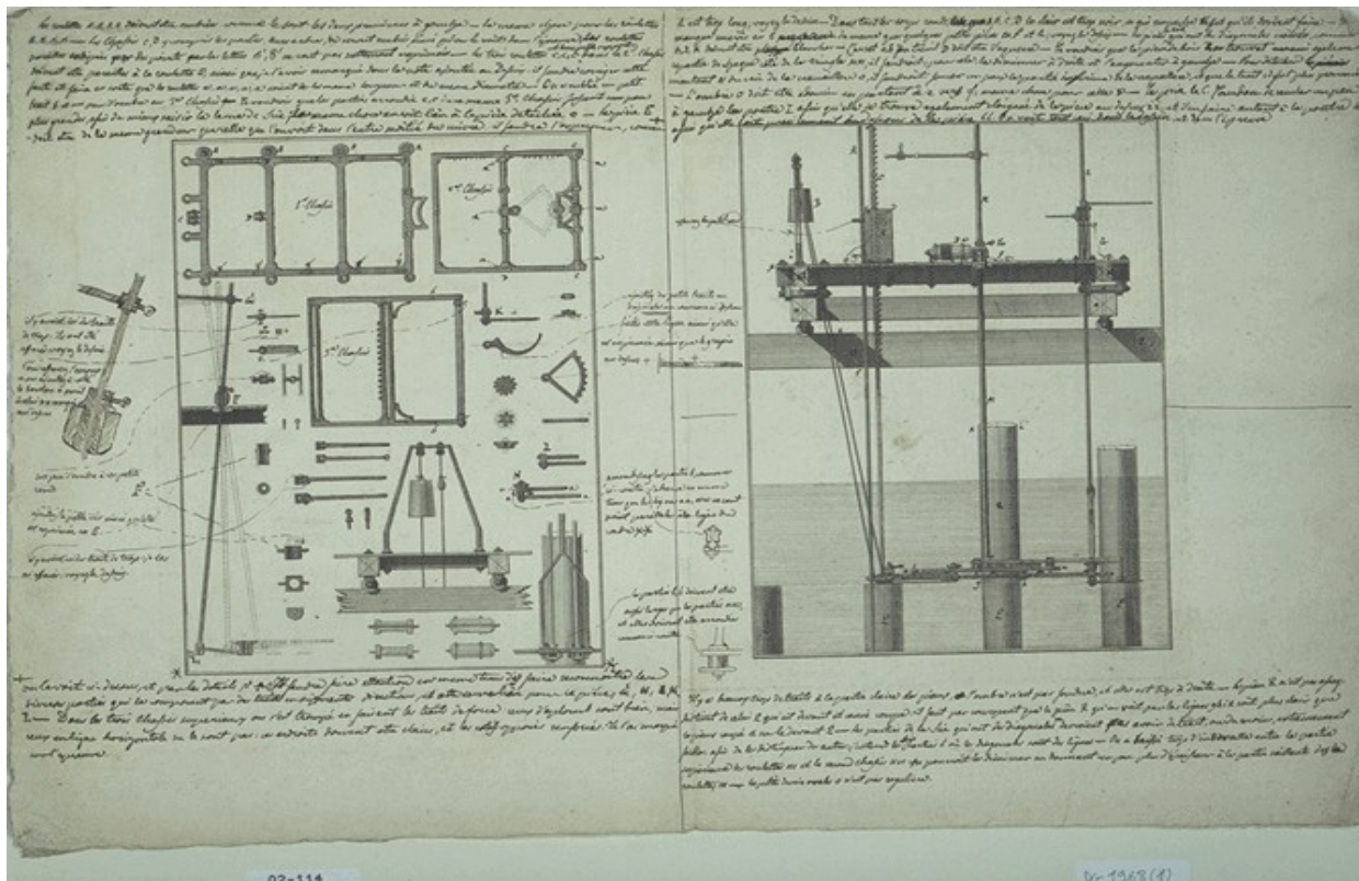
Figura 12 J. Dillon, Elément métallique de la machine à réceper les pieux dans l'eau , 1791
