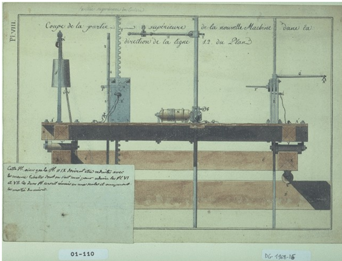
Figura 5 J. Dillon, Coupe de la partie supérieure de la nouvelle machine à recevoir les pieux dans l'eau dans la direction de la ligne 1. 2 du plan (1) , 1791
