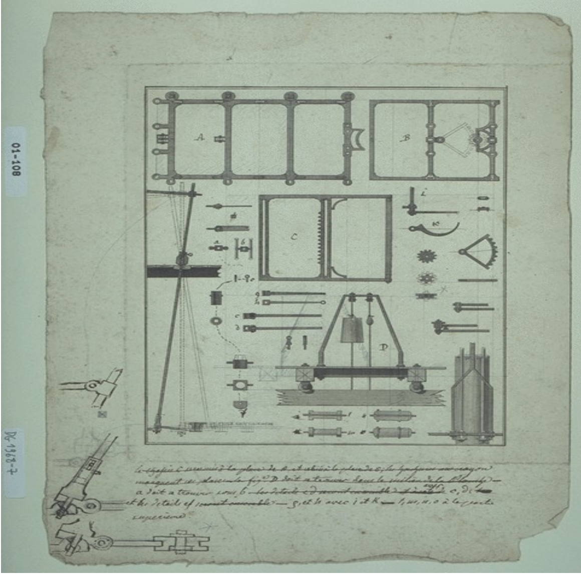
Figura 11 J. Dillon, Machine à réceper les pieux dans l'eau. Outils, 1791
