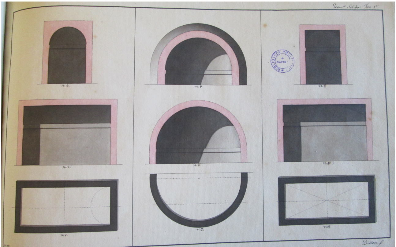
Figura 44 G. Dillon, Lezioni di disegno geometrico, Geometria solida, Tavola 5 , disegni 1–2–3 Pianta e spaccati in punto reale della volta a botte; disegni 4–5–6 Lo stesso in quella a croce; disegni 7–8–9 Lo stesso in quella a cupola, 1790
