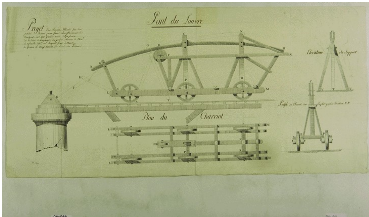
Figura 30 J. Dillon, Pont du Louvre: plan, coupe, profil et élévation du charriot pour le transport des 130 grandes arches en fer fondu pour former les 9 arches du pont du Louvre, 1801 – 1803
