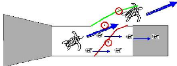
Système de grille adapté au chalut, avec une porte de sortie pour les tortues Détail du dispositif Flip-TED et BFD-FES. La Grille Nordmore peut remplacer le TED Grille ou TED comme Turtle Excluder Device (Source : IFREMER)
