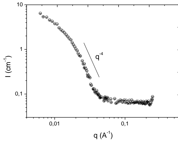
Figure II.17 : Spectre DNPA des nanoparticules PEG- b -PMA t Bu à 0,25 mg/mL dans 100 % de D 2 O
