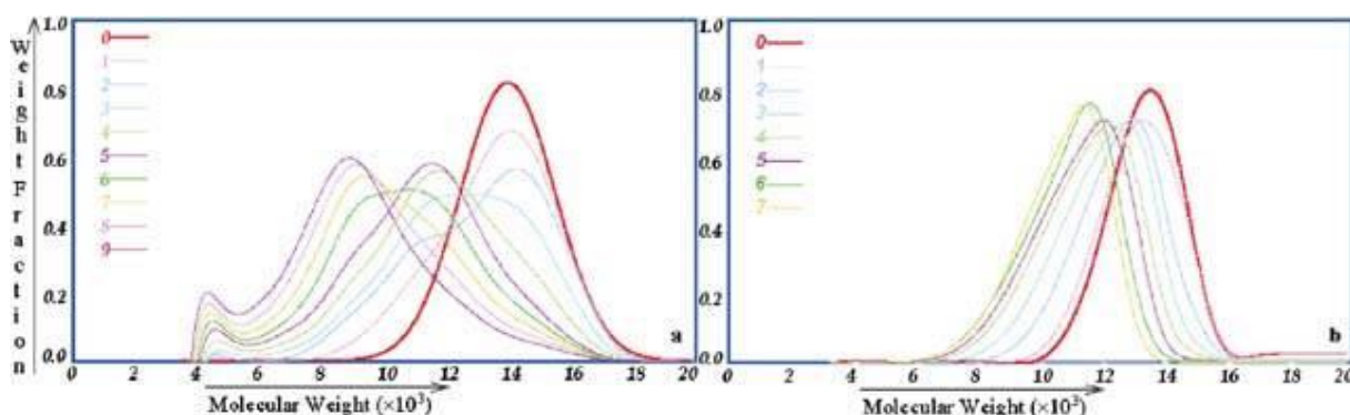
Figure V.15 : Evolution des spectres théoriques des masses molaires des polymères ( M ) en fonction de la fraction en poids ( \phi_M ) avec une distribution normale en taille initiale pour des coupures pourcentages de 5 % à 30 % (a) et de 5 % à 10 % (b)
