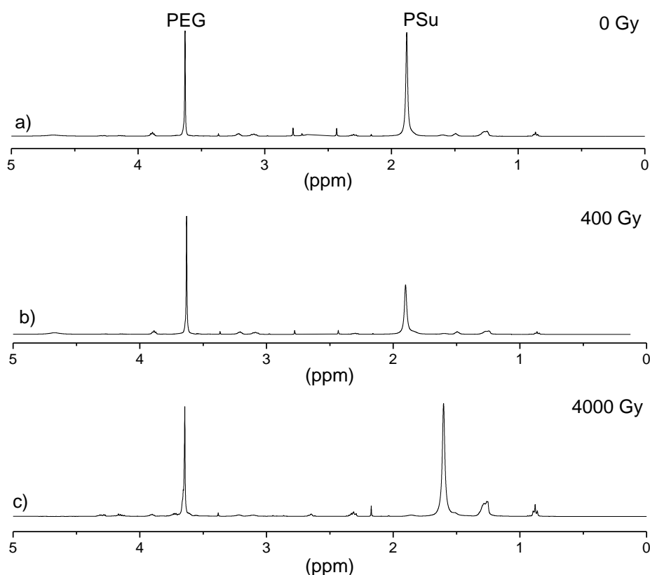
Figure III.23 : Spectres RMN 1 H dans le CDCl 3 des copolymères PEG- b -PSu après irradiation en milieu désoxygéné
