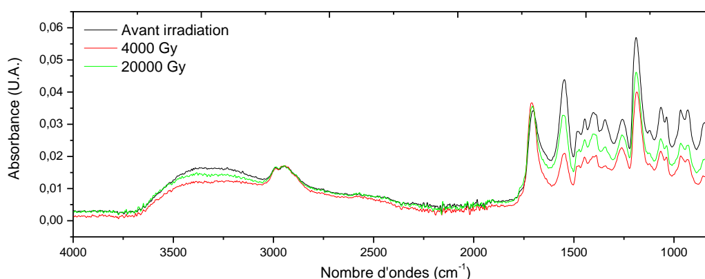
Figure V.7 : Spectres infrarouge des couronnes de polymères des NPs Au-PMAA-2 après irradiation
