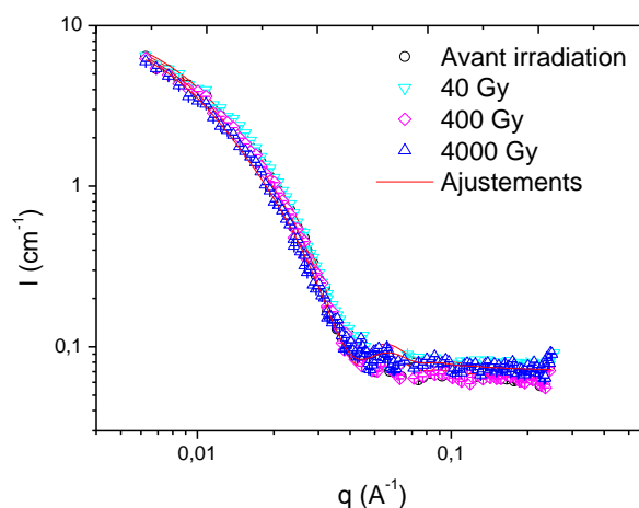
Figure III.8 : Spectres DNPA des micelles PEG- b -PMAtBu après irradiation en milieu oxygéné et leur courbe d'ajustement
