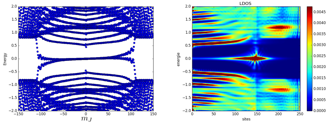
FIGURE 4.3 – Phase hélicale. Dispersion en m_J et LDOS pour les paramètres \mu = 10 , t = 25 , \Delta_S = 3 , \Delta_R = 2 .
