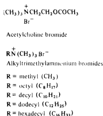
Figure 3 : Dérivés de sels d'alkylammonium testés, d'après [43]
