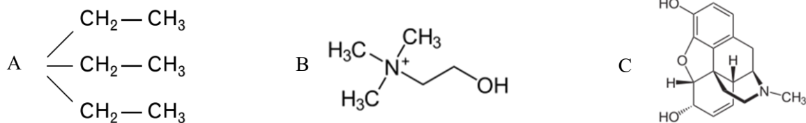
Figure 2 : Structure biochimique A/ de la triéthylamine N(CH_2CH_3)_3 , B/ de la choline C_5H_{14}NO et C/ de la morphine C_{17}H_{19}NO_3 .
