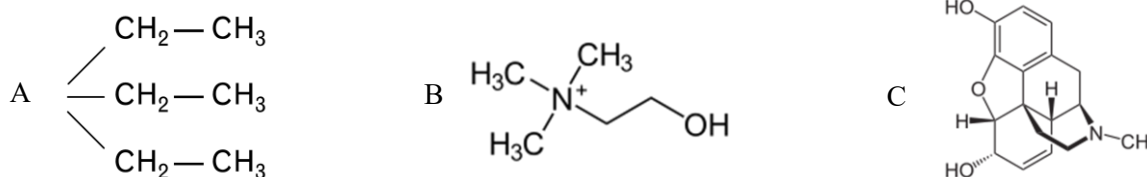
Figure 2 : Structure biochimique A/ de la triéthylamine N(CH_2CH_3)_3 , B/ de la choline C_5H_{14}NO et C/ de la morphine C_{17}H_{19}NO_3 .
