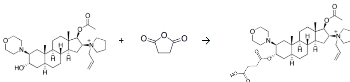
Figure 8 : Réaction de production de rocuronium--COOH : mise en présence de rocuronium et d'anhydride succinique .
