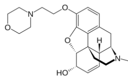
Figure 22 : Structure chimique de la pholcodine.
