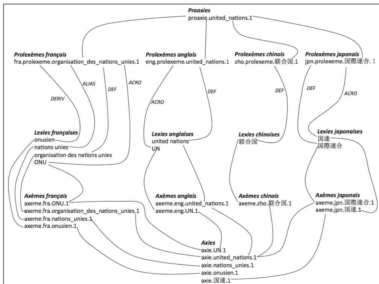
Figure 65 : Modélisation complète de l'exemple organisation des nations unies dans PIVAX-3
