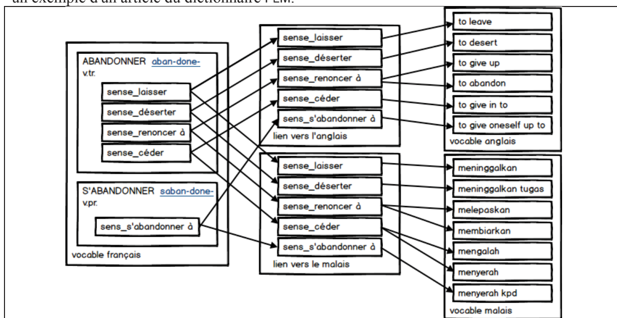
Figure 1 : Exemple de structure "furcoïde" d'un article du dictionnaire FEM
