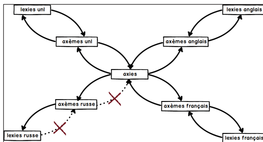
Figure 31 : Problèmes de la ressource de V. Dikonov
