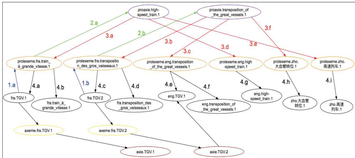
Figure 56 : Exemple de calcul des liens dans PIVAX-3
