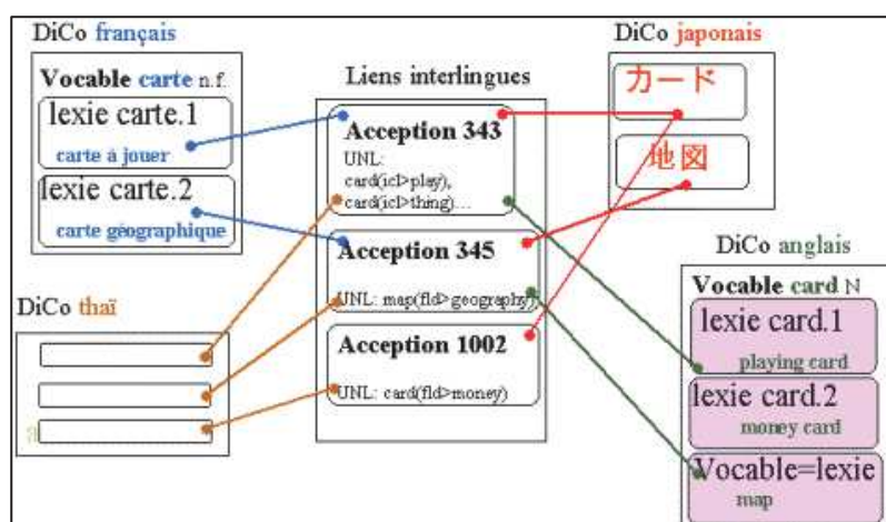
Figure 12 : Macrostructure du dictionnaire PAPILLON-NADIA
