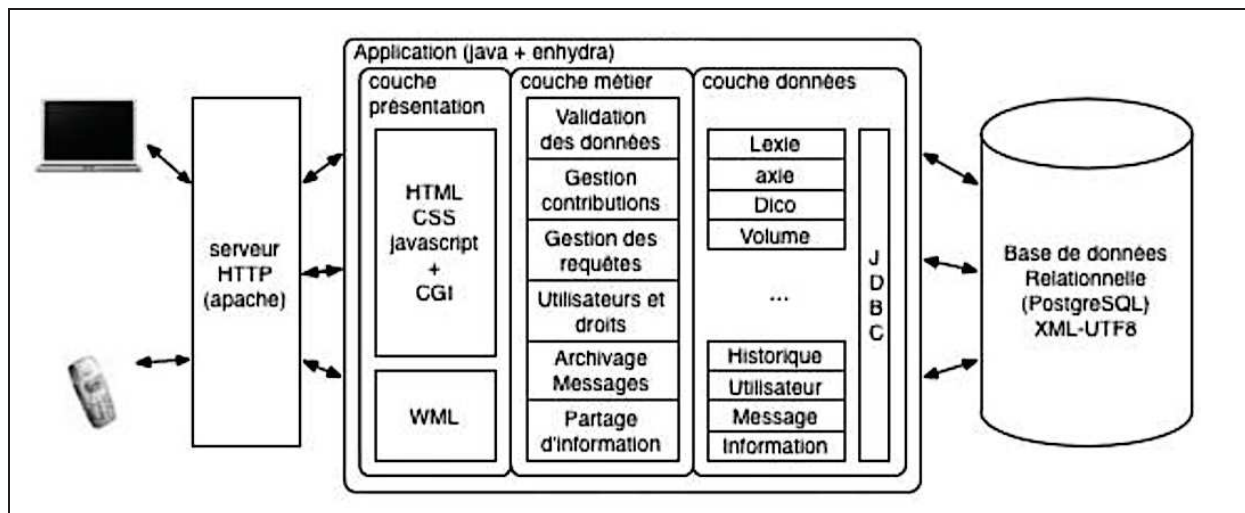
Figure 8 : Architecture à 3 couches de la plate-forme JIBIKI
