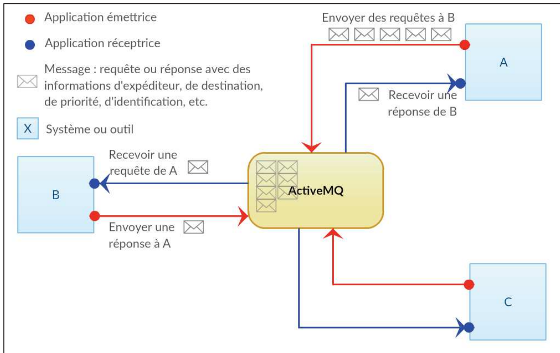
Figure 73 : Architecture "client- serveur" de gestion de travaux en utilisant ACTIVEMQ
