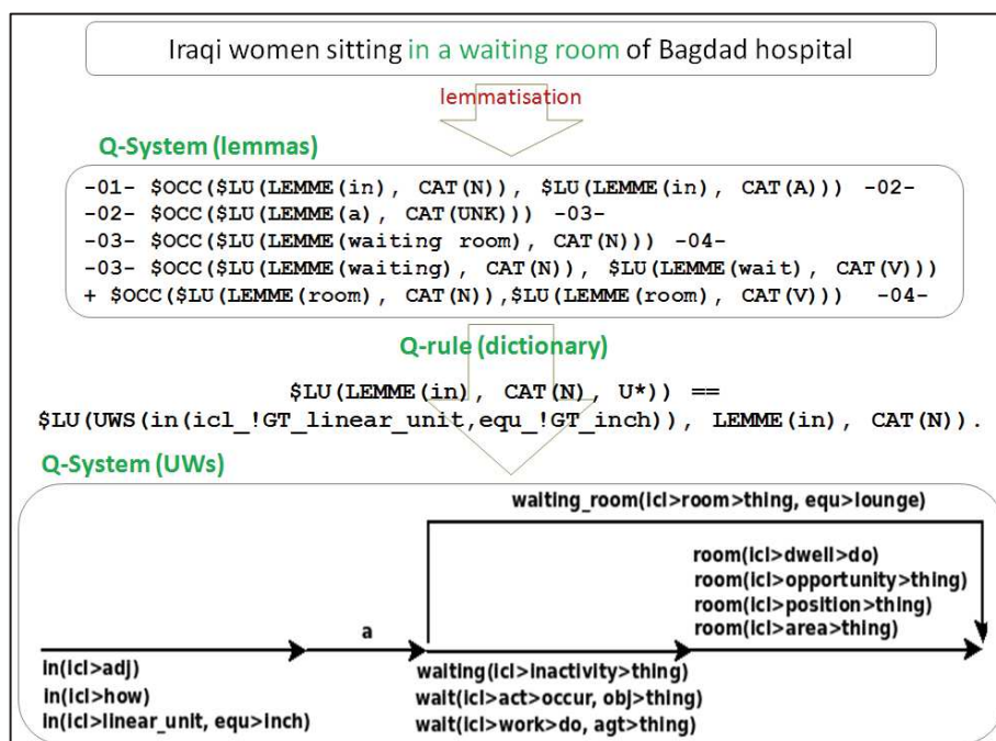
Figure 22 : Exemple d'annotation de texte dans OMNIA
