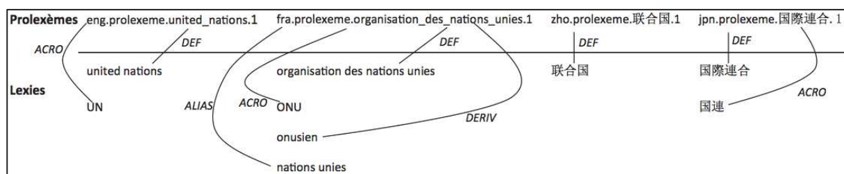
Figure 61 : Liens entre les prolexèmes et les proaxies
