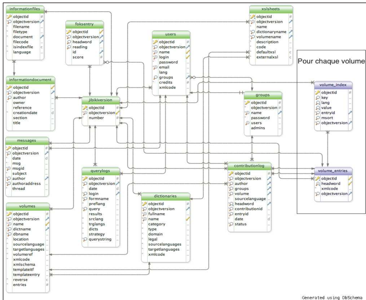
Figure 25 : Schéma de la base de données de JIBIKI-1
