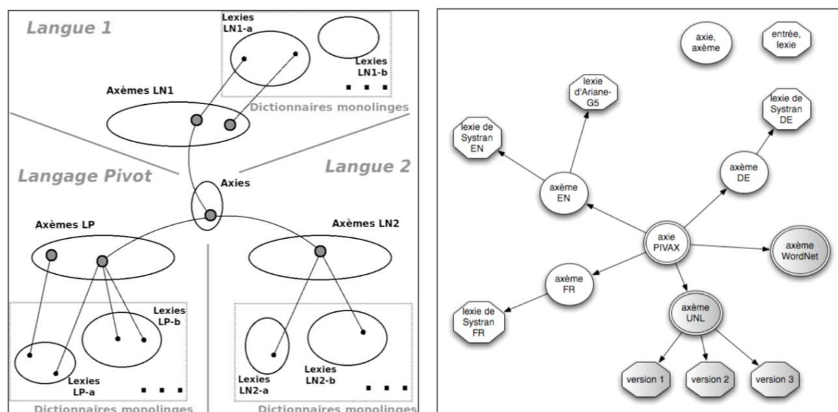
Figure 17 : Macrostructure de PIVAX et exemples de volumes
