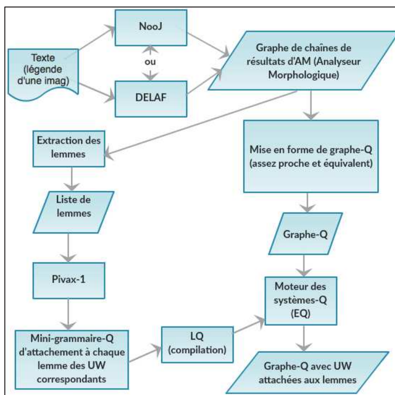
Figure 21 : Processus de traitement du projet OMNIA
