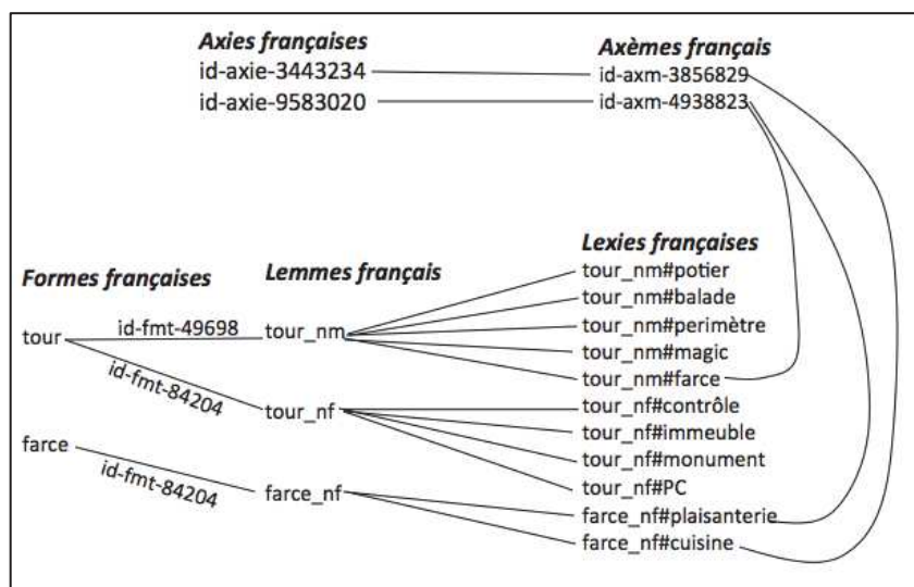
Figure 71 : Modélisation de BDLex pour LEXINNOVA
