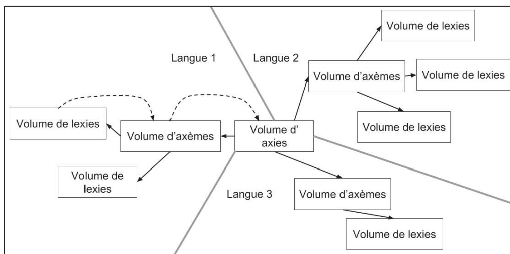
Figure 19 : Algorithme de calcul des liens dans PIVAX-1
