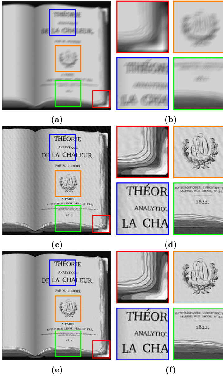
Figure 1.10 – Un exemple de déconvolution (1.45) montrant l'importance de la méthode de seuillage. En haut l'image dégradée avec un flou de mouvement et un bruit Gaussien i.i.d. de niveau 5 \cdot 10^{-3} le \text{pSNR} = 17.85\text{dB} . Les deux matrices \Theta ont été construites avec le même nombre de coefficients (qui correspond à 57 opérations par pixels). Au milieu : la méthode de seuillage simple \text{pSNR} = 23.71\text{dB} . En bas : le seuillage pondéré (1.41), \text{pSNR} = 24.07\text{dB} . Au delà de l'augmentation du \text{pSNR} , on observe que les artefacts de restauration sont réduits significativement.
