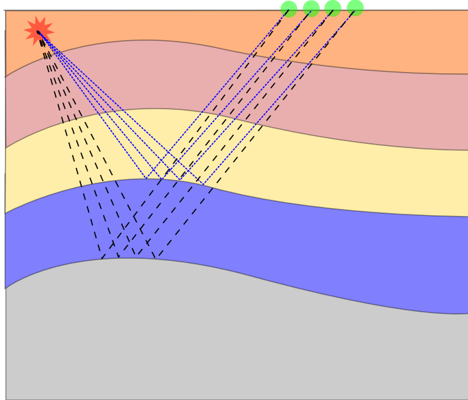
Figure 1.5 – Schématisation d'une prospection géophysique sur Terre. Les couches de différentes couleurs représentent la stratification de la croûte terrestre. Des chocs ou des vibrations sonores sont générés (étoile rouge) et se propagent dans les couches géophysiques. Les ondes peuvent être réfractées ou réfléchies et sont recueillies en surface par les capteurs en vert.
