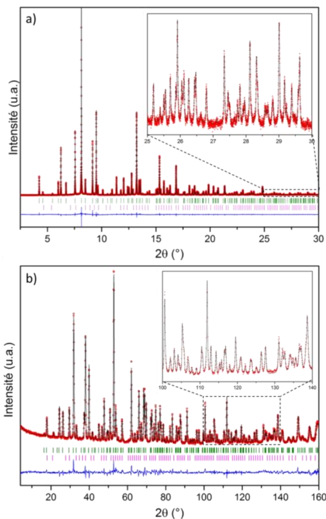
Figure IV.30 : Affinement Rietveld final des données synchrotron (a) et neutrons (b) de la céramique de \text{Sr}_{0,6}\text{Tb}_{1,4}\text{Ga}_3\text{O}_{7,2} ( R_{wp} = 5,91\% , R_p = 6,25\% et GOF = 1,36 pour le synchrotron). Les profils observé (en rouge), calculé (en noir) et différence (en bleu) sont présentés. Les lignes vertes et roses correspondent respectivement aux indexations de la mélanite \text{Sr}_{0,6}\text{Tb}_{1,4}\text{Ga}_3\text{O}_{7,2} et du grenat \text{Tb}_3\text{Ga}_5\text{O}_{12} .
