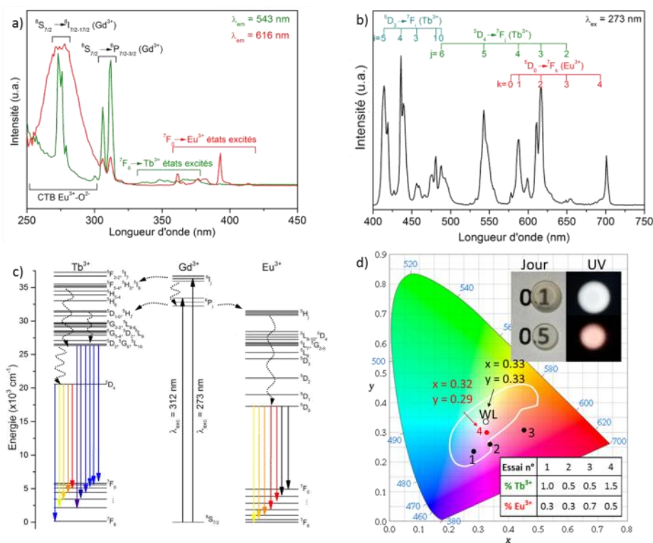
Figure IV.21 : a) Spectres d'excitation de \text{SrGa}_3\text{O}_7:1,5\%\text{Tb}^{3+}; 0,5\%\text{Eu}^{3+} enregistrés en monitorant les bandes d'émission caractéristiques de \text{Tb}^{3+} à 543 nm (en vert) et \text{Eu}^{3+} à 616 nm (en rouge). b) Spectres d'émission de \text{SrGa}_3\text{O}_7:1,5\%\text{Tb}^{3+}; 0,5\%\text{Eu}^{3+} sous excitation à 273 nm. c) Diagramme des niveaux d'énergie des ions \text{Gd}^{3+} , \text{Tb}^{3+} et \text{Eu}^{3+} . d) Diagramme de chromaticité de \text{SrGa}_3\text{O}_7:x\text{Tb}^{3+}, y\text{Eu}^{3+} , où les coordonnées de différents essais sont rapportées (excitation à 273 \pm 2 \text{ nm} .) La photographie représente des céramiques de \text{SrGa}_3\text{O}_7:1,5\%\text{Tb}^{3+}, y\text{Eu}^{3+} ( y = 0,1 ou 0,5\% ) prises sous lumière du jour puis en utilisant une lampe UV commerciale fonctionnant à 312 nm.
