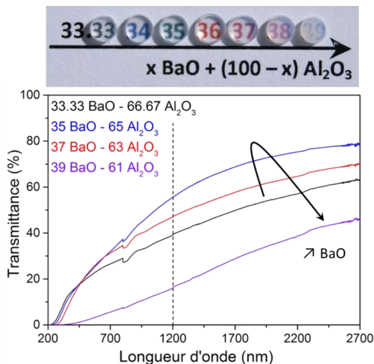
Figure III.32 : Photographie et courbes de transmittance des céramiques biphasiques de \text{BaO} - \text{Al}_2\text{O}_3 après normalisation de la transmittance pour 1 mm d'épaisseur.
