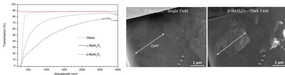
Figure 1.11 : Gauche : courbes de transmittance du verre et des deux polymorphes de \text{BaAl}_4\text{O}_7 . Droite : observations au MET de la microstructure de \text{BaAl}_4\text{O}_7 en modes champ clair et champ sombre.
