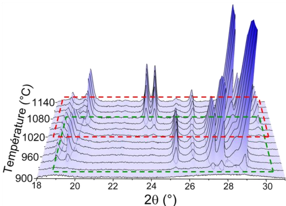
Figure II.2 : Diffraction de rayons X acquise in situ lors du chauffage d'un verre de composition 35 BaO – 65 Al 2 O 3 . On peut voir se former deux phases cristallines distinctes à partir de 920 °C (en vert) puis 1050 °C (en rouge).
