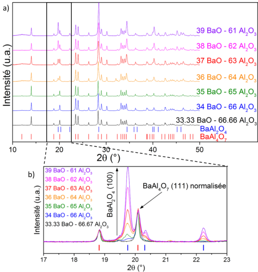
Figure III.18 : a) Diffractogrammes des rayons X pour des céramiques polycristallines de x \text{ BaO} - (100-x) \text{ Al}_2\text{O}_3 . Les lignes rouges et bleues correspondent respectivement aux indexations des phases \text{BaAl}_4\text{O}_7 et \text{BaAl}_2\text{O}_4 . b) Agrandissement de la zone 17-23 ^{\circ}(2\theta) après normalisation de la raie (111) de \text{BaAl}_4\text{O}_7 . L'augmentation du pic de \text{BaAl}_2\text{O}_4 est directement liée à la quantité de BaO dans le verre.
