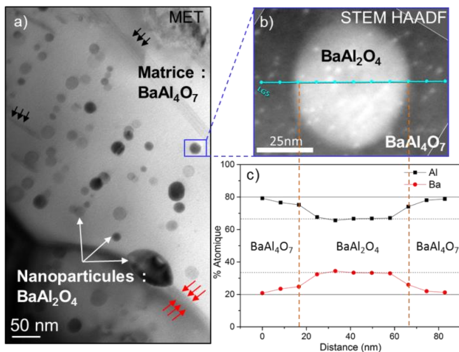
Figure III.24 : a) Micrographie MET en champ clair d'une céramique de composition 34 BaO – 66 Al 2 O 3 montrant la dispersion des nanoparticules de BaAl 2 O 4 dans les grains de BaAl 4 O 7 et au niveau des joints de grains. Les flèches noires pointent les fautes d'empilements et les rouges un joint de grains de BaAl 4 O 7 . b) Micrographie en mode STEM-HAADF et c) évolution de la composition le long de la ligne bleue traversant le grain de BaAl 4 O 7 et la nanoparticule de BaAl 2 O 4 . Les résultats sont obtenus à partir de pointés EDX. Sur le graphique, les traits pleins représentent la composition de BaAl 4 O 7 et les traits en pointillés celle de BaAl 2 O 4 .
