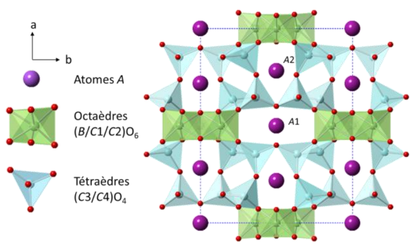
Figure III.3 : Projection de la structure de \text{A}_3\text{BC}_{10}\text{O}_{20} selon l'axe c . Les atomes A sont représentés par les sphères violettes dans les canaux pentagonaux ( A2 ) et hexagonaux ( A1 ), formés par les tétraèdres (\text{C}3/\text{C}4)\text{O}_4 en bleu et les octaèdres (\text{B}/\text{C}1/\text{C}2)\text{O}_6 en vert.
