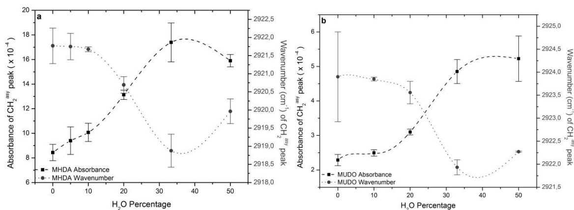
Figure 3.24: Absorbance et nombre d'onde des vibrations \nu\text{CH}_2^{\text{asy}} pour les SAMs constituées (a) de MHDA et (b) de MUODO en fonction du pourcentage d'eau dans la solution de thiols
