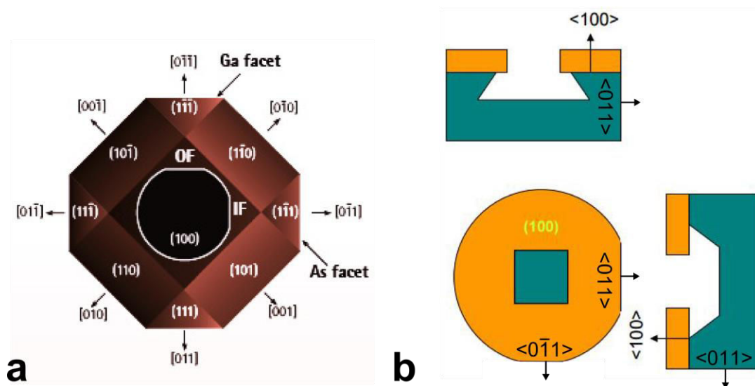
Figure 2.17: (a) Représentation des plans du GaAs en fonction de l'orientation du wafer et (b) exemple de gravure humide anisotrope d'un wafer de GaAs 204 .
