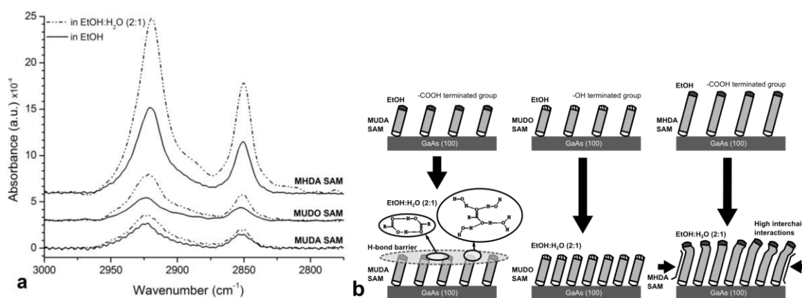
Figure 3.23: (a) Région \nu_{\text{CH}_2} du spectre IR des SAMs de MHDA, MU DO and MU DA formées dans l'éthanol ou dans le mélange EtOH:H 2 O (2:1) et (b) Schéma de principe des phénomènes lors de l'auto-assemblage des différentes monocouches dans l'éthanol et dans le mélange EtOH:H 2 O
