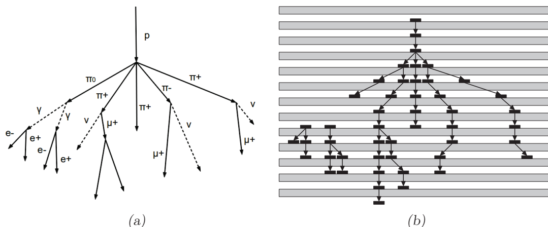
FIGURE 4.8 – (a) Illustration du développement d'une gerbe hadronique initiée par un proton. (b) La même gerbe hadronique telle qu'elle pourrait être détectée dans un calorimètre à échantillonnage à grande granularité. Les flèches suggèrent une reconstruction des gerbes hadroniques suivant une topologie en arbre orientée.
