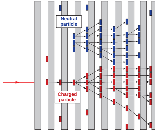
FIGURE 5.8 – Exemple de reconstruction finale d'une particule neutre (en bleu) et d'une particule chargée (en rouge) par l'algorithme ArborPFA dédié au SDHCAL.
