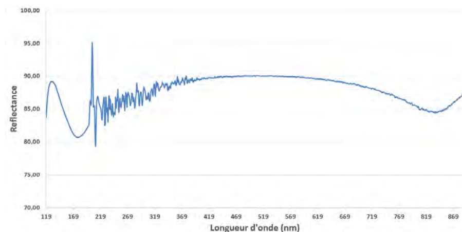
FIGURE B.1 – Réflectivité d'un miroir utilisant le traitement de surface en \text{MgF}_2 fournit par l'IOF.
