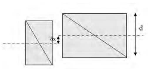
FIGURE 2.20 – Situation considérée pour étudier le décentrement relatif des prismes.
