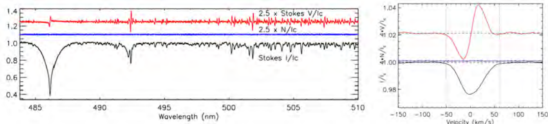
FIGURE 1.12 – Exemple de résultat obtenu grâce à la technique LSD. A gauche : morceau du spectre d'intensité (en bas), de la polarisation nulle (milieu) et de Stokes V (en haut). A droite : profils LSD correspondants. Ici la signature Zeeman de l'étoile HD 175362 obtenue avec des observations de l'instrument ESPaDOnS au CFHT (Wade et al., 2016).
