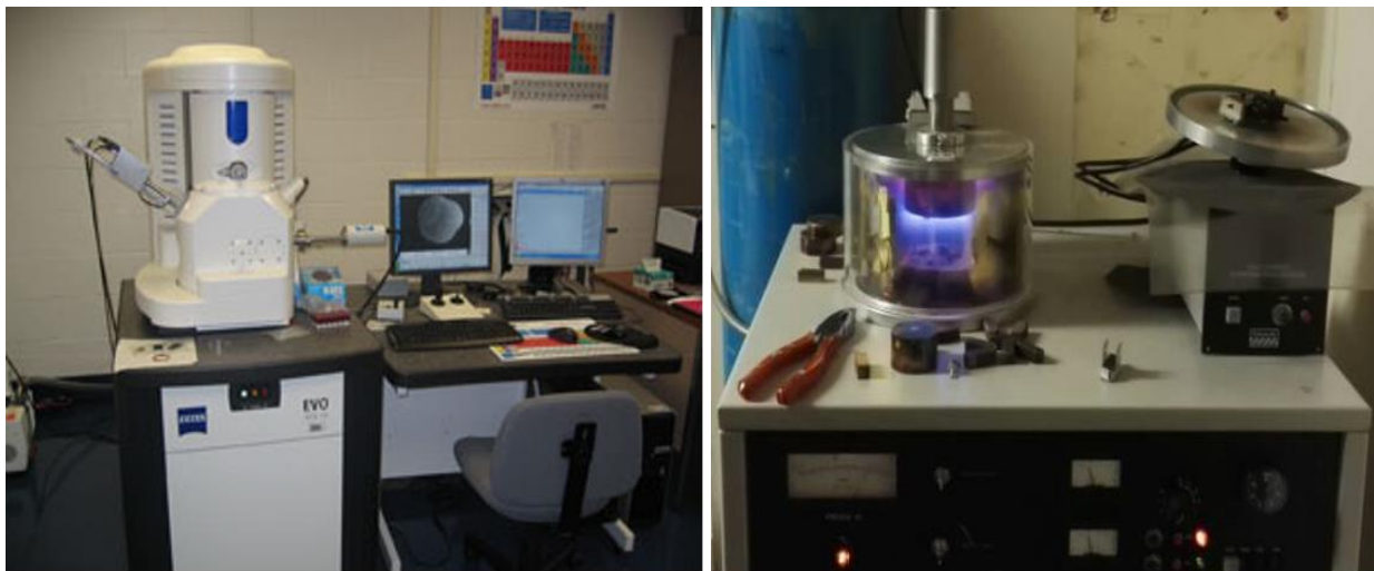
Figure 2.18 EVO MA10 SEM (left) and SC-6 Pelco Sputter Coater (Laboratoire Procédés et Ingénierie en Mécanique et Matériaux, PIMM, Conservatoire National des Arts et Métiers, CNAM, Paris).
