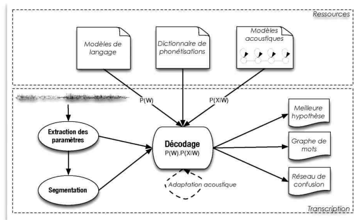
FIGURE 1.5 – Vue d'ensemble d'un système de RAP probabiliste
