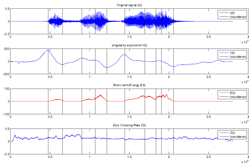
FIGURE 5.3 – HAUT - Signal original s(t) et sa transcription manuelle avec les frontières, MILIEU-1 en bleu, courbe des changements de niveaux des EdS h(t) , MILIEU-2 en rouge, variation temporelle de l'énergie à court-terme E(t) , BAS - variation temporelle du taux de passage par zéro Z(t) .
