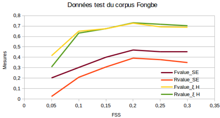
FIGURE 5.7 – Courbes de Fvalue et Rvalue de chaque méthode
