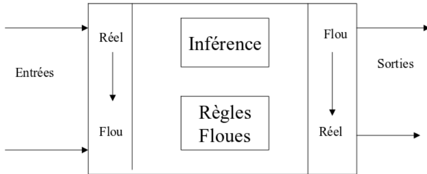
FIGURE 4.3 – Architecture d'un système de logique floue
