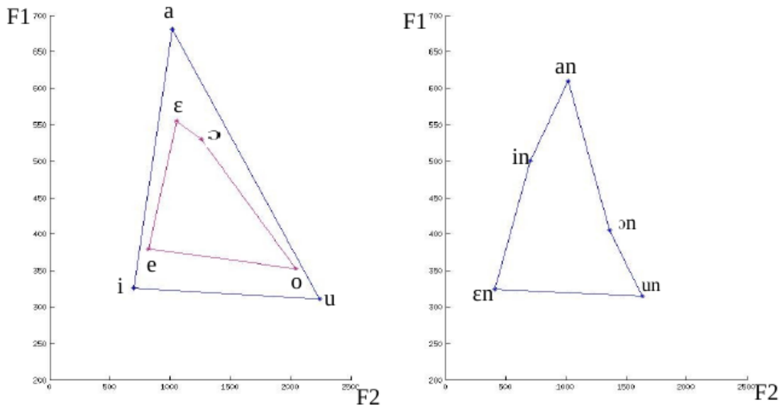
FIGURE 3.1 – Triangle vocalique sur le plan F1-F2, Gauche - Les voyelles orales, Droite - Les voyelles nasales
