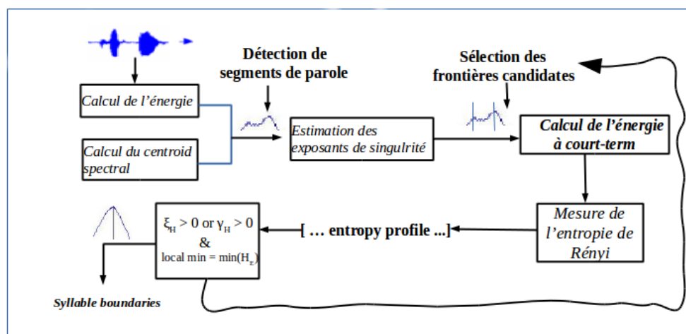
FIGURE 5.1 – Vue d’ensemble des étapes de l’approche proposée
