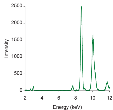
(d) X-Fluorescence of SCoMPI
