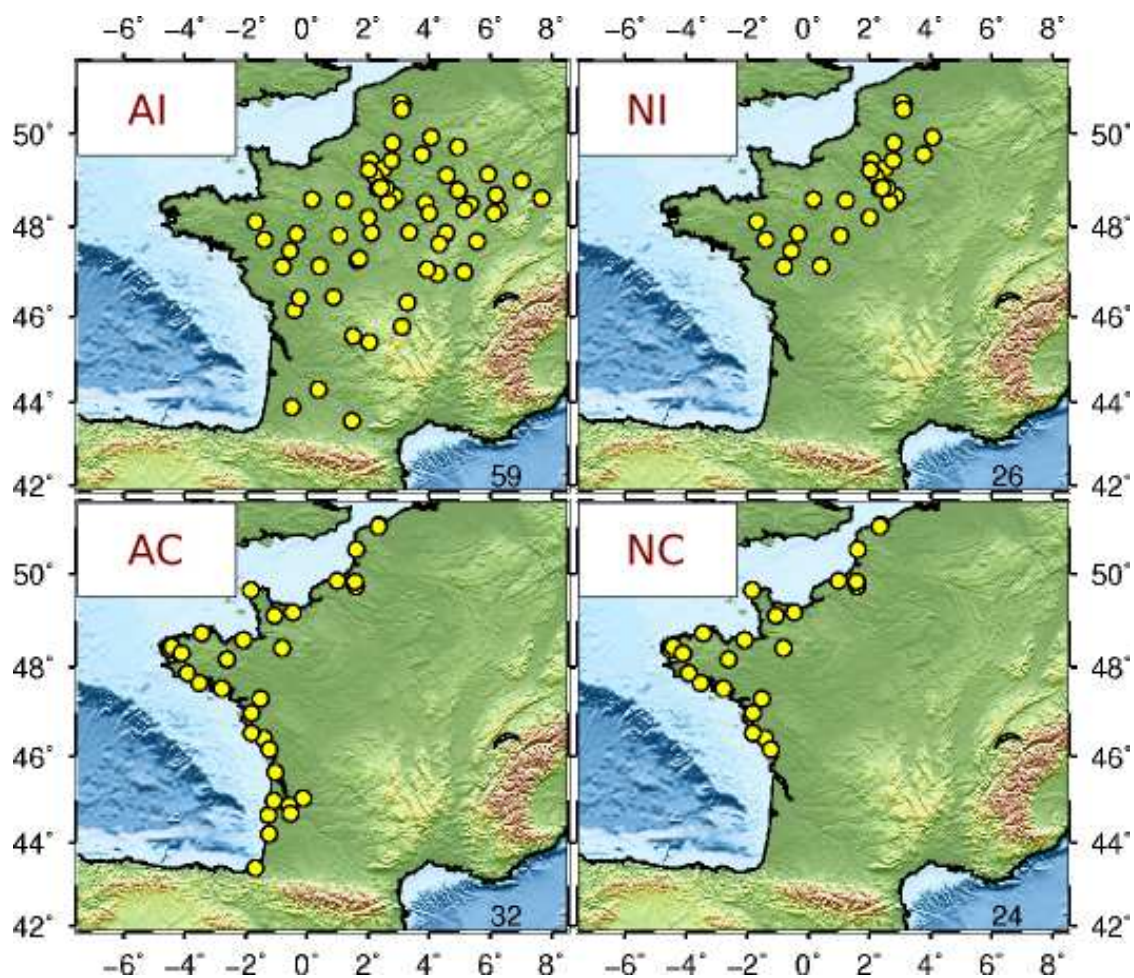
Figure 8 – Sélection des stations: Continental étendu (AI pour all inland), continental proche (NI pour nearby inland), côtier étendu (AC pour all coastal) et côtier proche (NC pour nearby coastal), les stations étant considérées proches lorsqu'elles sont situées à moins de 200 km de la trace de la tempête. Les nombres dans les coins gauche indiquent le nombre de stations.
