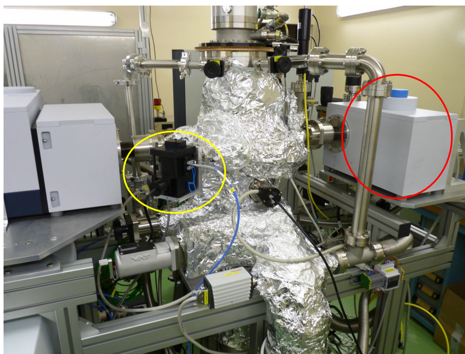
Figure 5.3.2 : Photographie montrant l'arrière d'IGLIAS par rapport à la figure 5.1.2. Jaune : sphère intégrant le spectromètre visible-ultraviolet. Rouge : détecteur MCT du spectromètre infrarouge.
