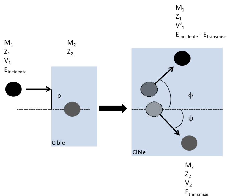
Figure A.1.1 : Schéma représentant une collision élastique entre un ion de masse M_1 , de numéro atomique Z_1 , de vitesse V_1 , d'énergie cinétique E_{incidente} et de paramètre d'impact p et un atome-cible de masse M_2 , de numéro atomique Z_2 au repos dans le référentiel du laboratoire. Après l'interaction, l'atome-cible est dévié d'un angle \psi avec une énergie cinétique E_{transmise} . L'ion est dévié d'un angle \phi avec une énergie cinétique diminuée de E_{transmise} .
