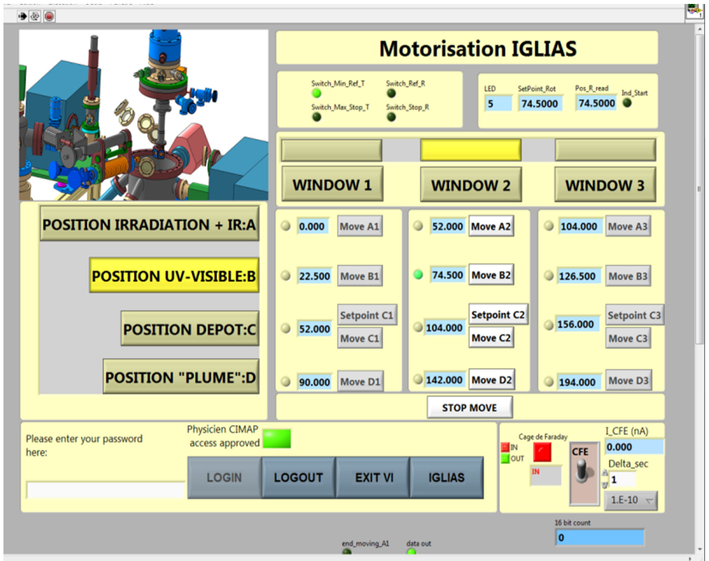
Figure 5.2.5 : Interface LabVIEW du pilotage d'IGLIAS depuis laquelle tous les déplacements motorisés s'effectuent manuellement. L'image montre que la tête rotative est en position B_2 correspondant à un angle de 74,5^\circ par rapport à l'origine A_1 , c'est-à-dire que la seconde fenêtre est placée en face de l'entrée du faisceau du spectromètre visible-ultraviolet.
