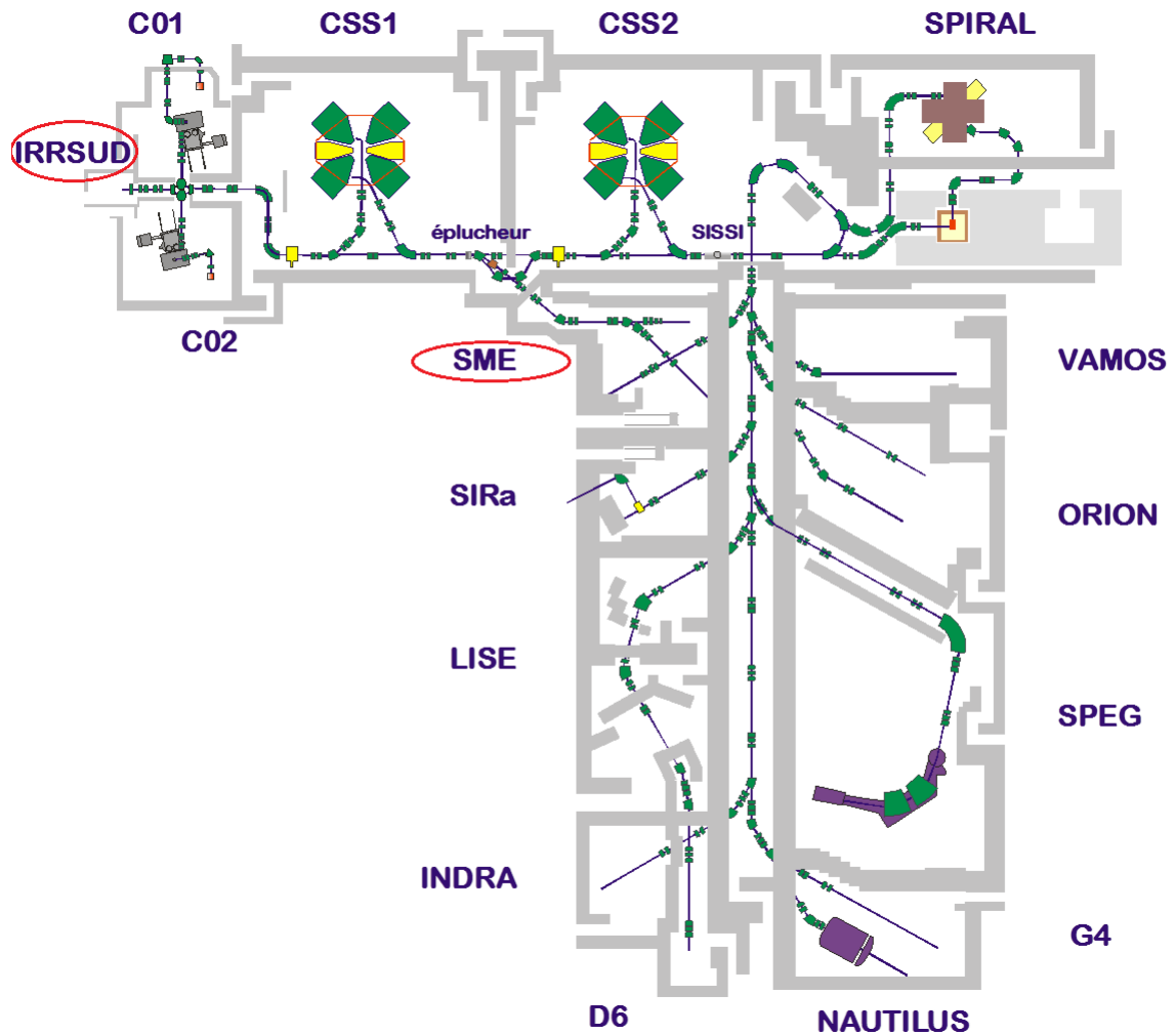
Figure 3.1.5 : Plan du GANIL comprenant notamment les sources couplées aux cyclotrons C01 et C02, la ligne à basse énergie IRRSUD, les cyclotrons à secteurs séparés CSS1 et CSS2 ainsi que la sortie à moyenne énergie SME. Les autres installations visibles sont essentiellement exploitées pour la physique nucléaire.
