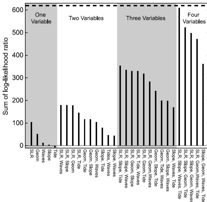
FIGURE 6.2 – Somme des ratios de log-vraisemblance obtenus pour des réseaux bayésiens intégrant différents sous-ensembles de variables explicatives de l'évolution du trait de côte de la côte est des Etats-Unis. Plus la valeur est élevée, plus la connaissance des variables précisée en-dessous de chaque barre permet d'améliorer les prédictions d'évolution du trait de côte du réseau Bayésien. Ce graphique montre que pour la côte est des Etats-Unis, l'élévation du niveau de la mer est la variable la plus importante. Source : Gutierrez et al. (2011).
