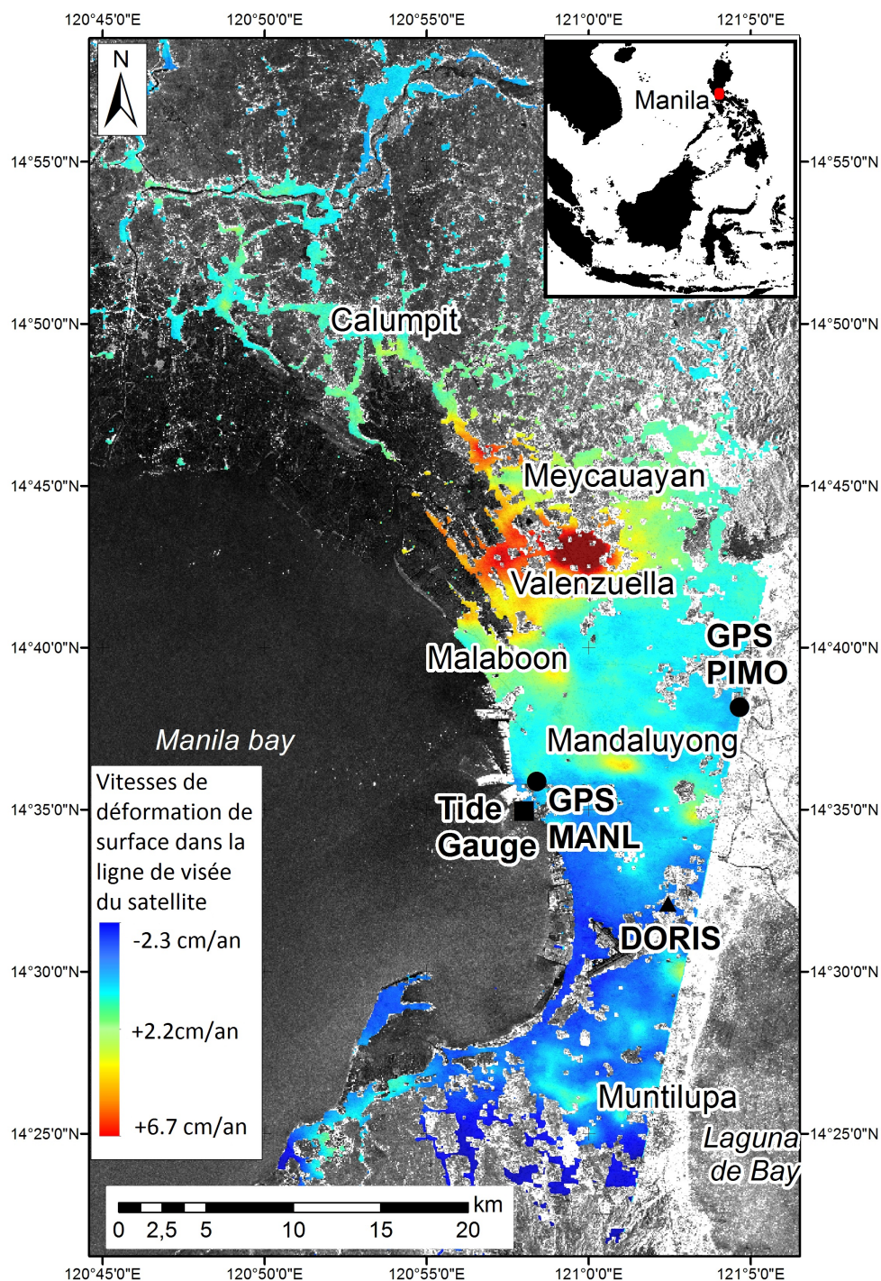
FIGURE 3.4 – Vitesse des déformations de surface dans la ligne de visée du satellite à Manille (Philippines), pour la période 1993-1998. Les valeurs négatives correspondent à des déplacements en direction du capteur, c'est à dire à des surrections. Données : ERS 1/2 (ESA) ; Traitements réalisés sous GAMMA par Daniel Raucoules ; Figure réalisée sous ArcGIS. D'après : Raucoules et al., 2013b.
