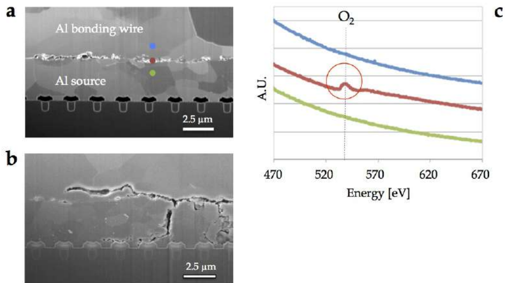
Figure 149: (a) Spectres EELS enregistrés à trois endroits, relatives aux points colorés en (a), proche de l'interface fil/métallisation dans un composé non vieilli. Le pic correspondant à l'oxygène ne ressort qu'à l'interface et prouve donc la présence d'oxyde localisé. (b) Pendant vieillissement, ces imperfections favorise la propagation de fissures le long de l'interface fil/métallisation, qui détermine un détachement local de deux métal. À cette endroit, des fissures verticales along the joints de grains peuvent aussi se propager jusqu'au substrat de Si, comme dans les portions de métallisation nues.
