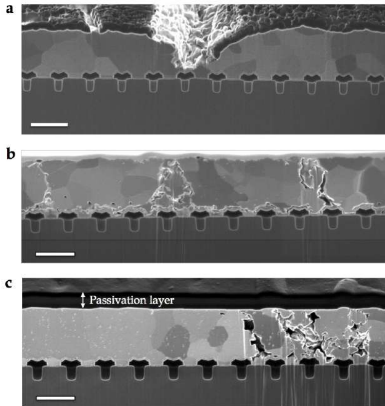
Figure 147: Fissuration de la métallisation développée dans une zone (a) non passivée, (b) passivée par mold compound et (c) passivé par \text{SiO}_2 (plus mold compound). Barre d'échelle: 2.5\mu\text{m} .
