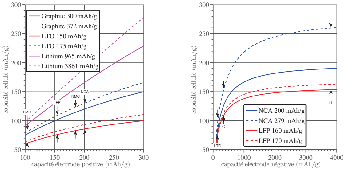
(a) Variation en fonction de la capacitè spécifique de la positive pour plusieurs électrodes négatives. Traits continus : capacitès réelles, traits tiretés : capacitès théoriques (maximum atteignable) (b) Variation en fonction de la capacitè spécifique de la négative pour plusieurs électrodes positives. Traits continus : capacitès réelles, traits tiretés : capacitès théoriques (maximum atteignable)
