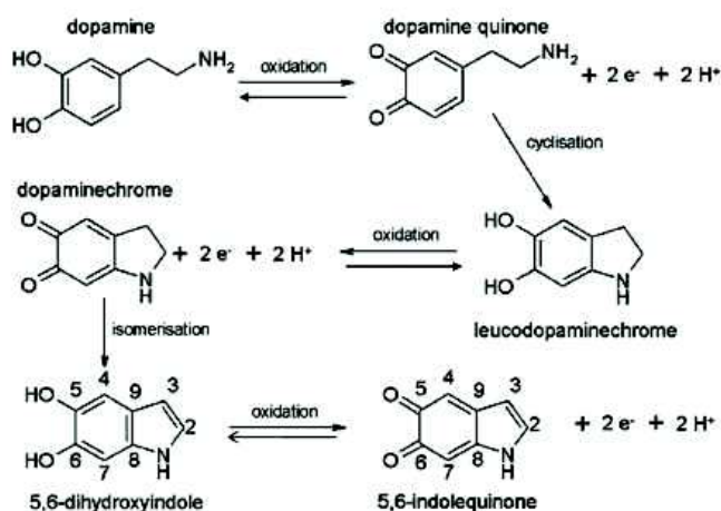
Figure 41 : Mécanisme de formation du 5,6-dihydroxyindole.
