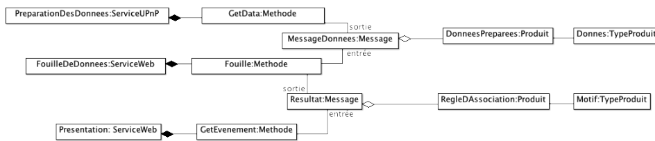
FIGURE 3.14 – Exemple de modèle d'orchestration
