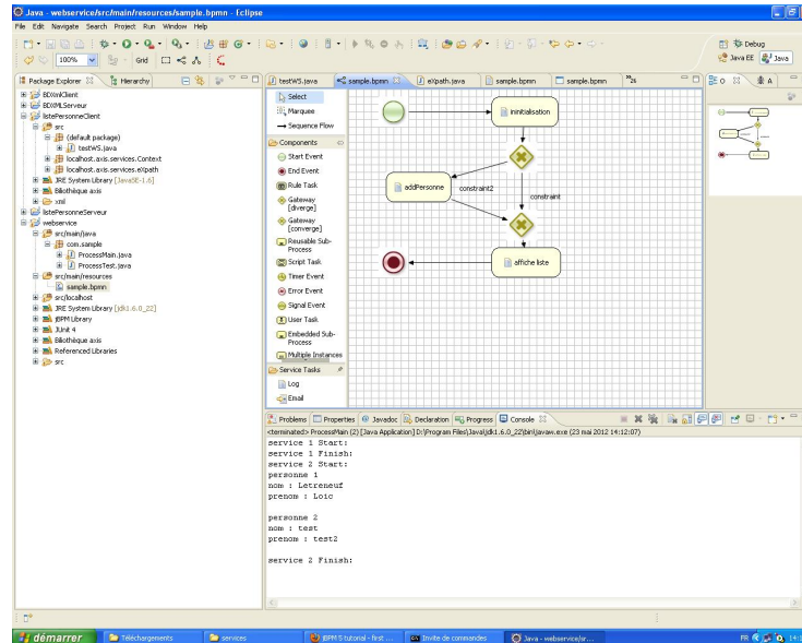
FIGURE 2.9 – Exemple de procédé WS-BPEL
