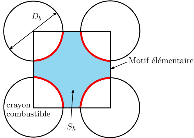
FIGURE 2.9 – Maille élémentaire d'écoulement de fluide.
