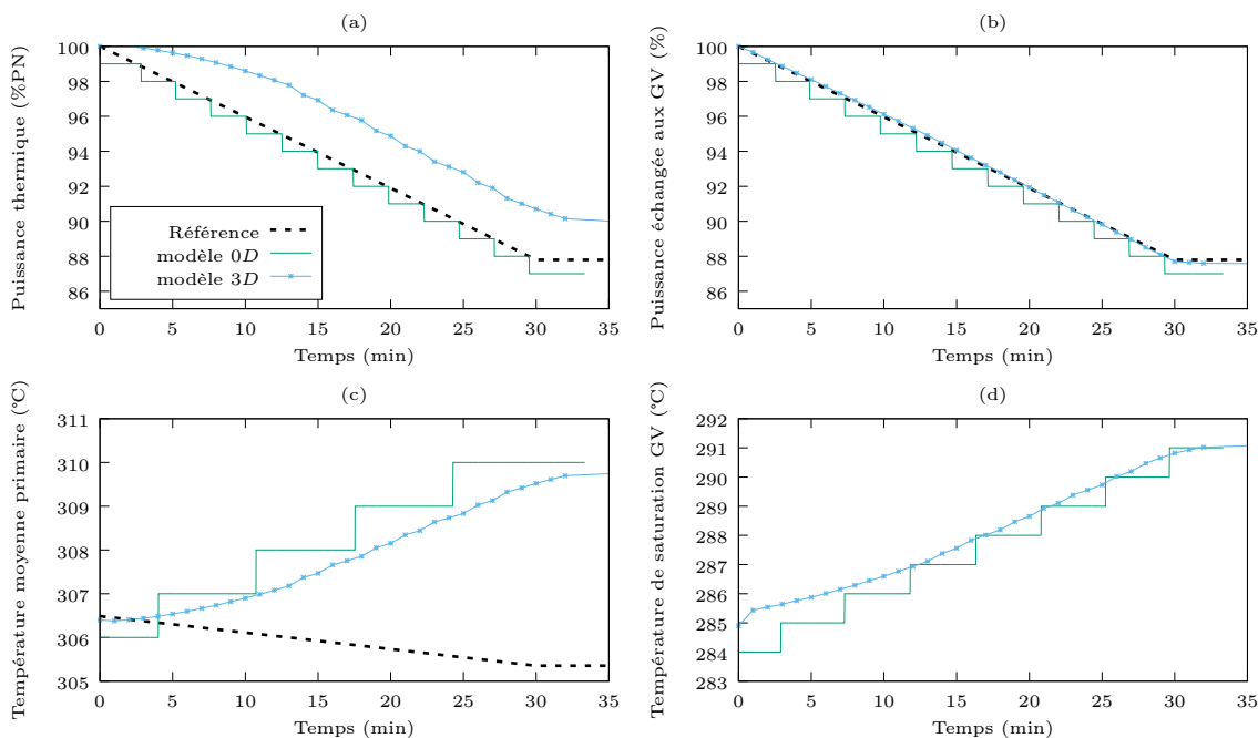
FIGURE 3.13 – Comparaison de grandeurs caract ristiques du c ur et du GV lors d'une rampe en dynamique libre, avec les diff rents mod les.
