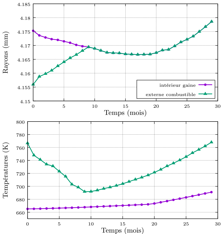
FIGURE B.2 – Evolution des rayons interne gaine et externe combustible ainsi que des températures correspondantes lors d'un fonctionnement en base à puissance nominale pour la tranche axiale la plus sollicitée du crayon subissant la plus importante puissance linéique moyenne.
