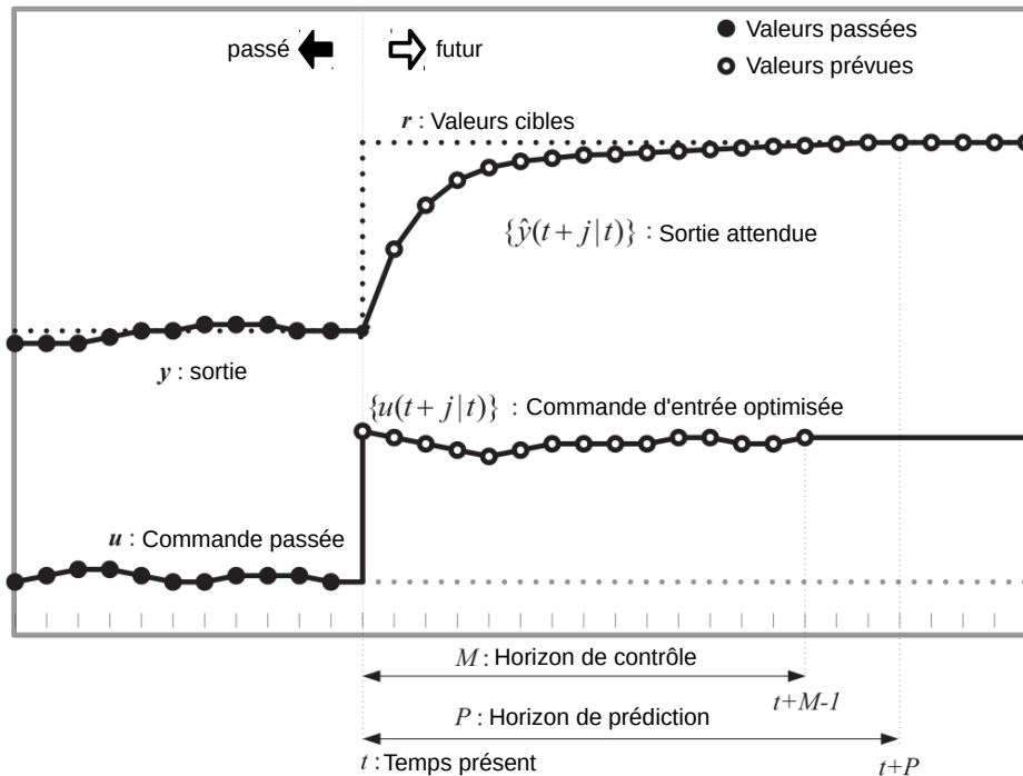
FIGURE 4.3 – Illustration, pour un pas de temps donné, des horizons de contrôle et de prédiction, et de la prévision de la sortie attendue en fonction de la commande d'entrée [62].
