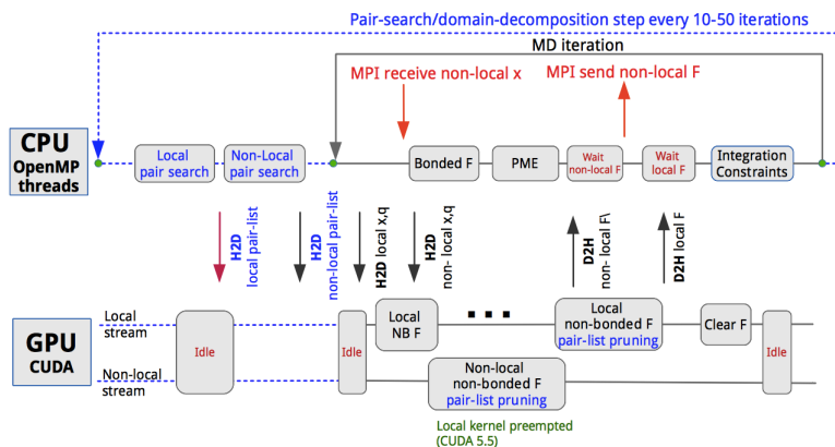
FIGURE 3.8 – Pipeline d’une itération avec support GPU. Les données sont d’abord transférées sur le GPU avant le calcul des forces non liées sur le GPU. 9
