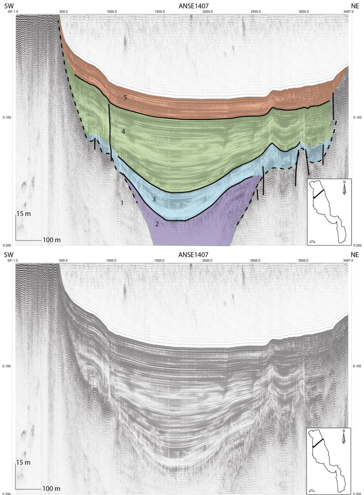
Figure III-50 : Profil sismique transversal de très haute résolution (SEISTEC™ Boomer). La localisation est marquée dans l'encart, les échelles horizontales et verticales sont également présentes sur la gauche du profil. Ce profil présente toutes les unités du lac d'Annecy ainsi que des ruptures dans le substratum, l'unité 2 et l'unité 4.
