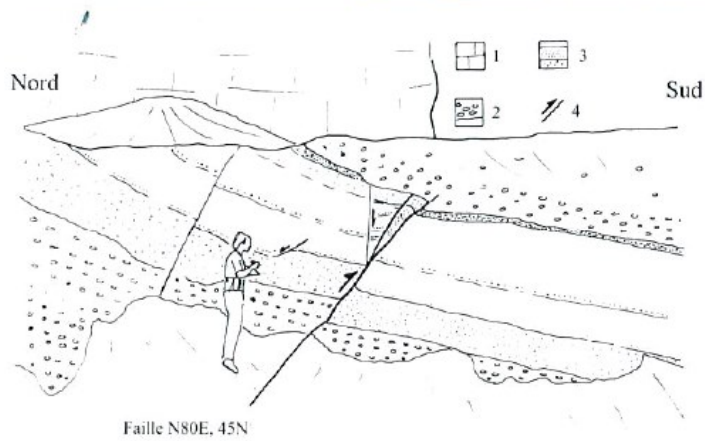
Figure I-10 : Coupe près du contact faillé entre les séries quaternaires et les calcaires crétaçés ; 1 : calcaire crétaçé ; 2 : moraines « würmiennes » ; 3 : sables (fluvio-lacustres ?) ; 4 : failles (Baize et al., 2002).
