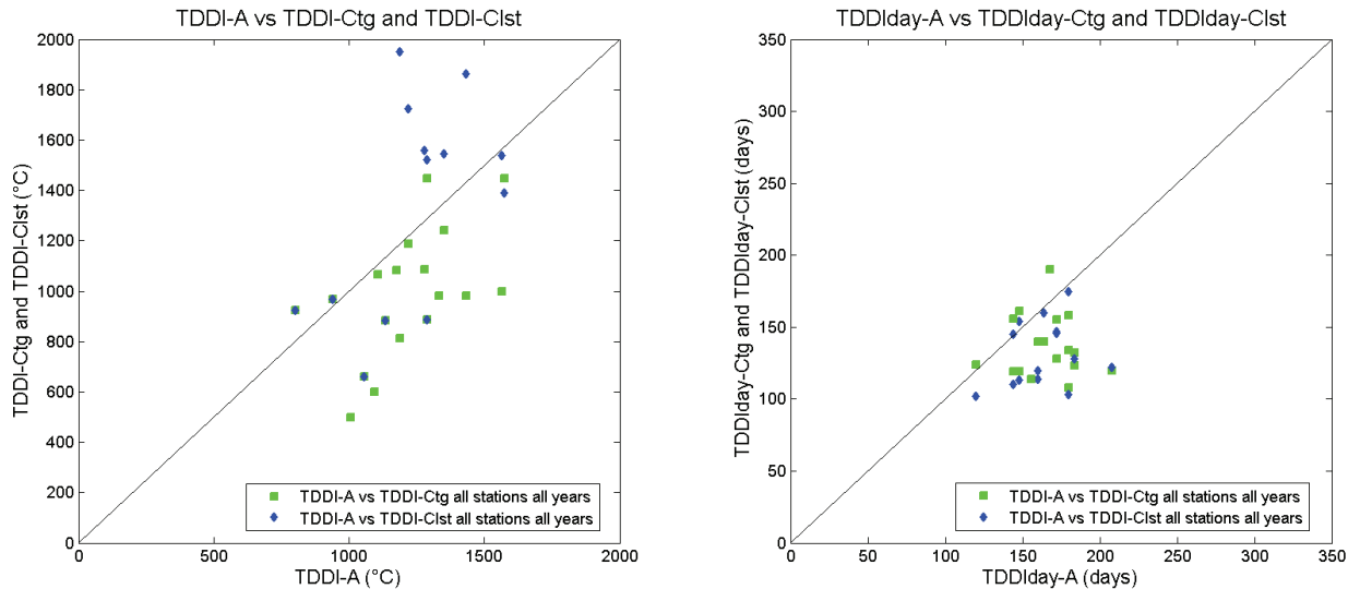
FIGURE 6.3 – La figure de gauche représente la comparaison des TDDI-A (André et al., 2015) et des TDDI-C_{tg} et des TDDI-C_{lst} . La figure de droite représente, pour les mêmes variables, une comparaison des nombres de jours de fonte et de gel. Ces résultats regroupent l'ensemble des stations pour toutes les années disponibles et permettent de rendre compte du bon accord des différentes données.
