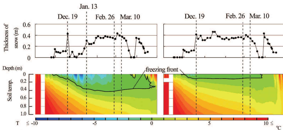
FIGURE 5.3 – Comparaison de la profondeur de pénétration du froid au cours de l’hiver. A gauche un terrain où la neige a été retirée après chaque chute de neige entre le 19 Décembre et le 13 Janvier, soit le temps que le gel atteigne une profondeur de 40 cm, puis que l’épaisseur de neige du site test a été remise à équivalence de l’épaisseur de neige du site témoin. A droite l’expérience témoin non perturbée. Les températures sont indiquées en degrés Celsius, et les profondeurs en mètres (Iwata et al., 2010).
