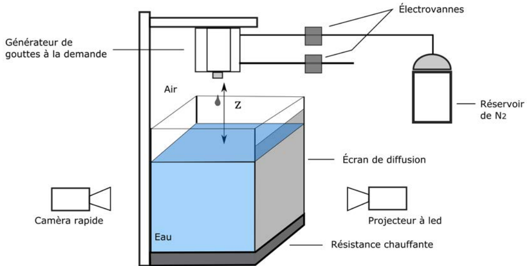
FIGURE 2.12 – Dispositif expérimentale.
