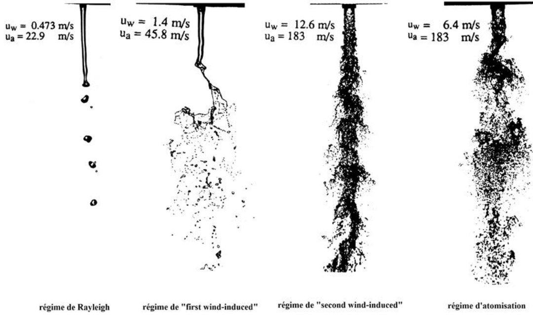
FIGURE 1.2 – Les quatre régimes de fragmentation typiques pour un jet coaxial eau-air ( u_w est la vitesse du jet eau, u_a la vitesse du courant d'air), Chigier et Farago [1992].
