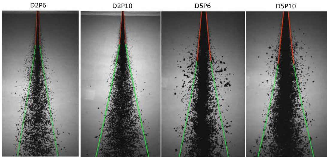
FIGURE 3.5 – Images typiques du jet en régime permanent en fonction de la pression d’injection et du diamètre de la buse. La première partie du jet en rouge ( \theta_1 ), la seconde partie du jet en vert ( \theta_2 ). D2P6 : [D=2mm, P=6bar, \theta_1=5^\circ , \theta_2=18^\circ ]; D2P10 : [D=2mm P=10bar, \theta_1=7.5^\circ , \theta_2=24^\circ ]; D5P6 : [D=5mm, P=6bar, \theta_1=10^\circ , \theta_2=21^\circ ]; D5P10 : [D=5mm, P=10bar, \theta_1=12.5^\circ , \theta_2=25^\circ ].
