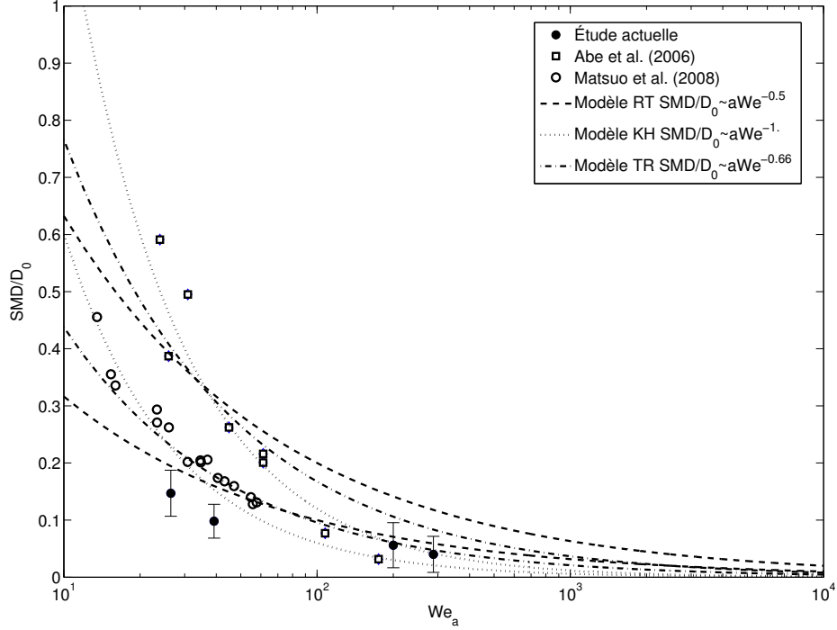
FIGURE 3.20 – Diamètre de Sauter en fonction du nombre de We . Une courbe de tendance SMD/D_0 = aWe^{-0.67} est déterminée par la méthode des moindres carrés. Modèle RT : représente le modèle de Rayleigh-Taylor ( SMD/D_0 \simeq aWe^{-0.5} avec a = 1 et a = 2 ), Modèle KH : représente le modèle de Kelvin-Helmholtz ( SMD/D_0 \simeq aWe^{-1} avec a = 6 et a = 12 ) et Modèle TR : représente le modèle turbulent suggéré par Rimbert et Castanet [2011] ( SMD/D_0 \simeq aWe^{-0.66} avec a = 2 et a = 3.5 ). Le détail du calcul d'erreurs est donné dans la section B.2.
