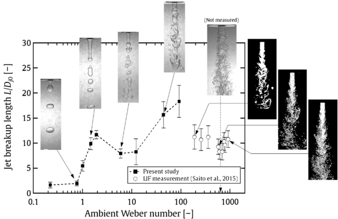
FIGURE 1.8 – Longueur de rupture de jet en fonction du nombre de Weber ambiant. Les cercles ouverts \circ représentent les données obtenues via LIF planaire (Fluorescence Induite par Laser) en utilisant la technique d'indexation, Saito et al. [2017]. Les trois images à droite sont obtenues par la méthode LIF planaire.
