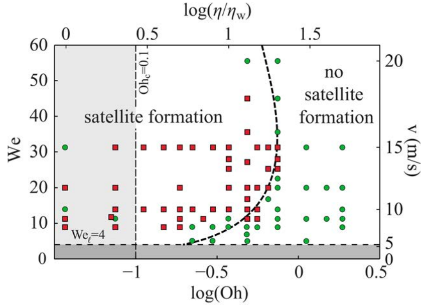
FIGURE 1.7 – Diagramme de la formation des gouttes satellitaires pour différentes vitesses et valeurs de viscosité du liquide. Carré : les cas où le calcul prédit la production des gouttes satellitaires, Cercle : cas sans production de gouttes satellitaires. Le rayon, ainsi que la tension de surface et la densité sont constants, fixés respectivement à D_0 = 20\mu m , \rho_L = 1000kg/m^3 , et \sigma = 72mN/m .
