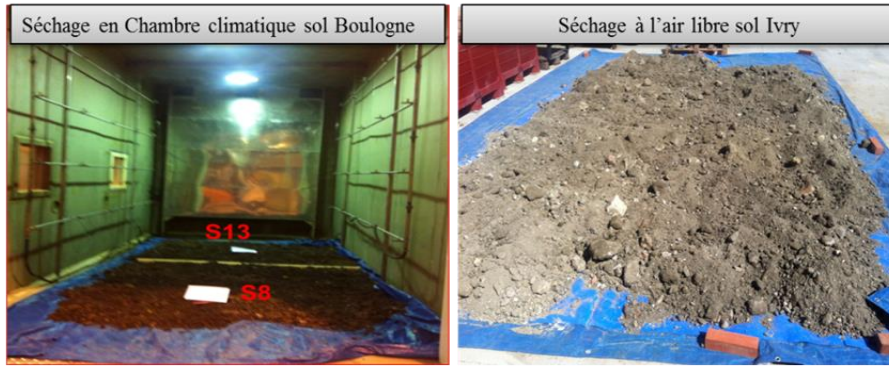
Figure 30: Séchage des matériaux étudiés
