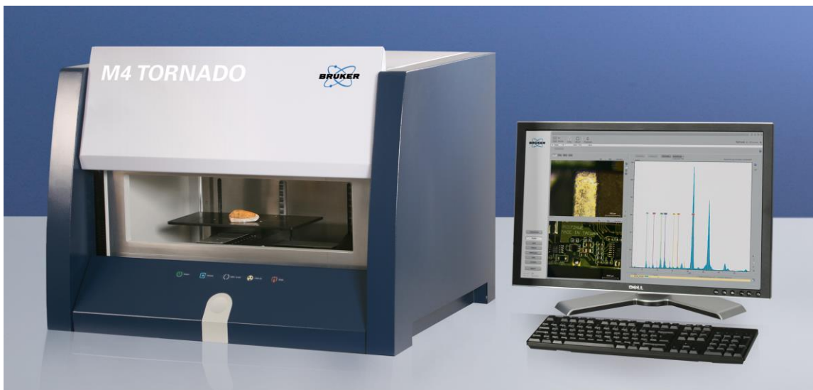
Figure 48: Spectromètre de fluorescence X de type Tornado M4
