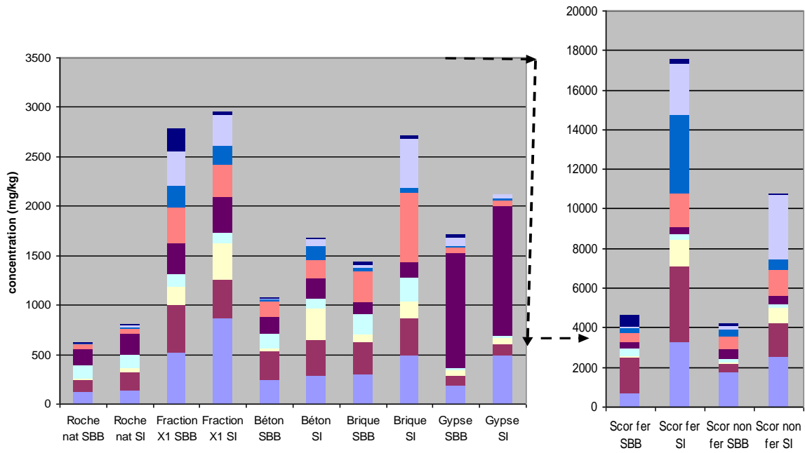
Figure 81: Répartition des éléments intermédiaires dans les composants issus de l'essai de tri
