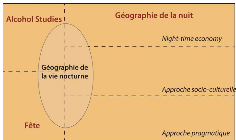
Figure 2 : Schéma récapitulatif situant l'objet de la recherche M. Bonte, 2017
