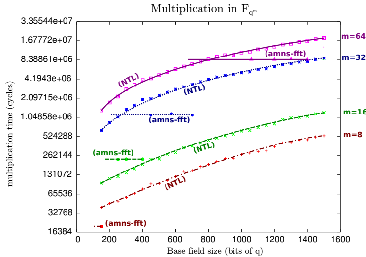
FIGURE II.1 – Résultat de notre implémentation AMNS.
