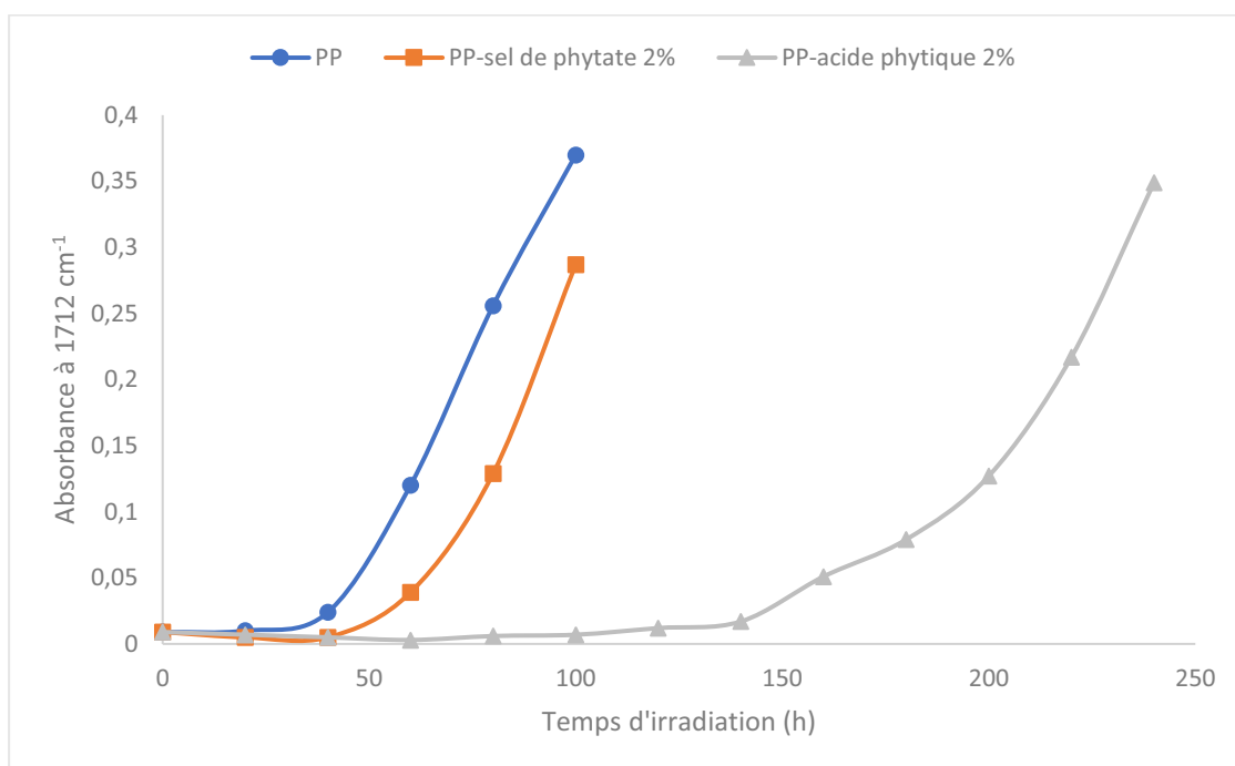
Figure 102 : Comparaison des absorbances à 1712\text{ cm}^{-1} en fonction du temps d'irradiation en SEPAP 12/24 à 60^\circ\text{C} , du PP seul, PP-stabilisé avec du sel de phytate à 2%, PP stabilisé avec de l'acide phytique à 2%
