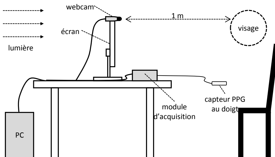
FIGURE 3.37 – Configuration expérimentale.
