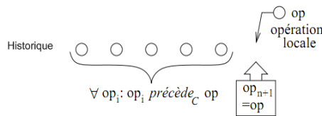
FIGURE 2.8 – Exécution d'une opération locale
