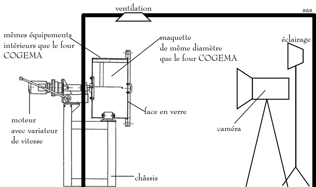
Figure I- 3 : Schéma de l'installation (par exemple avec la maquette COGEMA).
