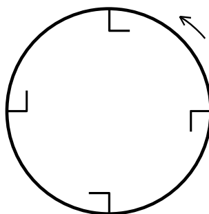
Figure IV- 27 : Montage actuel des releveurs dans le four FBFC numéro 7.
