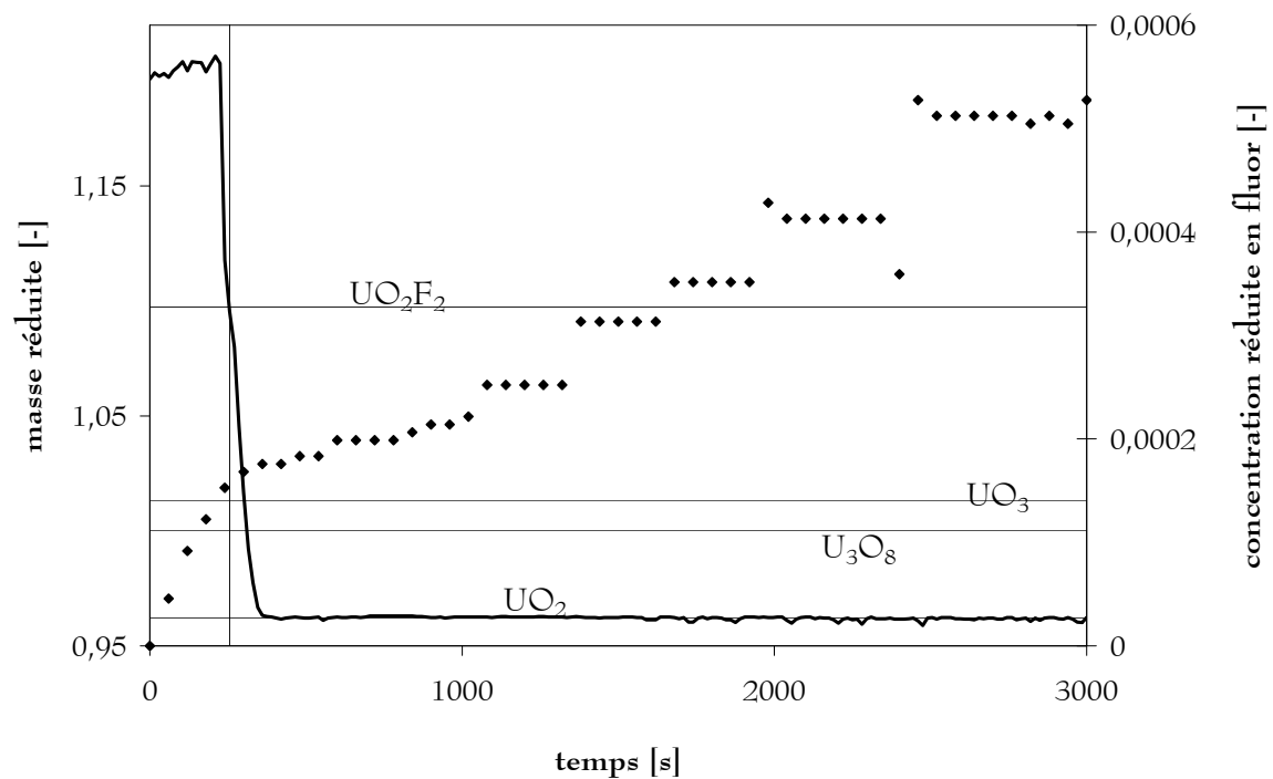
Figure II- 8 : Perte de masse et concentration en fluor. essai 12 – 45 % \text{H}_2\text{O} – 45 % \text{H}_2 – 700 °C
