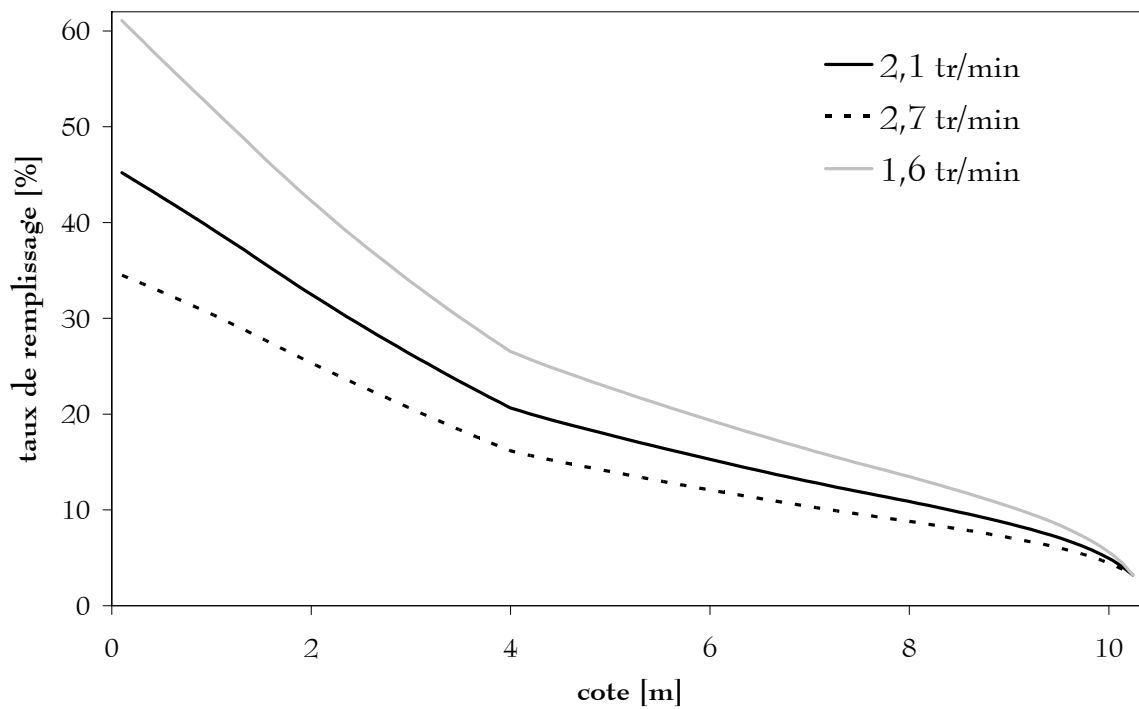
Figure I- 47 : Influence de la vitesse de rotation. (four COGEMA ; débit d'alimentation de 890 kg UF6 /h)
