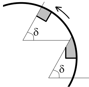
Figure I- 13 : Définition de l'angle d'avalanche.
