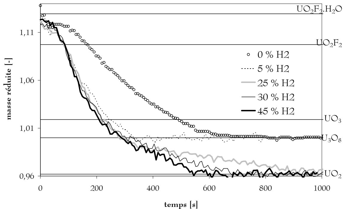
Figure II- 13 : Essais pour différentes teneurs en hydrogène, à 700 °C, sous 300 mbar d' \text{H}_2\text{O} .
