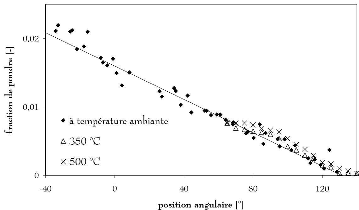
Figure I- 21 : Déchargement de \text{UO}_2\text{F}_2 .
