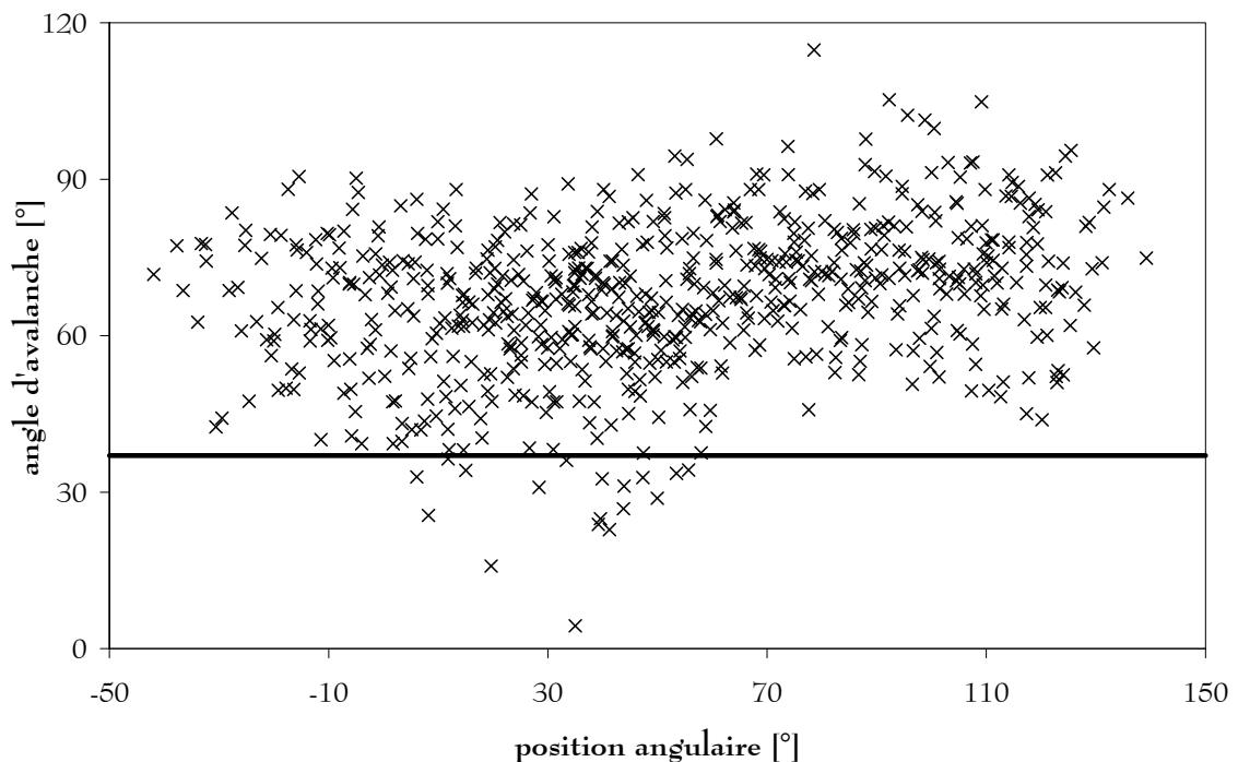
Figure I- 14 : Valeurs mesurées de l'angle d'avalanche. (le trait horizontal correspond à la moyenne des valeurs d'angle dynamique de repos)
