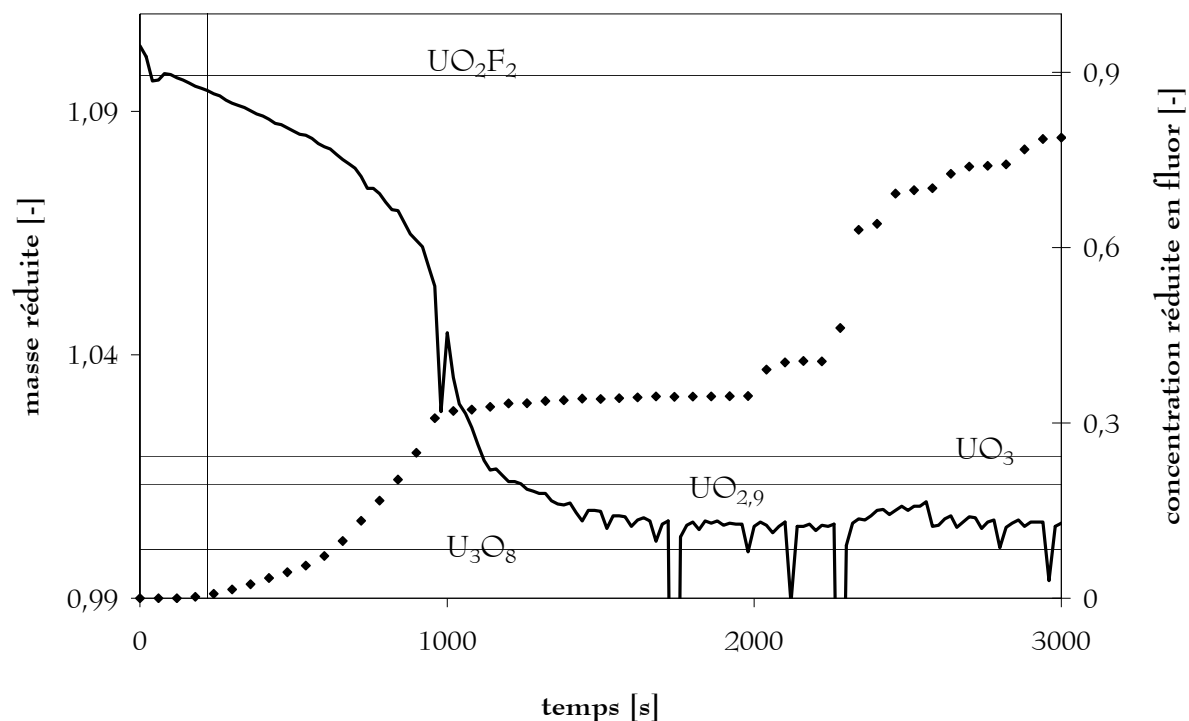
Figure II- 6 : Perte de masse et concentration en fluor.
