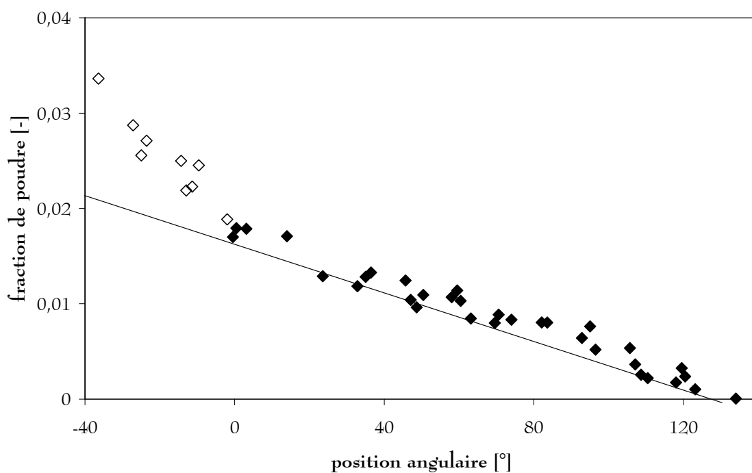
Figure I- 11 : Déchargement des relevurs à température ambiante, pour un taux de remplissage élevé.
