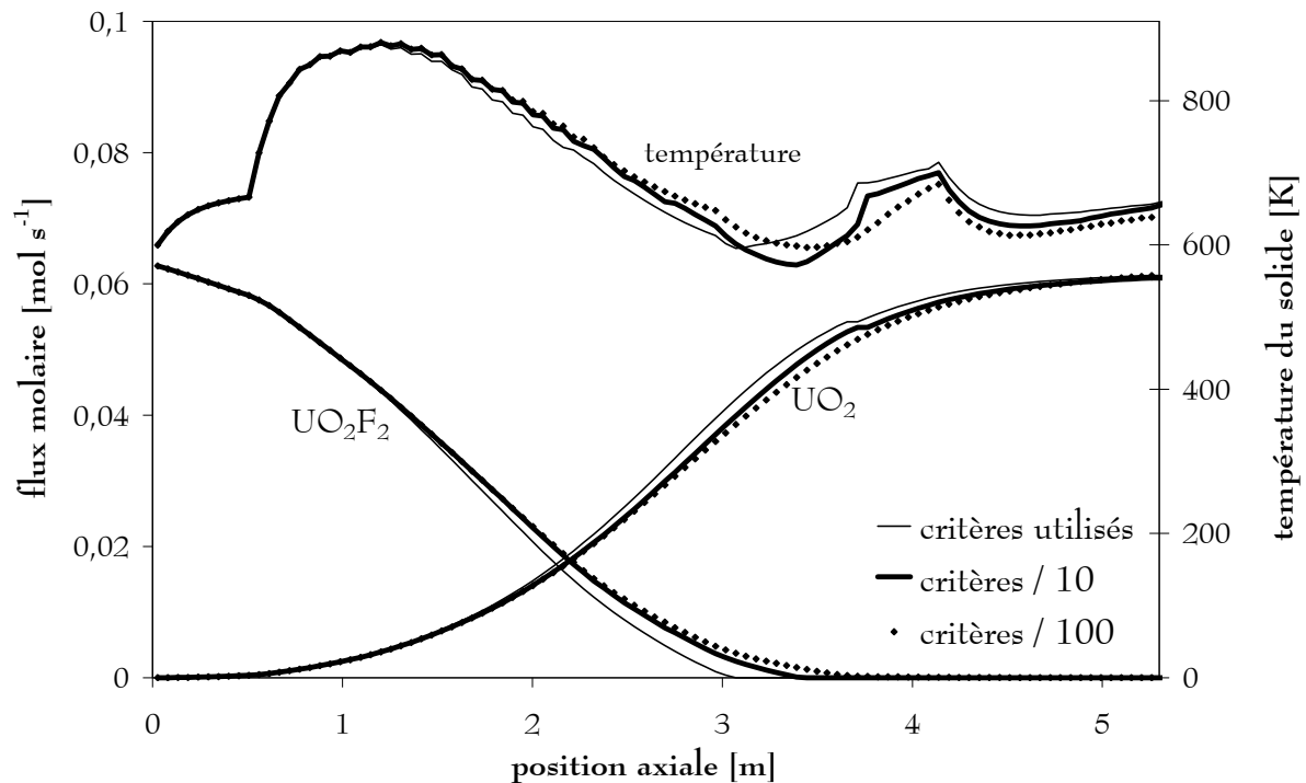
Figure IV- 24 : Influence des critères de convergence sur les flux molaires d' \text{UO}_2\text{F}_2 et d' \text{UO}_2 et sur les températures du solide. (four FBFC)
