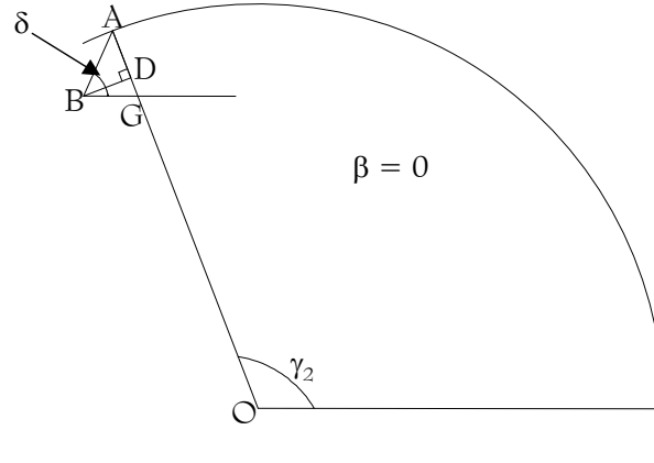
Figure I- 56 : Géométrie dans le cas \gamma = \gamma_2 .
