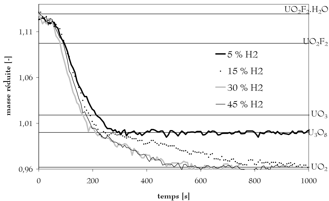
Figure II- 14 : Essais pour différentes teneurs en hydrogène, à 700 °C, sous 450 mbar d' \text{H}_2\text{O} .
