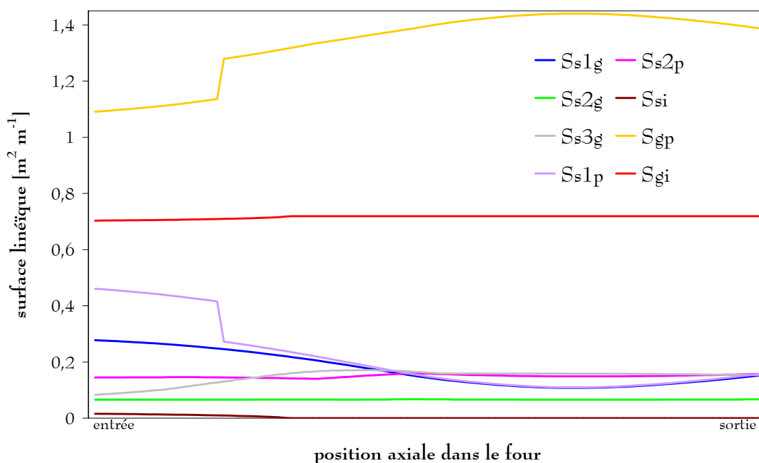
Figure III- 9 : Surfaces d'échange thermique dans un four FBFC.
