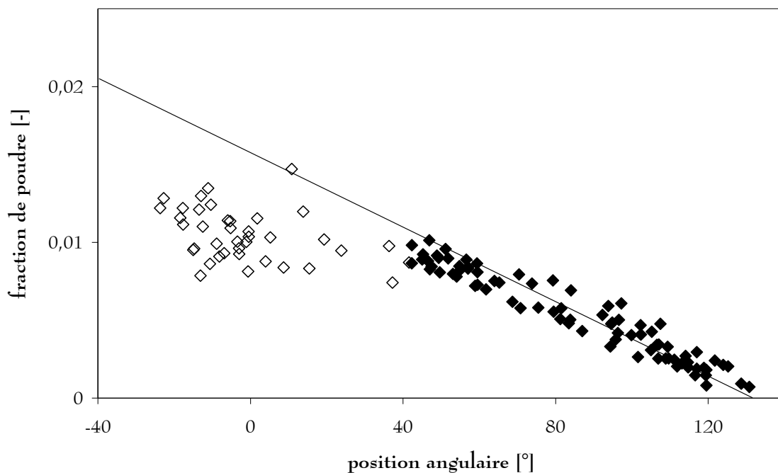
Figure I- 10 : Déchargement des relevurs à température ambiante, pour un faible taux de remplissage.
