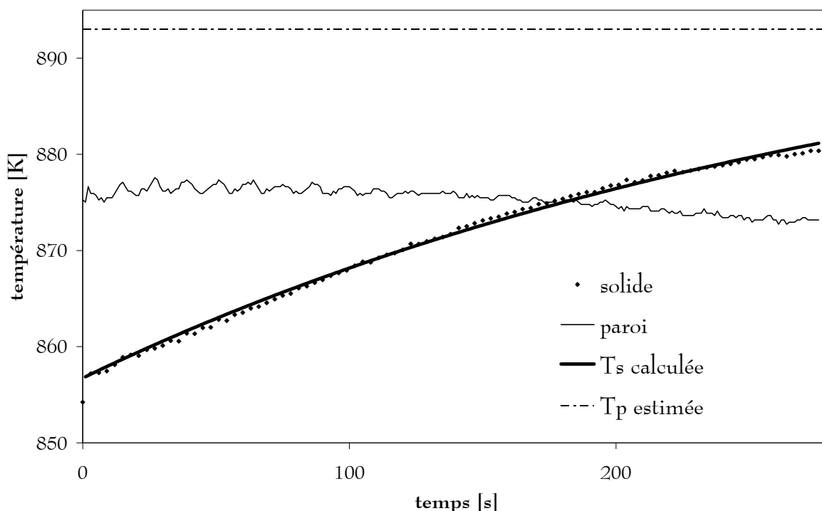
Figure III- 3 : Mesure du coefficient de transfert thermique solide / paroi : exemple de résultat avec le second protocole expérimental. (vitesse de rotation 2 tr/min, température de paroi 600 °C)
