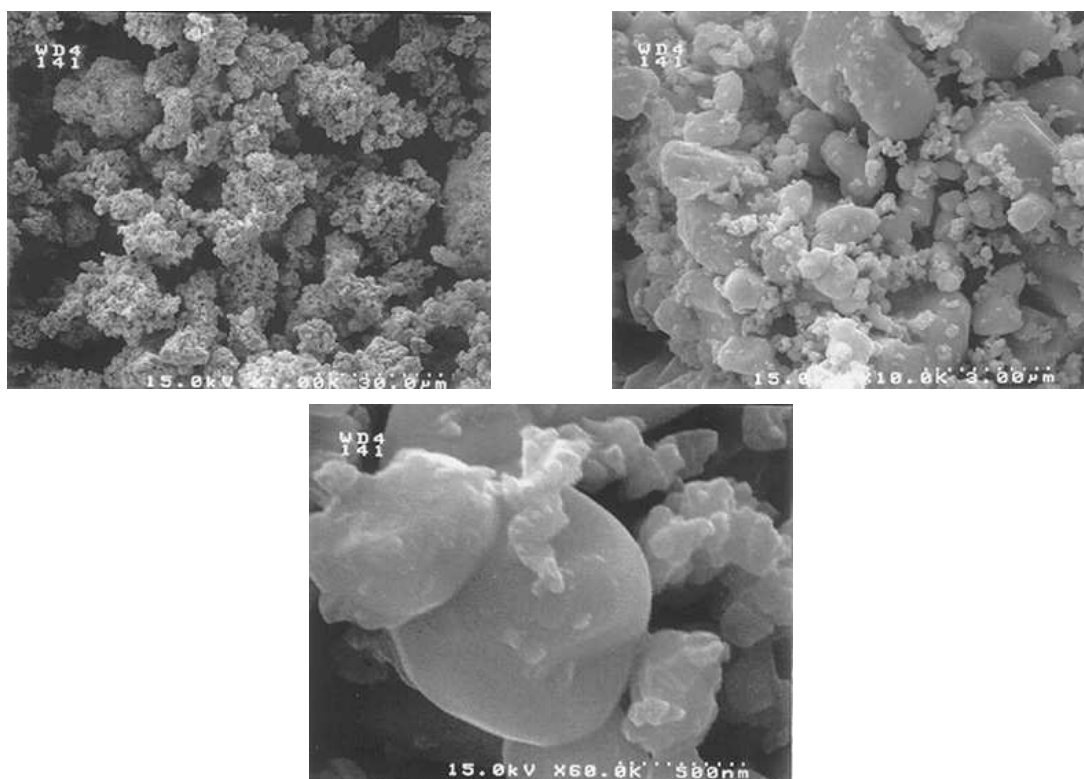
Figure 13 : Clichés MEB d'un échantillon d' \text{U}_3\text{O}_8 contenant 3,5 % d' \text{UO}_2\text{F}_2 . × 1000 ; × 10000 ; × 60000
