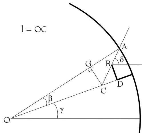
Figure I- 50 : Géométrie dans le cas \gamma_I \leq \gamma < \gamma_I .
