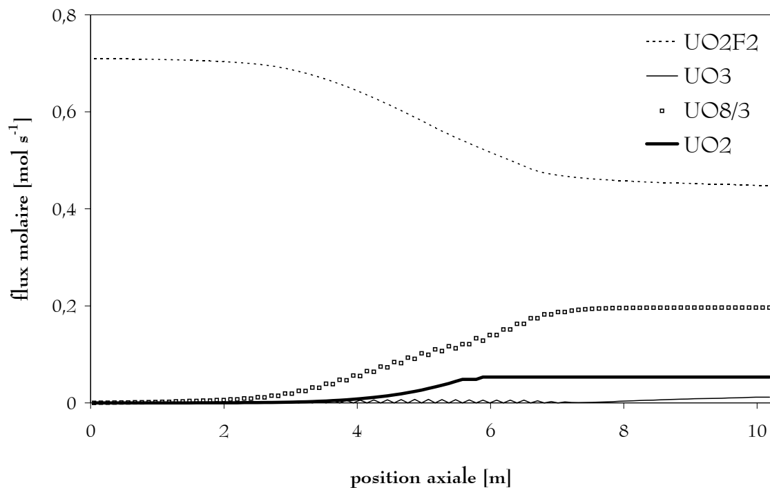
Figure IV- 6 : Profils de flux molaire des solides dans un four COGEMA. (premiers résultats)
