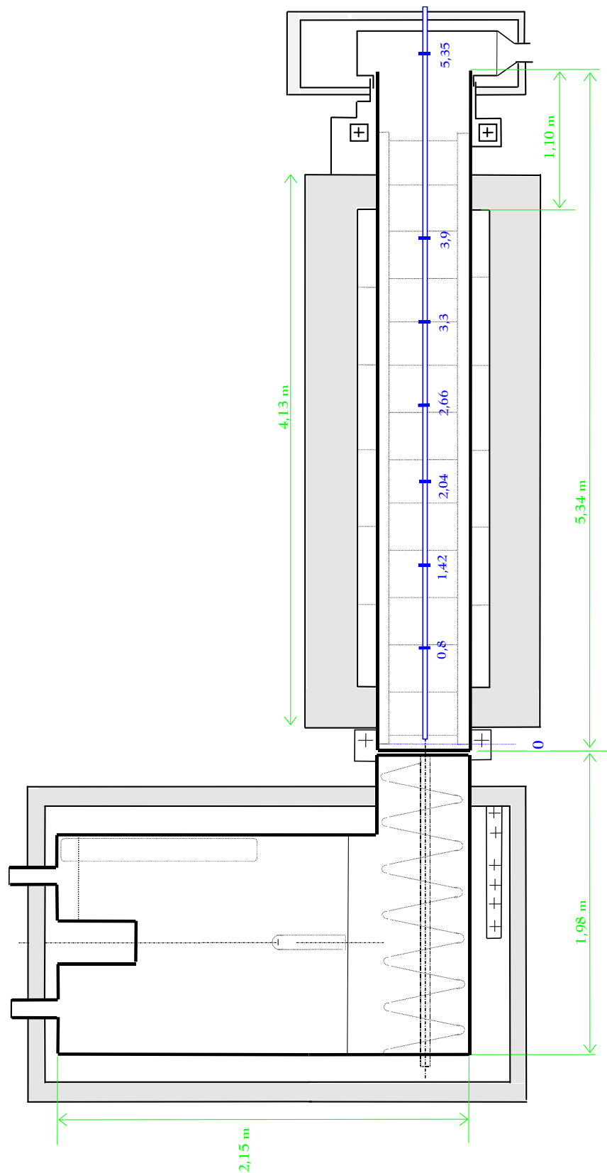
Figure 7 : Schéma coté d'un four FBFC.
