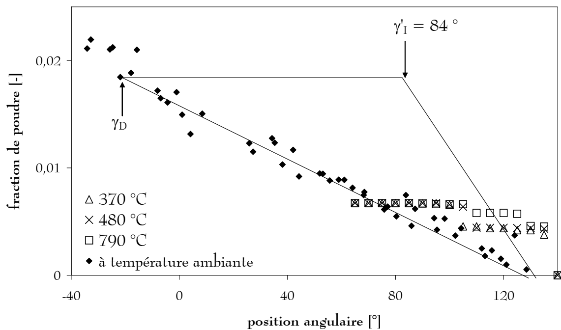
Figure I- 22 : Déchargement d'un oxyde d'uranium (exemple de \text{U}_3\text{O}_8 type COGEMA).
