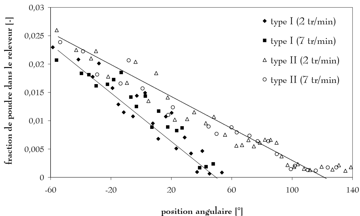
Figure I- 28 : Exemples de lois de déchargement de deux types de relevateurs.
