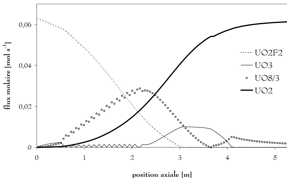
Figure IV- 19 : Profils de flux molaire des solides. (four FBFC)
