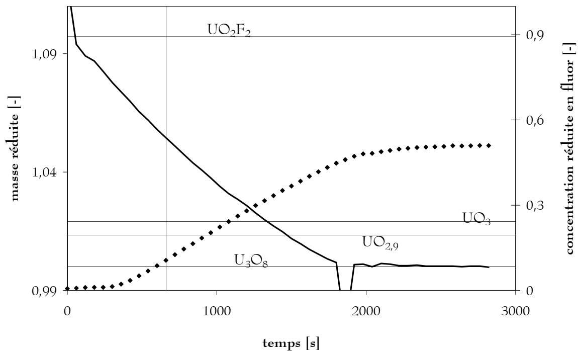
Figure II- 7 : Perte de masse et concentration en fluor. essai 8 bis – 30 % \text{H}_2\text{O} – 800 °C
