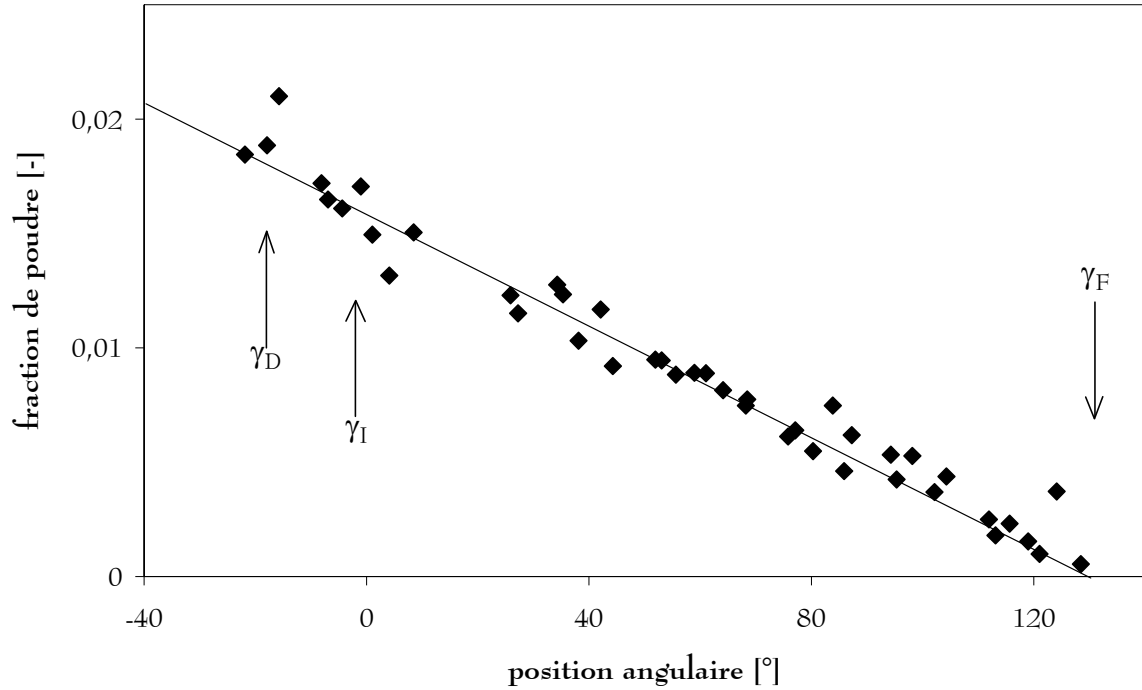
Figure I- 7 : Déchargement des releveurs à température ambiante.
