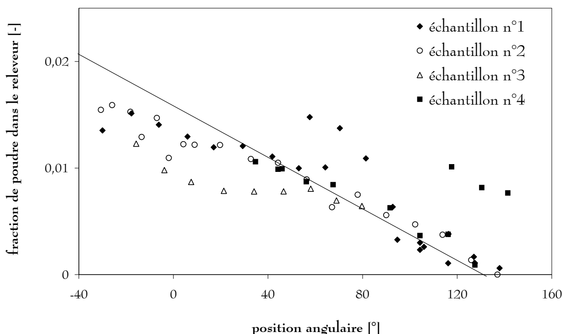
Figure I- 19 : Déchargement de U_3O_8 type COGEMA dans des relevateurs corrodés.
