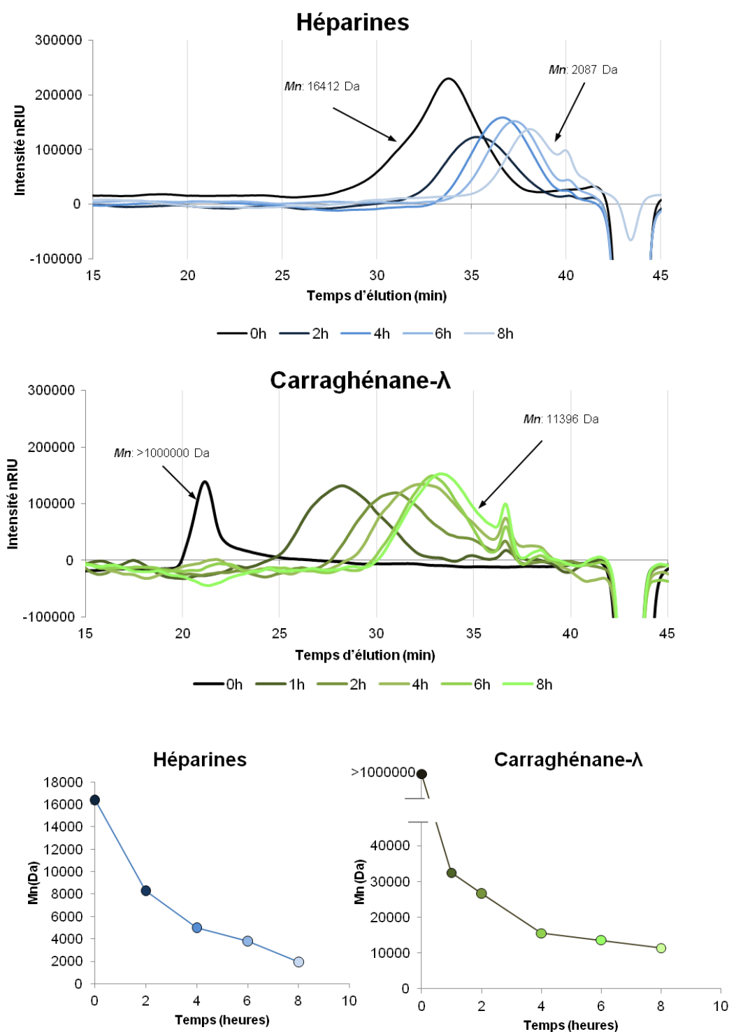
Figure 43 : Chromatogrammes SEC-HPLC des  chantillons d polym ris s par la m thode radicalaire assist es par ultrasons (DR) pour les temps de d polym risation entre 0 et 8h des h parines et carragh nanes- . Les masses molaires moyennes en nombre M_n sont indiqu es pour les temps 0 et 8h. Les M_n obtenus en fonction du temps de d polym risation sont  galement exprim s sous forme de graphiques. Les  chantillons ont  t  analys s   une concentration de 1g/L, s par s par une association de deux colonnes TSK-G5000PW et TSG-G4000PW   l'aide d'un  luant \text{NaNO}_3 0,1M et d tect s par r fractom trie diff rentielle.
