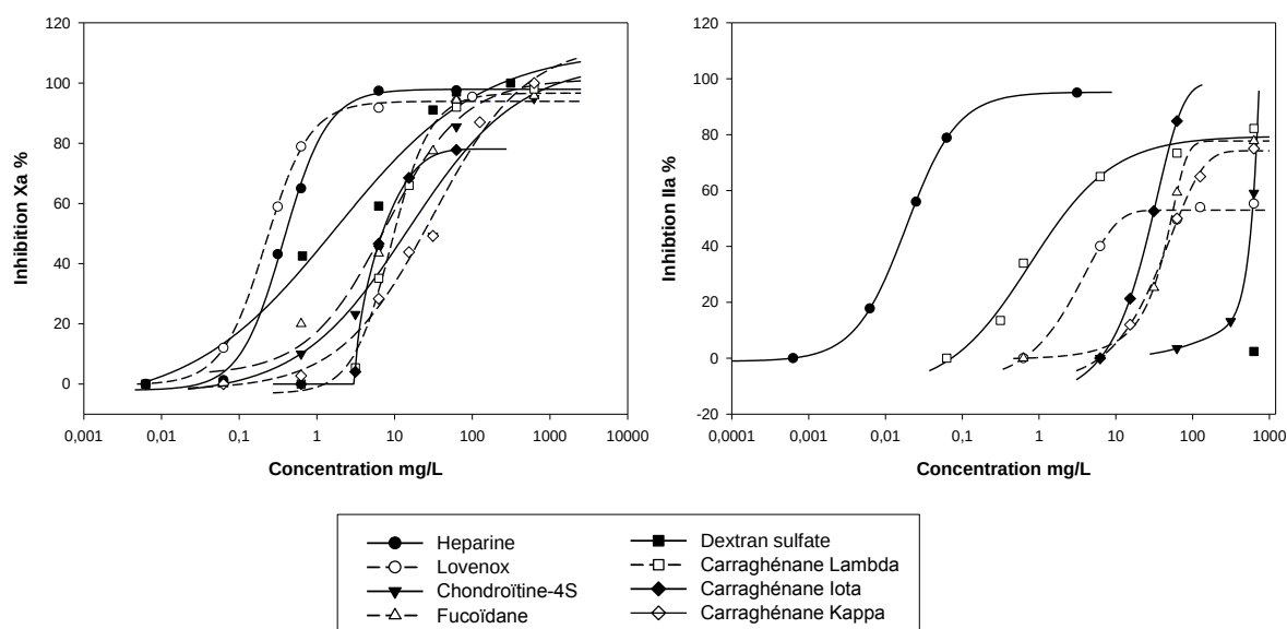
Figure 46 : Analyses dose/réponse des composés-NF pour l'inhibition des facteurs Xa et IIa de la coagulation en présence d'antithrombine.
