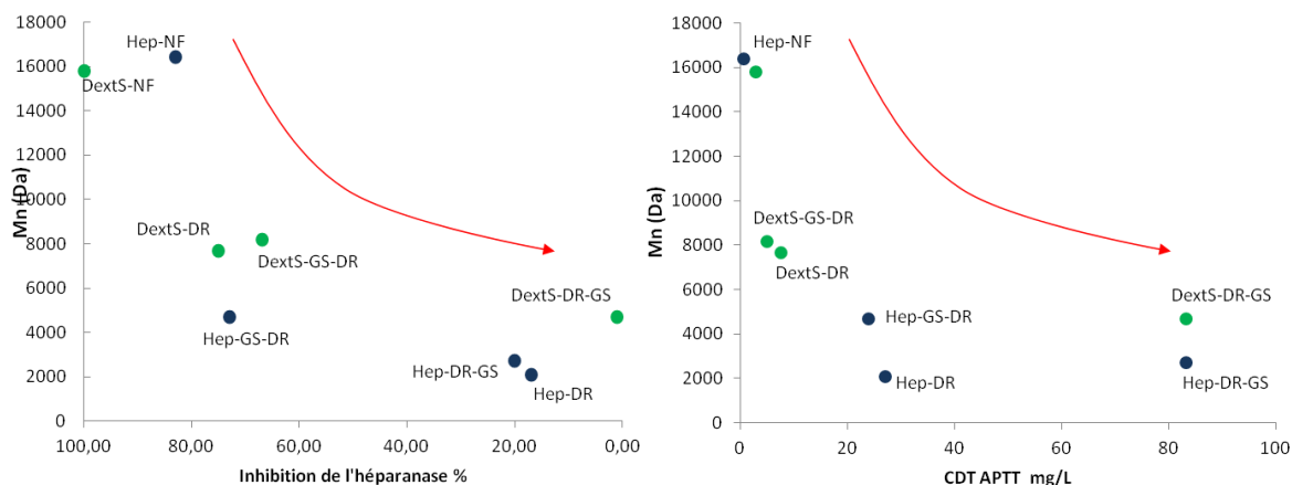
Figure 52 : Effet de la diminution du poids mol culaire moyen des polysaccharides sur leur capacit    inhiber l'h paranase ou la coagulation (via le test aPTT).
