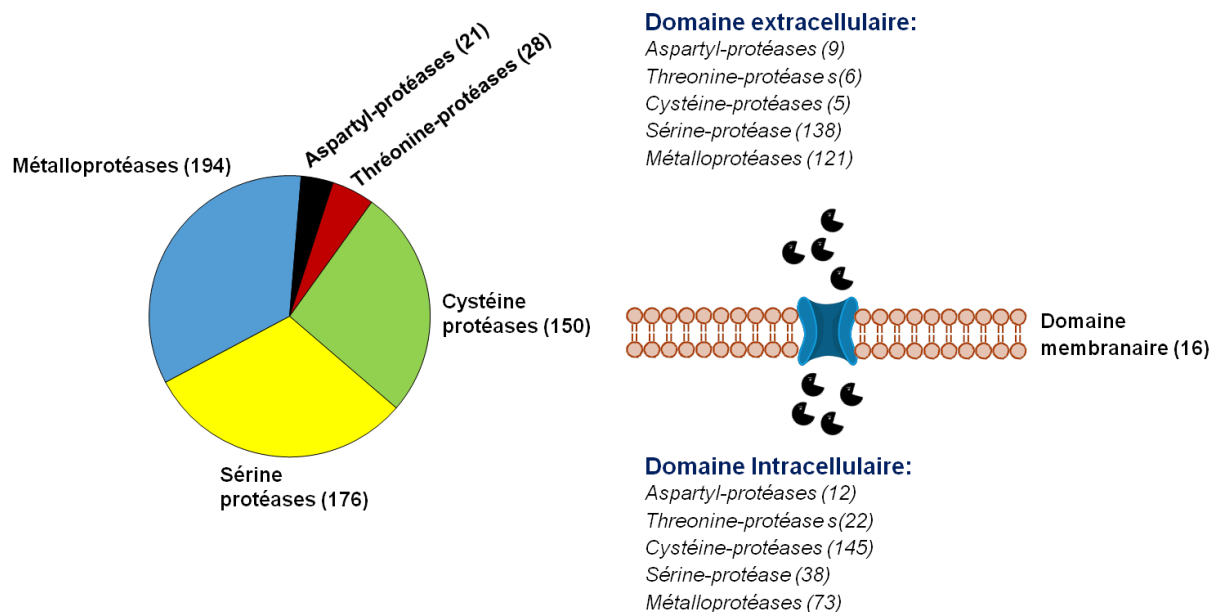
Figure 19 : Dégradome humain et localisation des protéases ( Theocharis, Adv Drug Deliv Rev, 2016)
