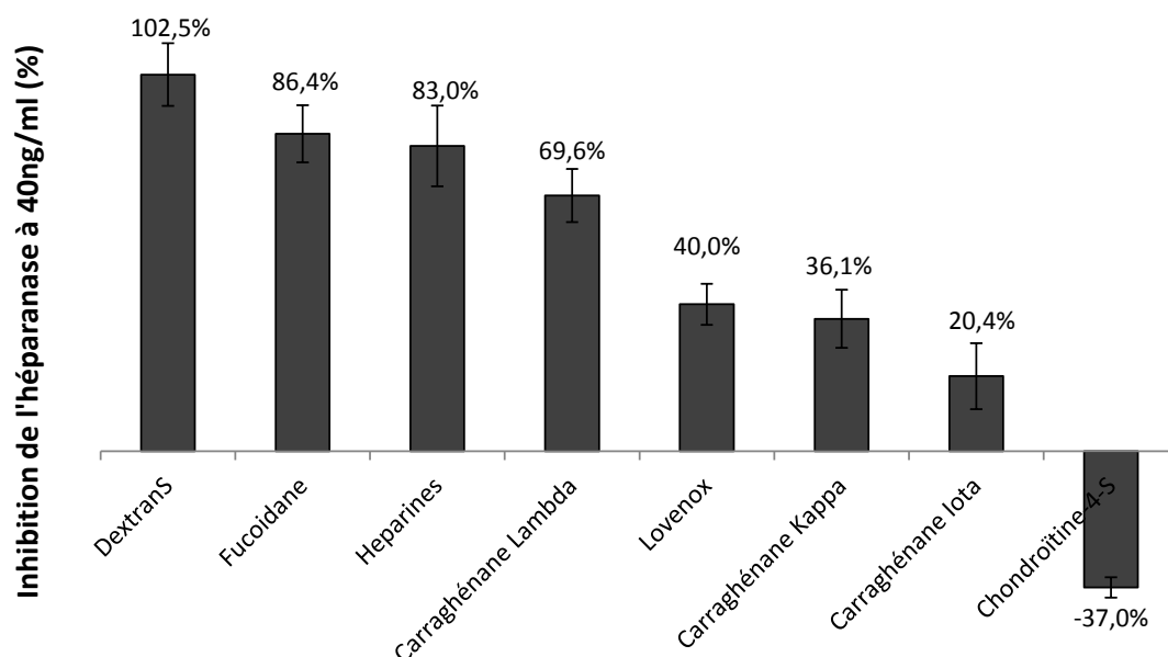
Figure 44 : Inhibition relative de l'héparanase par chaque polysaccharide non fractionné à une concentration de 40ng/ml
