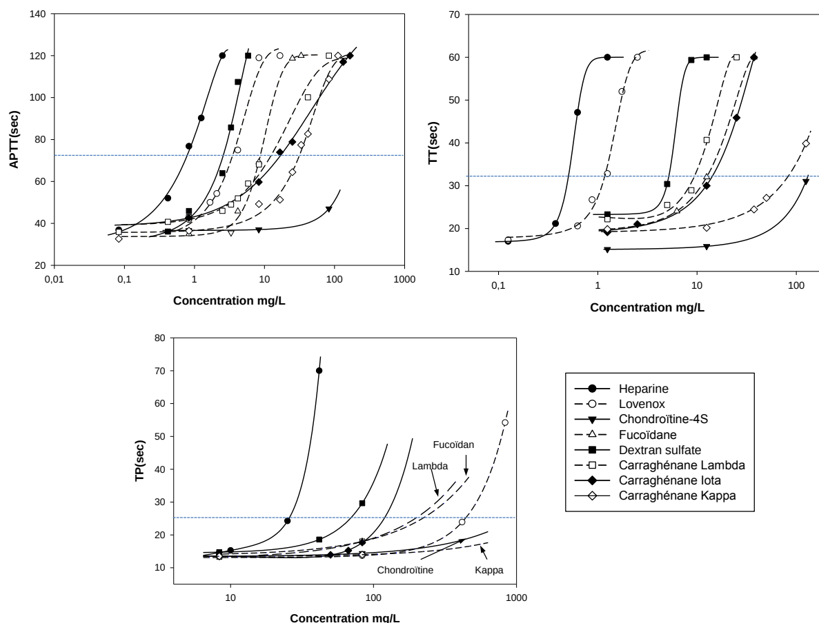
Figure 45 : Analyses chronométriques APTT, TT et TP des activités anticoagulantes des composés NF. Les temps de coagulation des plasmas en l'absence d'inhibiteurs (contrôle négatif NaCl 0,9%) sont de 37 s pour l'APTT, 16,2 s pour le TT et 13,1 s pour le TP. Les temps maximum de coagulation pour chaque test sont de 120 s pour l'APTT, 60 s pour le TT et 70 s pour le TP. Le double du temps de coagulation basal est indiqué sur chaque graphe par la ligne pointillée en bleu clair.
