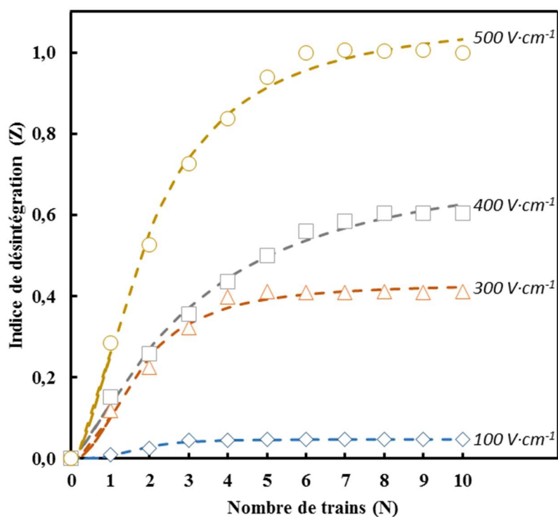
Figure III. 1 : Indice de désintégration Z en fonction de nombre de trains N pour les haricots verts (pièces de 1,1 \pm 0,1 cm) en appliquant quatre intensités de champ (100, 300, 400, et 500 V \cdot cm^{-1} ) (lignes : modèle, marques : valeurs expérimentales)
