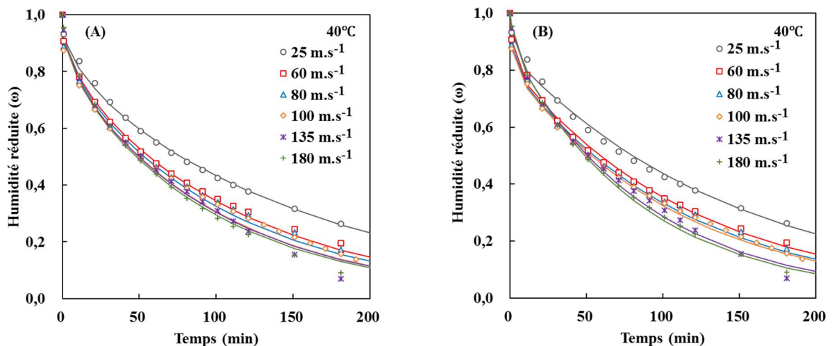
Figure V. 4 : Comparaison entre les données expérimentales et modélisées des courbes de séchage pour différentes vitesses d'air (a) modélisation avec la solution analytique n = 2 (1 paramètre identifié) (b) modélisation avec le modèle de diffusionnel (3 paramètres identifiés)
