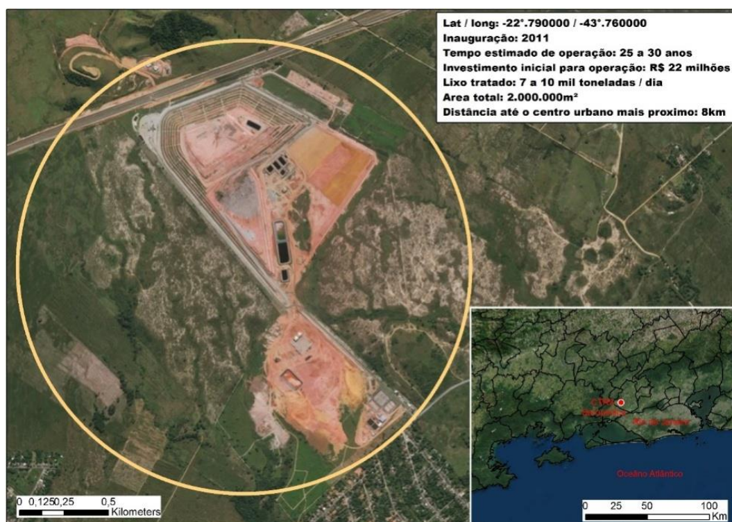
Figure 68: Carte-image satellite du CTRS Seropédica Cyclus.
