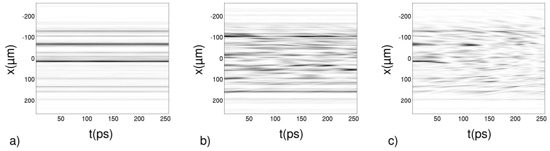
FIG. 5.10 – Evolution temporelle de la distribution de l'intensité laser le long de l'axe (x, y = 0) en sortie de plasma, pour différentes densités électroniques : a) n_0 = 0.01 n_c , b) n_0 = 0.03 n_c , c) n_0 = 0.05 n_c .
