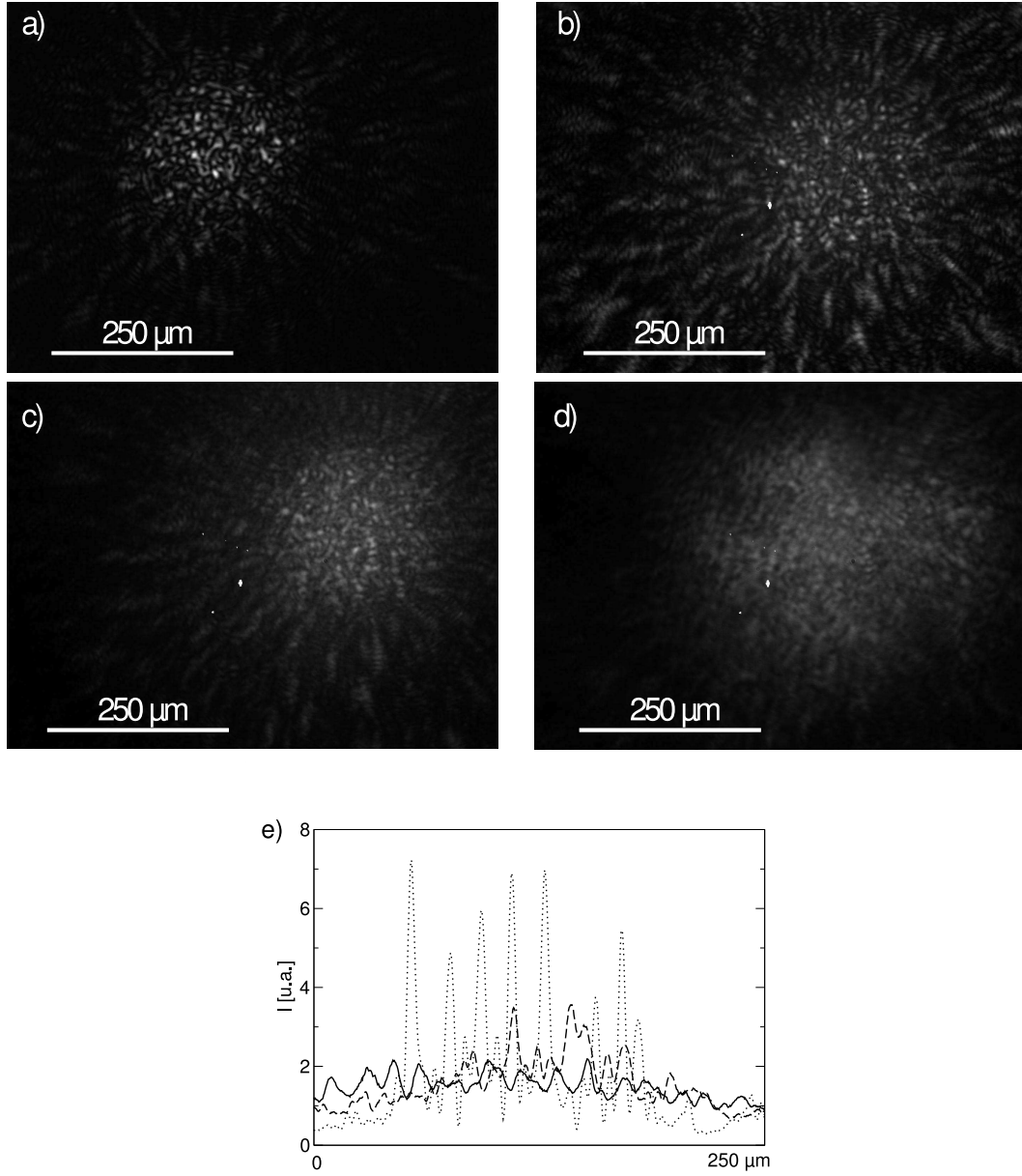
FIG. 6.7 – Imagerie 2D intégrée sur l'ensemble de l'impulsion laser du faisceau laser transmis après propagation dans : a) le vide b) pour un tir avec la composante plateau uniquement dans un gaz de densité électronique n_e \simeq 2.2 \times 10^{19} \text{ cm}^{-3} c) un gaz de densité électronique n_e \simeq 1.4 \times 10^{19} \text{ cm}^{-3} ( i.e. une pression amont sur la buse de 35 bars environ) d) un gaz de densité électronique n_e \simeq 2.2 \times 10^{19} \text{ cm}^{-3} ( i.e. une pression amont sur la buse de 90 bars environ). e) Coupe horizontale de l'intensité laser intégrée en temps pour ces différents cas (vide : courbe pointillet, n_e \simeq 1.4 \times 10^{19} \text{ cm}^{-3} courbe discontinue et n_e \simeq 2.2 \times 10^{19} \text{ cm}^{-3} courbe pleine).
