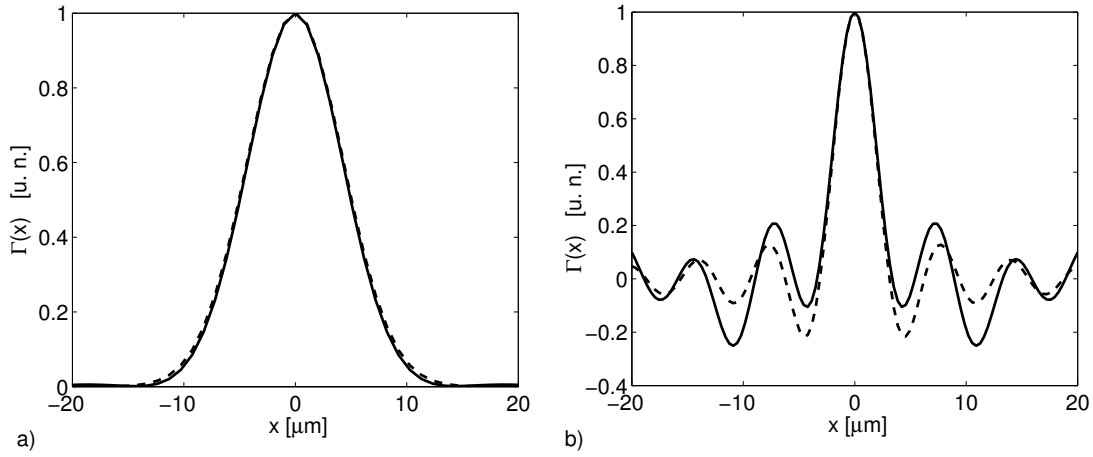
FIG. 5.2 – Fonction de corrélation spatiale du champ électrique dans le plan transverse au meilleur foyer telle qu'elle est calculée à partir des simulations PARAX (courbe continue) et sa forme théorique issue des Eqs. (1.83) et (1.84) (courbe discontinue). a) Cas du faisceau RPP en optique Gaussienne. b) Cas du faisceau SSD en optique carrée.
