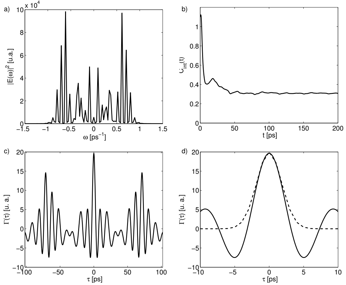
FIG. 5.3 – a) Spectre temporel du faisceau laser lissé par dispersion spectrale avec \nu_M = 14 \text{ GHz} et \beta_M = 3 . b) Evolution au cours du temps du contraste de la lumière intégrée. c) Fonction de corrélation temporelle pour le champ électrique. d) Détail de la même mesure pour des temps courts (courbe solide) et comparaison à l'Eq. (1.116) théorique (courbe discontinue).
