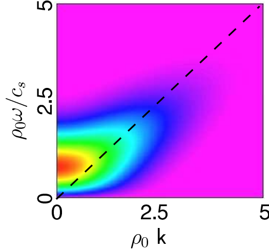
FIG. 3.10 – Evolution de la fonction \zeta_{\rho_0 \mathbf{k}}(\rho_0 \omega/c_s) avec la fréquence \omega et le nombre d'onde transverse |\mathbf{k}| . La ligne discontinue représente c_s |\mathbf{k}| = \omega .
