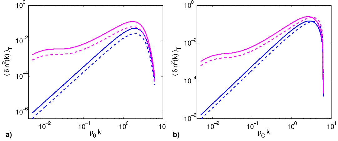
FIG. 3.6 – Spectre spatial, temporellement moyenné , des fluctuations de densité induites par un laser spatialement et temporellement lissé avec (courbes magenta) et sans (courbes bleues) prise en compte des effets thermiques. a) Pour une optique Gaussienne, le spectre est normalisé à \rho_0^2 (c_s T / \rho_0) \langle I \rangle^2 / (c n_c T_e)^2 . Pour un temps de cohérence \tau_C = \rho_0 / c_s (courbe solide), pour \tau_C = 0.1 \rho_0 / c_s (courbe discontinue). b) Pour une optique carrée, le spectre est normalisé à \rho_C^2 (c_s T / \rho_C) \langle I \rangle^2 / (c n_c T_e)^2 . Pour un temps de cohérence \tau_C = \rho_C / c_s (courbe solide), pour \tau_C = 0.1 \rho_C / c_s (courbe discontinue).
