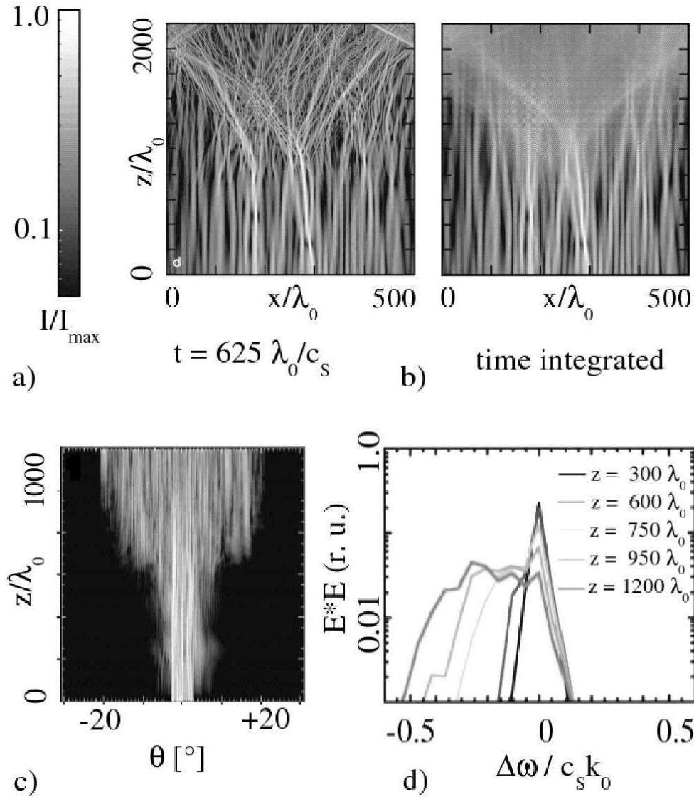
FIG. 2.1 – Distribution instantanée d'intensité dans le plasma au temps t = 625 \lambda_0/c_s (a) et intégrée en temps sur toute la simulation (b). Evolution au cours de la propagation de la distribution angulaire (c) et du spectre de la lumière laser (d). Résultats de simulations numériques tirés de la Réf. [Schmitt 98].
