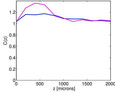
FIG. 5.20 – Evolution au cours de la propagation dans un plasma de densité n_0 = 0.05 n_c et pour un temps t \simeq 260 ps du contraste instantané avec (courbe magenta) et sans (courbe bleue) prise en compte des effets thermiques.
