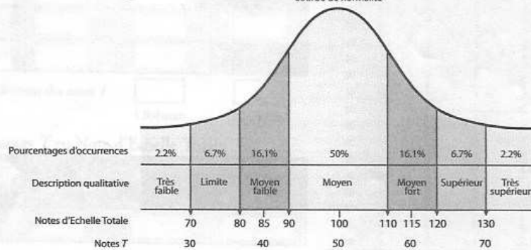
Courbe de normalité
