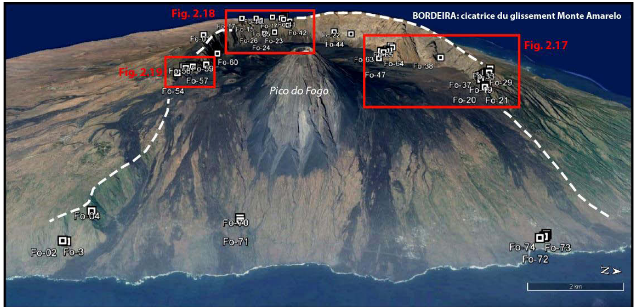
Figure 2.16 : Carte de l'échantillonnage dans la caldera de Fogo (Cap Vert), cicatrice d'une déstabilisation massive de l'édifice volcanique Monte Amarelo. Les échantillons pré-collaps sont situés sur les parois de la caldera (Bordeira), tandis que les échantillons post-effondrement fossilisent la paroi ou remplissent la cicatrice de glissement.
