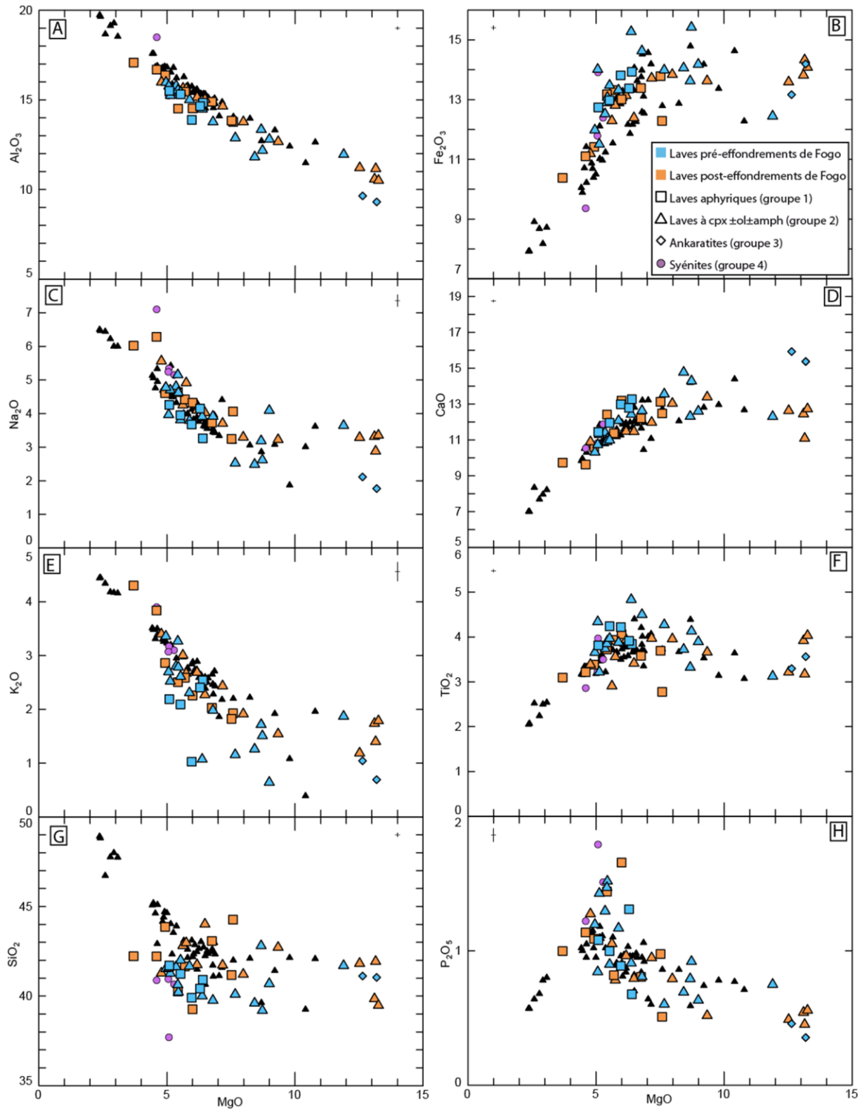
Figure 4.5 : Variation des teneurs des oxydes en fonction du MgO (pds.%). Les données de la littérature (Doucelance et al. , 2003; Escrig et al. , 2005 ; Hildner et al. , 2012, Mata et al. , 2017) sont représentées par les triangles noirs. Les barres d'erreur sont reportées en haut des graphiques.
