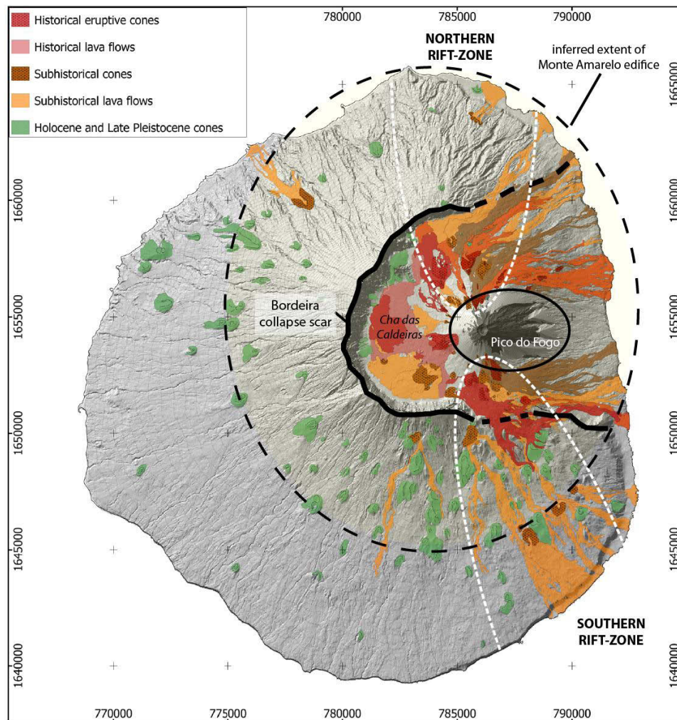
Figure 2.11 : Carte morpho-structurale schématisée de l'île de Fogo (Cap Vert). L'extension de l'édifice Amarelo n'est pas très bien documentée, mais elle correspond à une rupture de pente assez marquée dans la partie sommitale. Les rift-zones sont moins bien définies que celles des îles Canaries. En revanche, la cicatrice du glissement du Monte Amarelo (caldera ouverte vers l'Est délimitée par la Bordeira) est bien visible, avec le Pico et les coulées historiques en remplissage post-effondrement.
