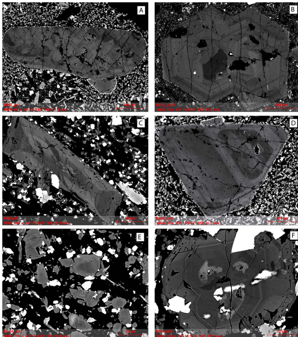
Figure 6.2 : Images en électrons rétrodiffusés (BSEI) de pyroxènes. A, B, C et D : mégacristaux de pyroxènes montrant des zonations chimiques complexes. E : mésostase de l'échantillon BC-04. F : microlite de pyroxène de la laves RF-03.
