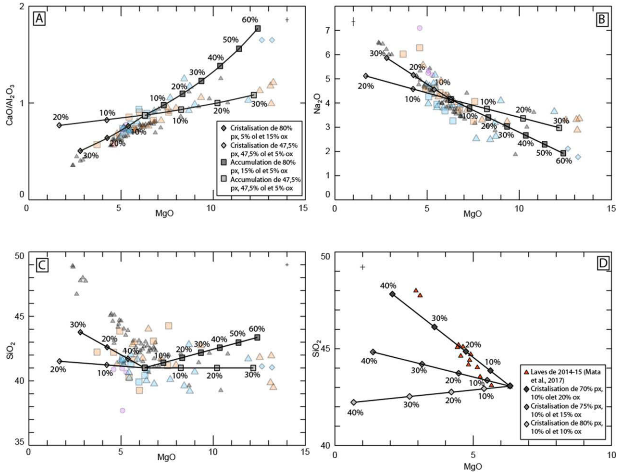
Figure 5.1 : Variation du rapport \text{CaO}/\text{Al}_2\text{O}_3 (A), des teneurs en \text{Na}_2\text{O} (B) et en \text{SiO}_2 (C, D) en fonction de \text{MgO} . Les losanges représentent l'évolution des différentes grandeurs par cristallisation fractionnée, alors que les carrés reflètent l'accumulation de cristaux dans les laves de Fogo. La sous-figure D considère la cristallisation de pyroxènes et d'oxydes (de fer et titane) à partir d'un magma dont la composition est identique à la lave la plus riche en \text{MgO} de l'éruption de 2014 (Mata et al. , 2017). Les teneurs des laves de Fogo sont reproduites par un maximum de 30% de cristallisation fractionnée d'un cumulat constitué de 80% de cpx, 5% d'ol et 10% d'ox, et par l'accumulation en proportions variables de cpx, ol et ox.
