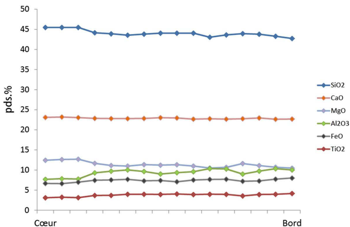
Figure 4.3 : Profil d'un macrocristal de clinopyroxène de la lave FO-24. Ce profil du cœur du cristal jusqu'à sa bordure mesure 500 µm. Les variations de zonation chimique sont faibles ; ~3 pds.% pour SiO 2 et 2 pds.% pour MgO.
