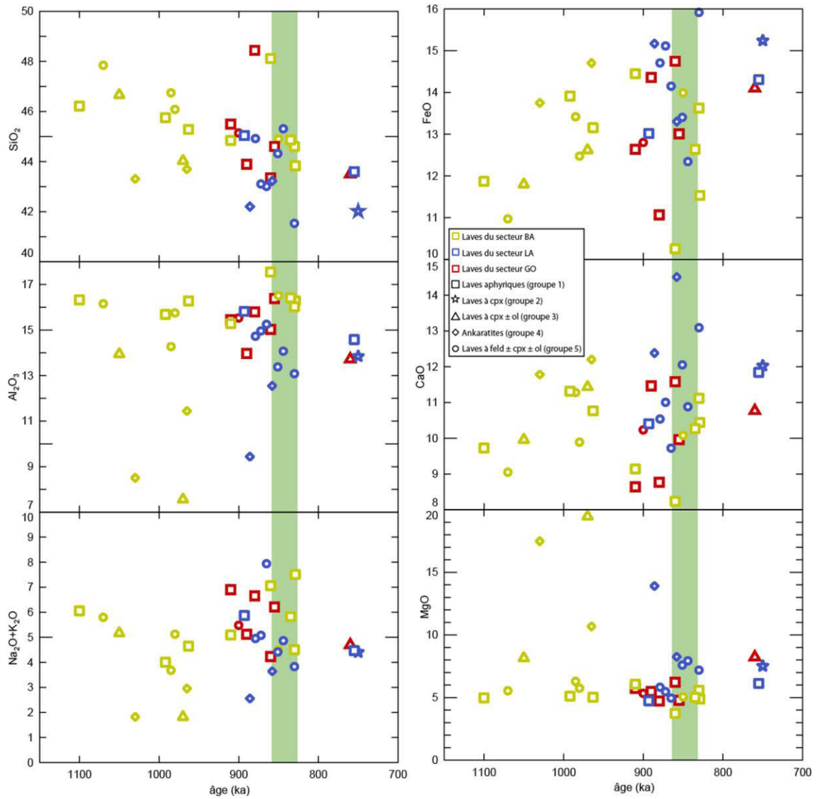
Figure 6.7 : Diagramme des concentrations des différents oxydes (pds.%) en fonction du temps (en ka) de trois secteurs de Güímar (BA, LA et GO).
