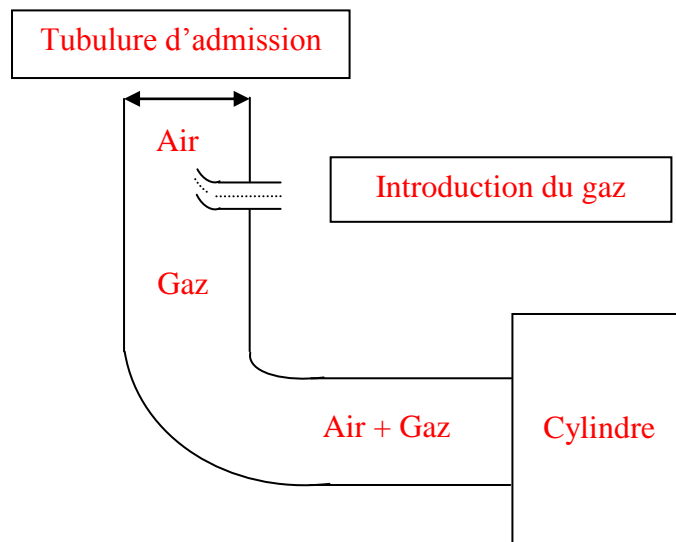
Figure II.6 : Schéma de l'introduction du combustible gazeux.
