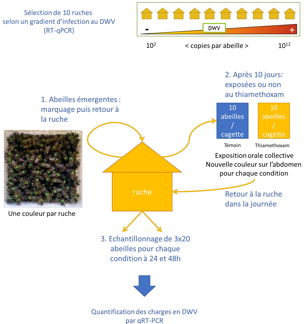
Figure 28 : Schéma récapitulant la méthode utilisée afin de tester l'effet d'une exposition aiguë au thiaméthoxam sur des abeilles provenant de colonies infectées selon un gradient de la plus faible charge en DWV à la plus élevée.
