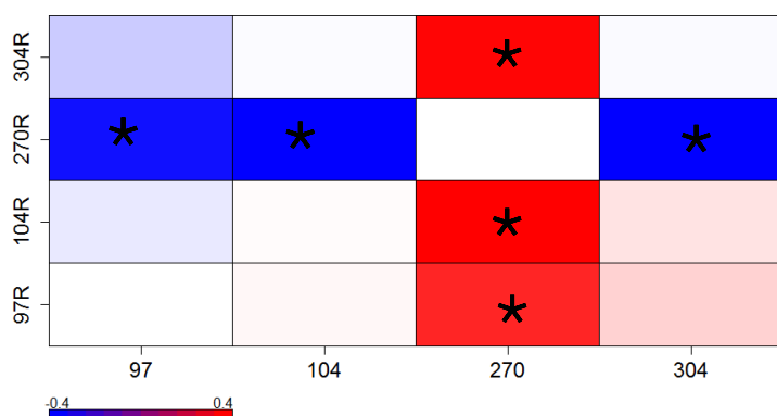
Figure 5-2: Fitness des souches transformées (représentées sur l'axe des ordonnées) dans les différentes compétitions. Les étoiles indiquent les fitness significativement différentes de zéro au seuil de 5%.
