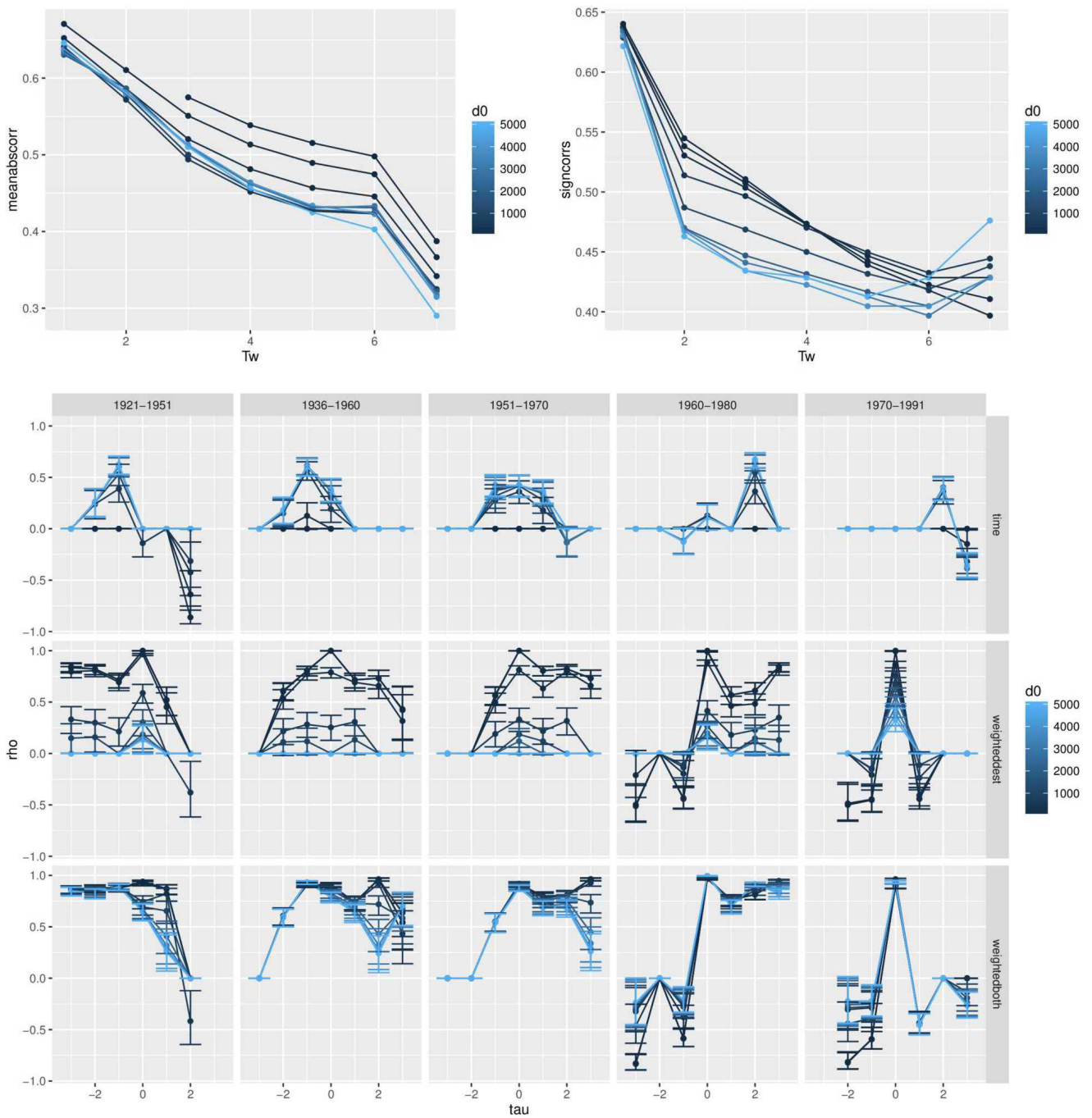
FIGURE 82: (Haut Gauche) Corrélations absolues moyennes sur l'ensemble des retards, en fonction de la taille de la fenêtre temporelle T_W (en nombre d'observations temporelles), pour différentes valeurs du paramètre de décroissance d_0 ; (Haut Droite) Proportion de corrélations significatives, en fonction de T_W pour d_0 variable; (Bas) Corrélations retardées en fonction du délai \tau , pour la taille optimale T_W = 3 , sur les différentes périodes successives (colonnes), pour les différents degrés de pondérations (première ligne w_i = 1, w_j = P_j / \sum_k P_k , deuxième ligne w_i = P_i / \sum_k P_k, w_j = P_j / \sum_k P_k ), et pour d_0 variable (couleur).
