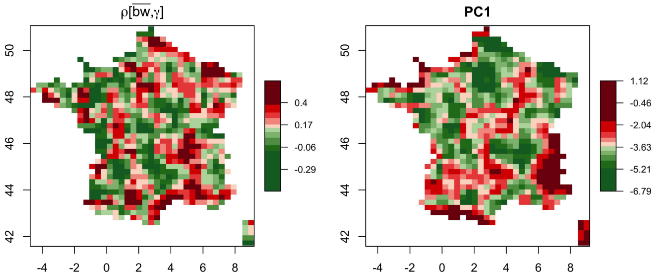
FIGURE 23 : Exemples de corrélations spatiales. Pour la France, les cartes donnent \rho[\bar{b}w, \gamma] , corrélation entre la centralité de chemin moyenne et la hiérarchie de la population ( Gauche ) et la première composante de la matrice réduite ( Droite ).
