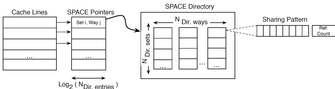
FIGURE 3.7 – Répertoire SPACE
